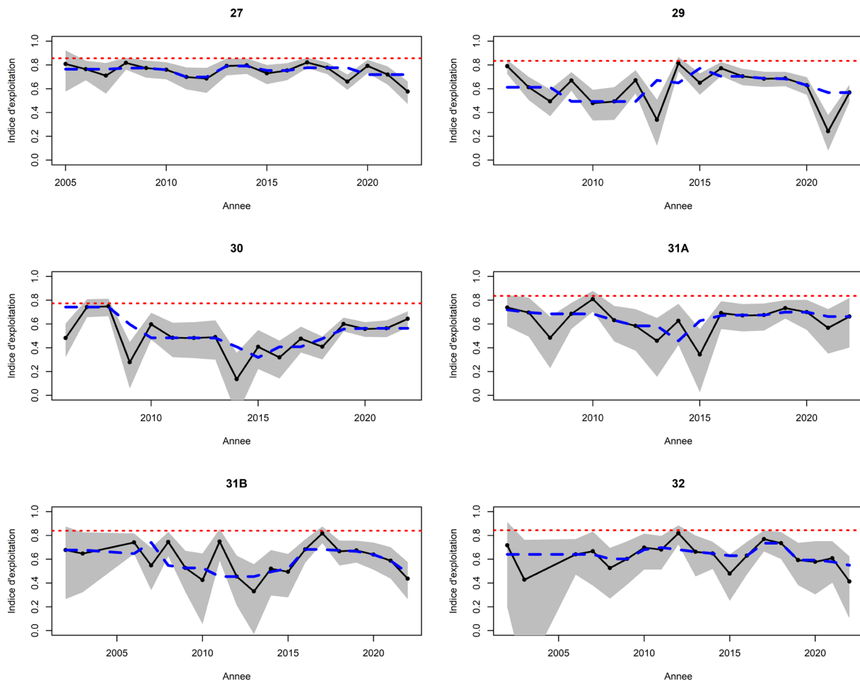
Figure 4. Séries chronologiques des indices d'exploitation calculés selon la méthode du changement de proportions en continu (noir), avec médiane mobile sur trois ans (ligne tiretée bleu) et taux d'exploitation de référence (ligne pointillée rouge). Les intervalles de crédibilité de 95 % sont grisés. Aucune estimation de l'exploitation n'existe pour la ZPH 28.
