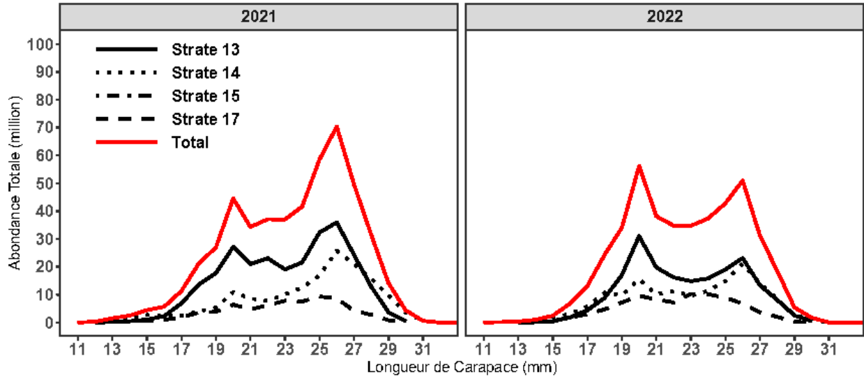
Figure 6. Prises selon la longueur d'après l'échantillonnage des prises commerciales par strate pour 2021 et 2022.
