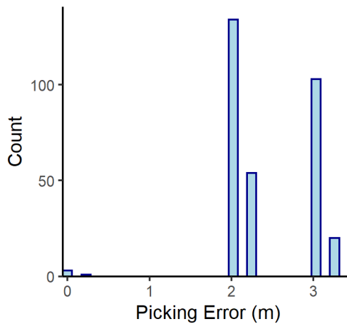
Springvale n= 315
