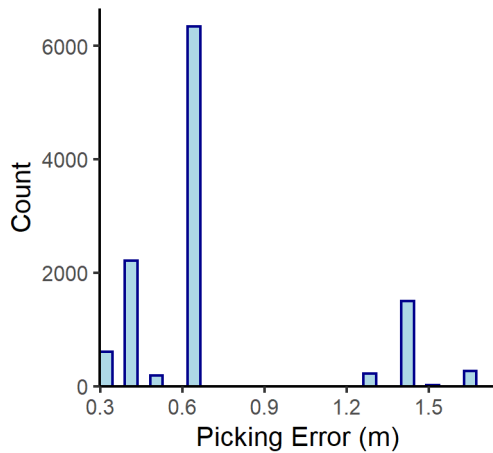
Dundee n= 11369
