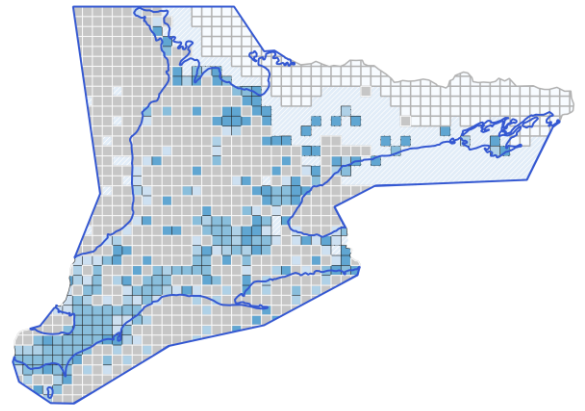
Cobourg
