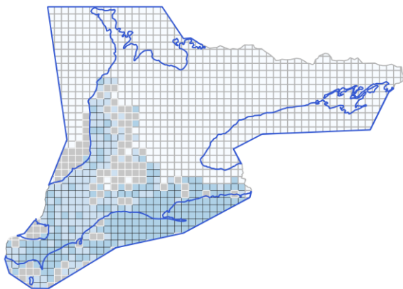
B Anhydrite
