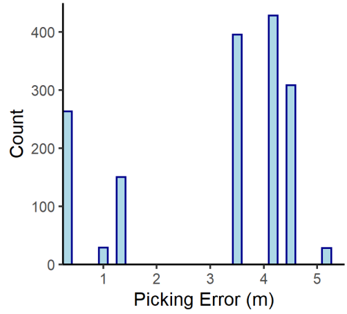
Cobourg n= 1601
