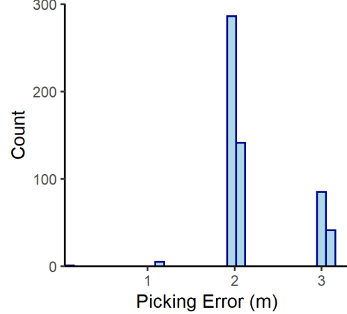
Eramosa n= 559
