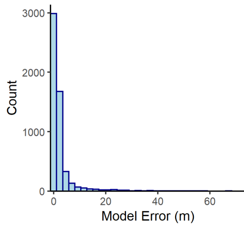
A-2 Anhydrite n= 5473
