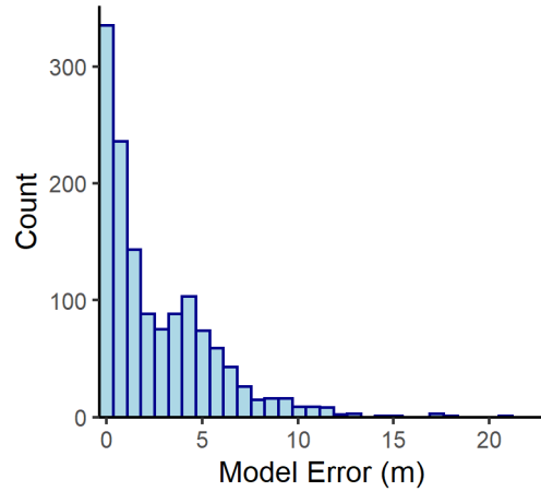
Eramosa n= 1355
