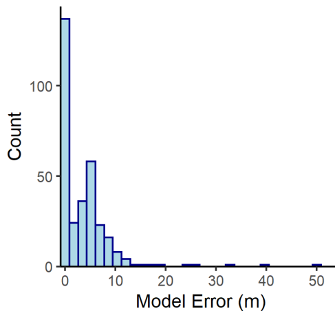
Springvale n= 315
