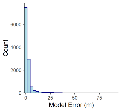
A-2 Carbonate n= 11497
