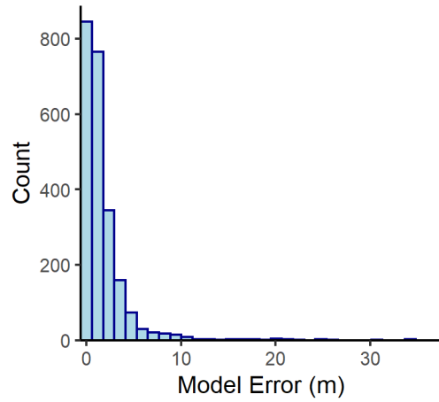
A-1 Evaporite n= 2305
