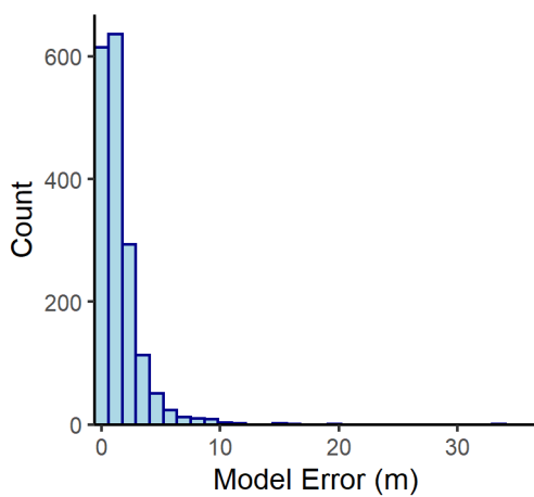
A-2 Salt n= 1772
