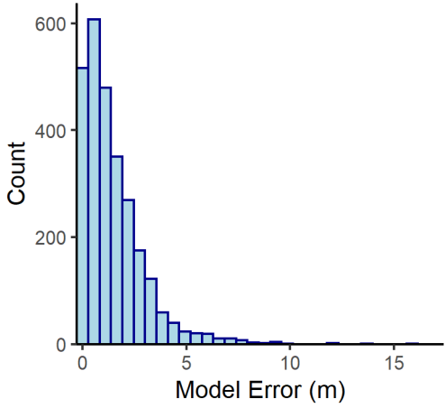
Thorold n= 2720
