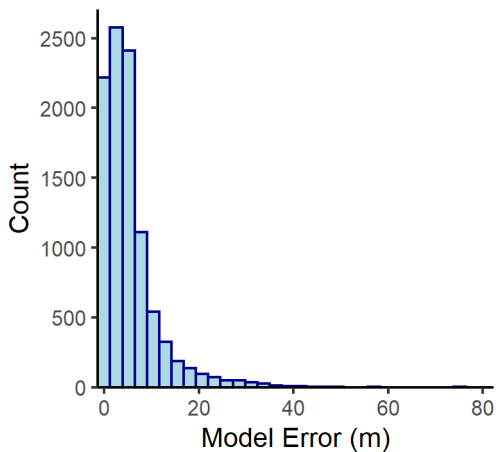
Bois Blanc n= 9866
