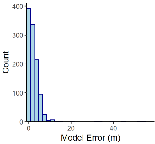
Shadow Lake n= 1082
