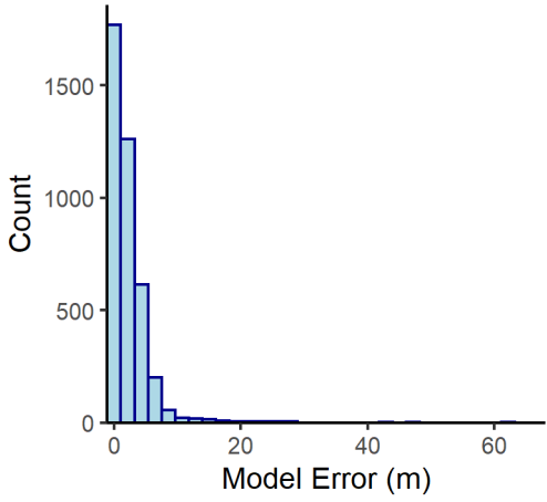
B Anhydrite n= 3992
