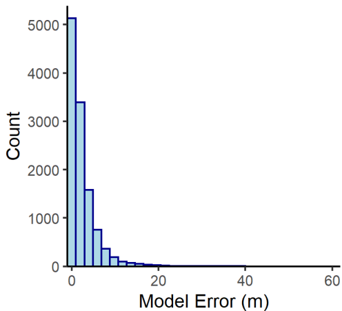
Onondaga - Amherstburg n= 11743
