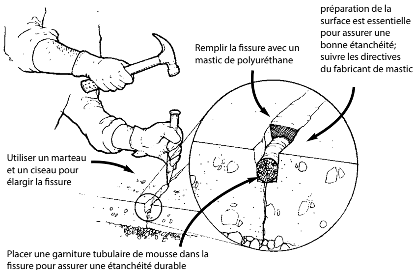
Figure 5 ↑ Obturation des fissures dans les murs de fondation et les planchers.
