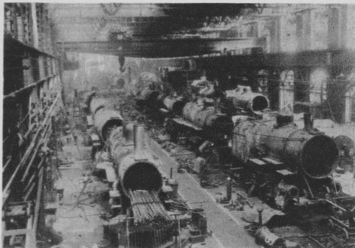
Un taller de los ferrocarriles canadienses donde se construyen algunas de las más grandes locomotoras.
