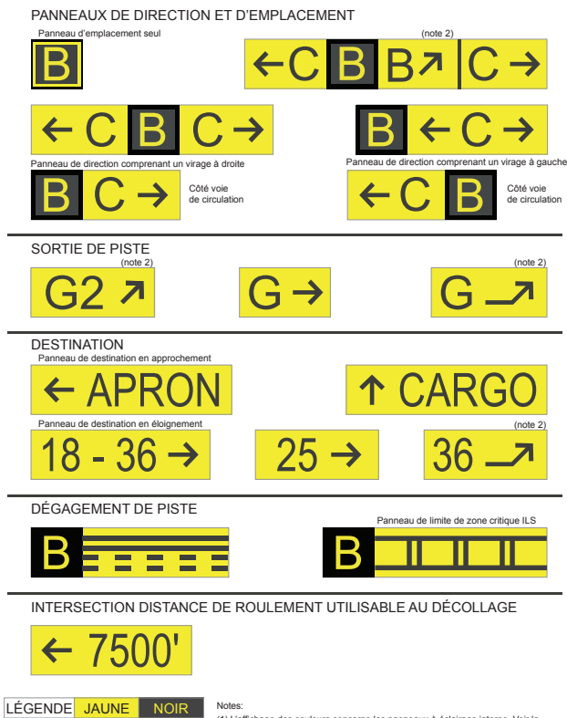
Figure 5.13 – Panneaux d'indication
