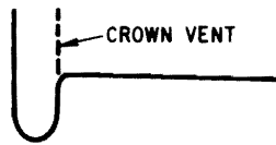
(d) Crown vented trap
