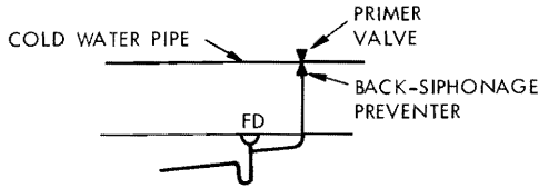
(d) Trap seal primer
