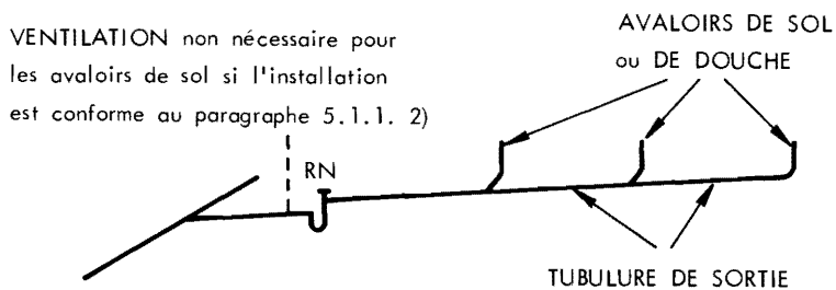
b) Avaloirs de sol et de douche
