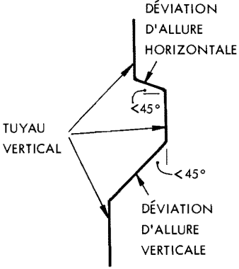
a) Tuyau vertical - élévation
