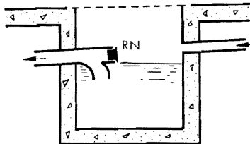
b) Puisard siphonné
