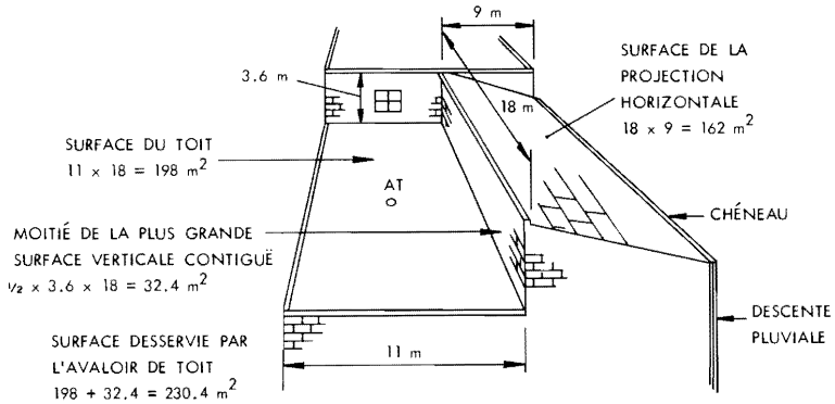
Surface de toit à desservir (exemple I)
