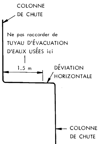
a) Raccordement à une déviation d'allure horizontale
