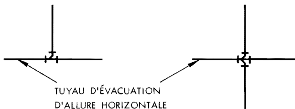
c) Interdit (utiliser une culotte simple suivie d'un coude au 1/8)
