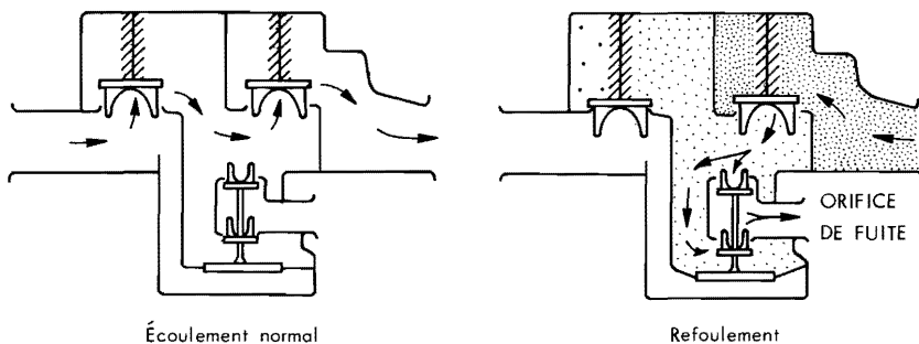
a) Dispositif anti-refoulement à réduction de pression
