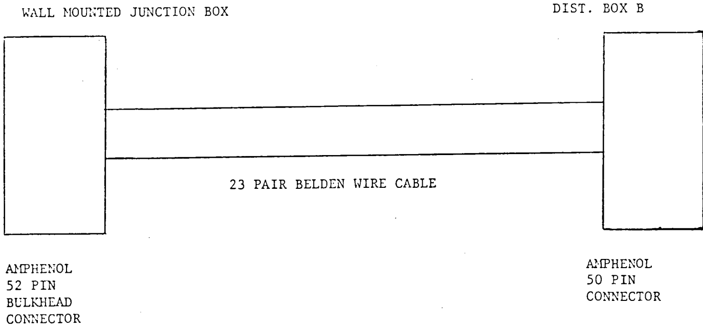
Fig. 9-II: Cable D
