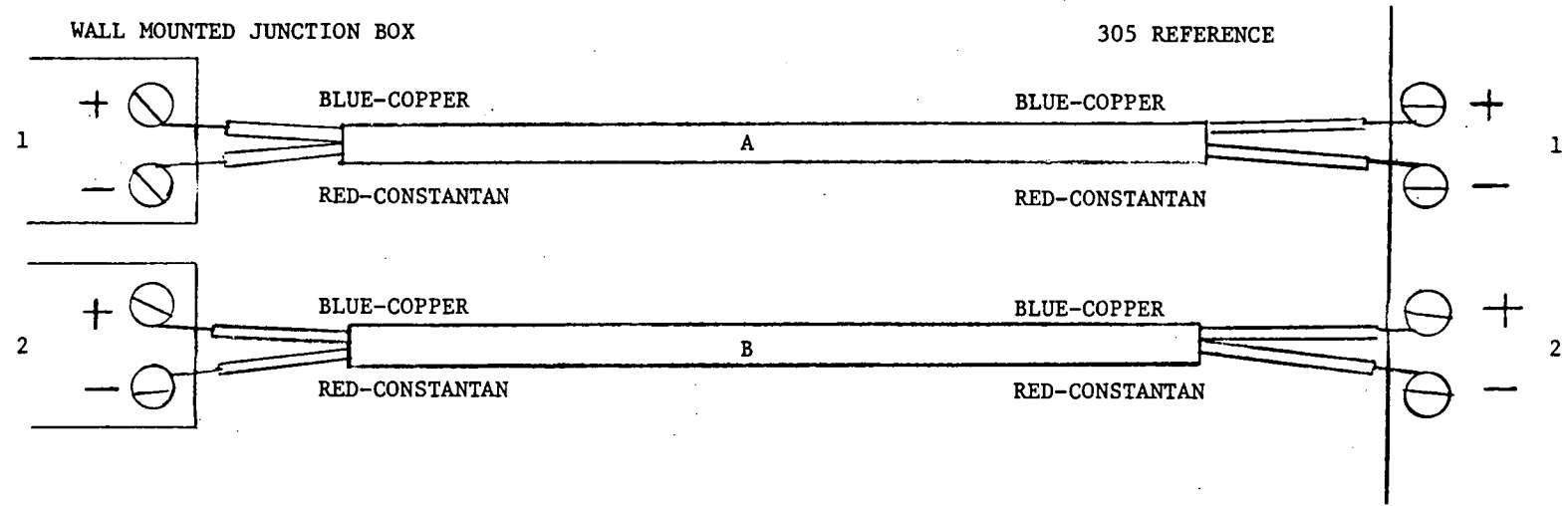
Fig. 8-II: Cable C
