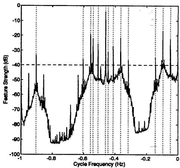
(d) A(N=32768, Np=8)
