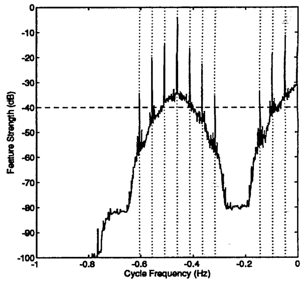
(d) A ( N=32768, Np=64 )
