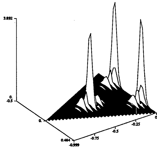
(b) A (N=32768, Np=32)
