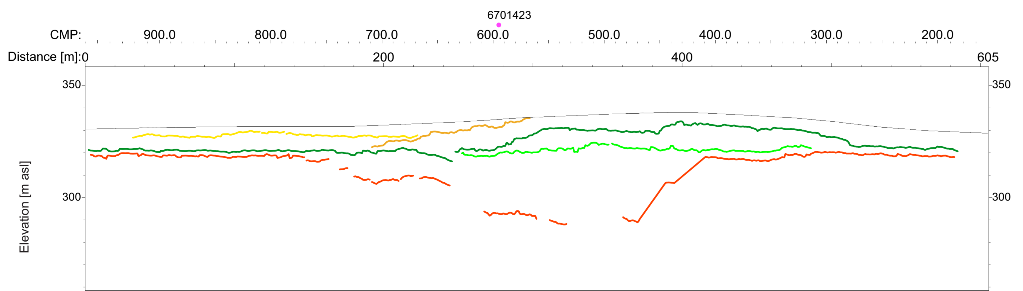
S-interpretation (depth):
