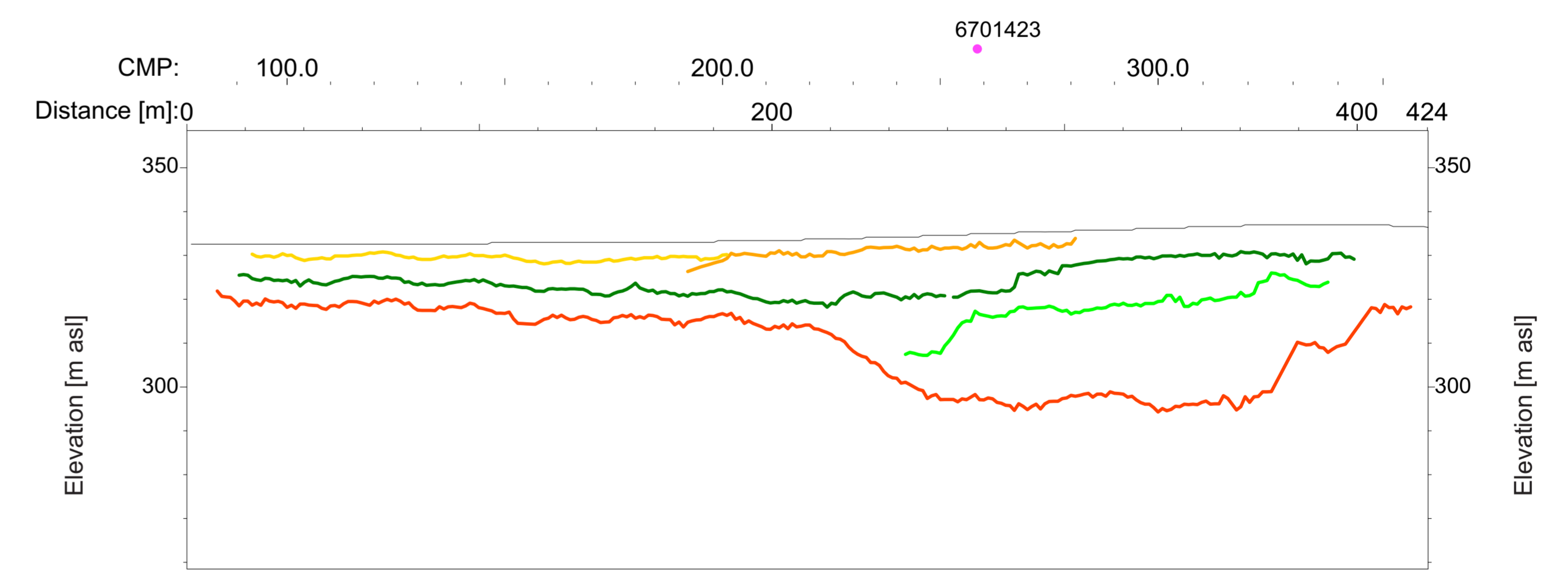
P-interpretation (depth):
