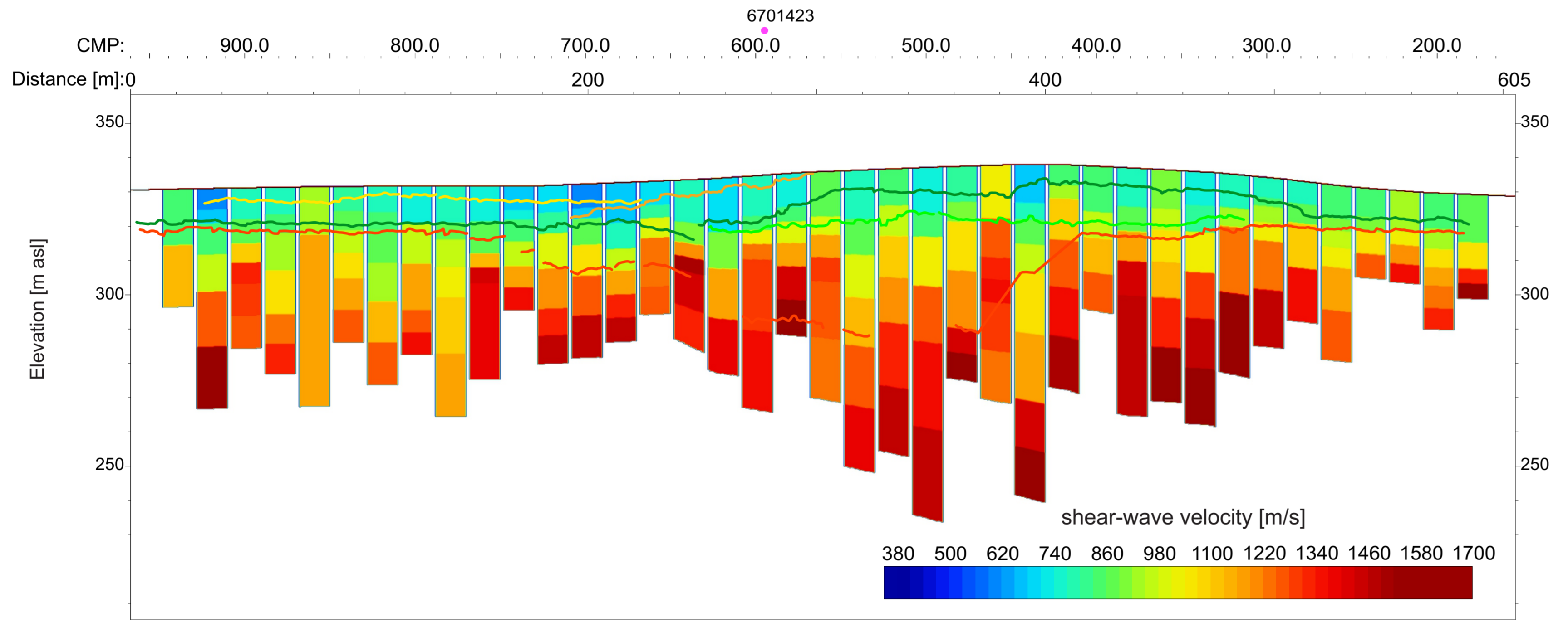
S-interpretation (depth):
