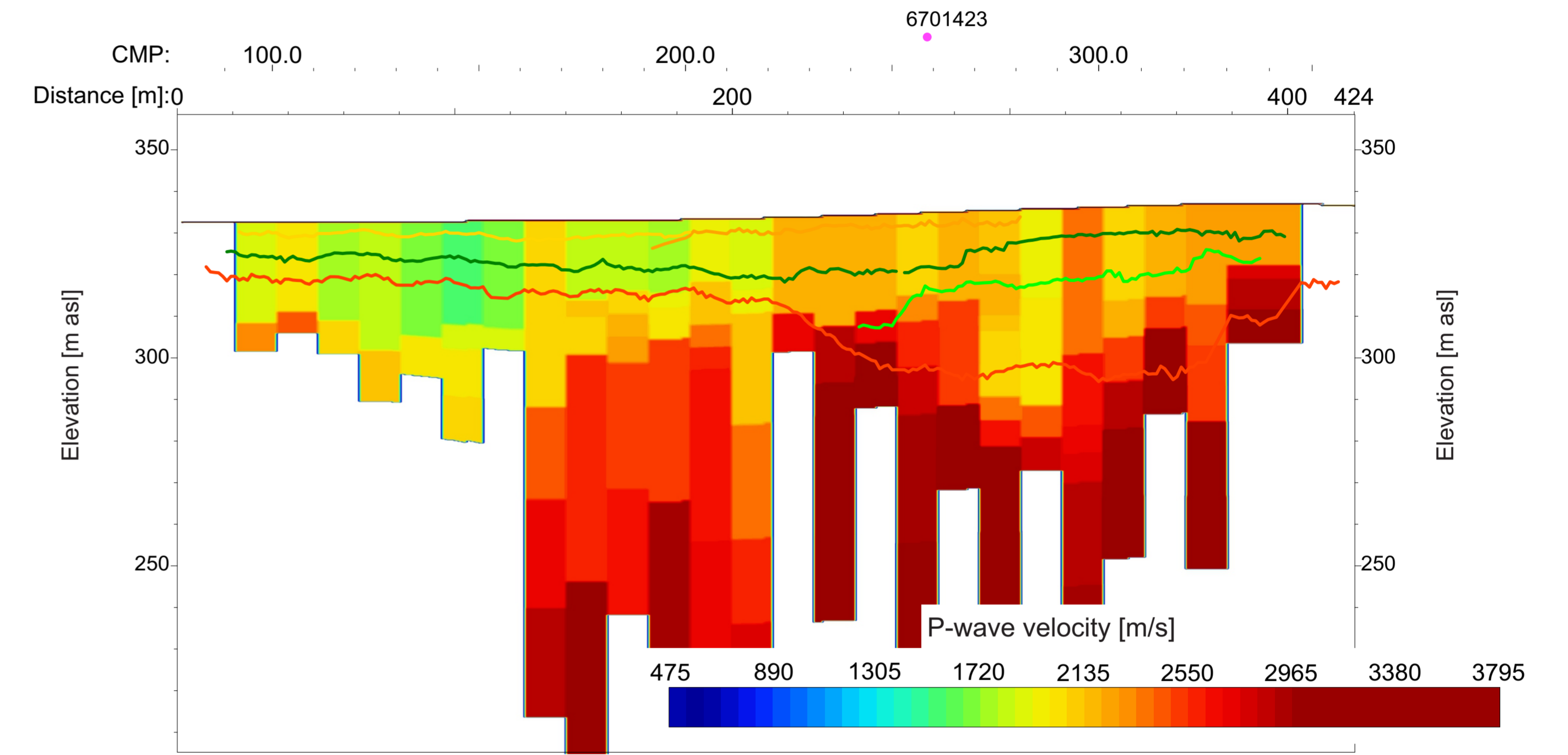
P-interpretation (depth):
