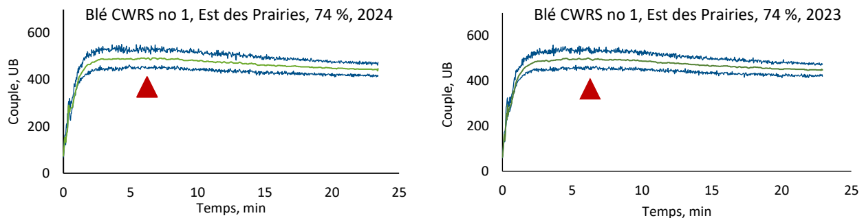
Figure 2. Exemples de farinogrammes (bol de 300 g) générés à partir de farine obtenue à un taux d'extraction de 74 % avec les échantillons de l'Est des Prairies regroupés de blé CWRS no 1 des campagnes agricoles 2023 et 2024. Les valeurs de couple minimal et maximal (bleu), les valeurs de couple moyen (vert) et le temps de développement de la pâte (flèche rouge) sont indiqués.
