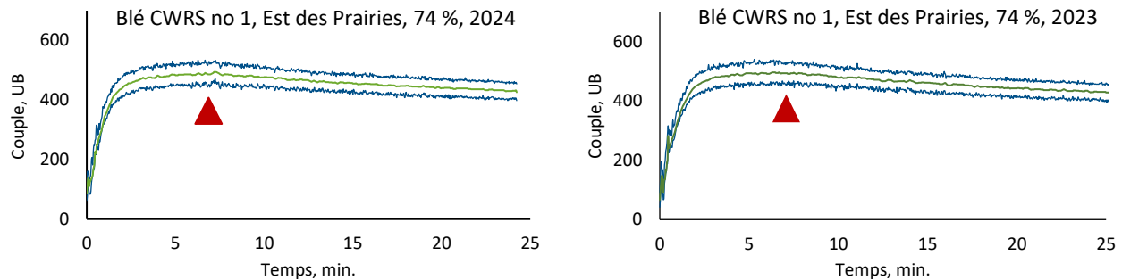
Figure 1. Exemples de farinogrammes (bol de 50 g) générés à partir de farine obtenue à un taux d'extraction de 74 % avec les échantillons de l'Est des Prairies regroupés de blé CWRS no 1 des campagnes agricoles 2023 et 2024. Les valeurs de couple minimal et maximal (bleu), les valeurs de couple moyen (vert) et le temps de développement de la pâte (flèche rouge) sont indiqués.
