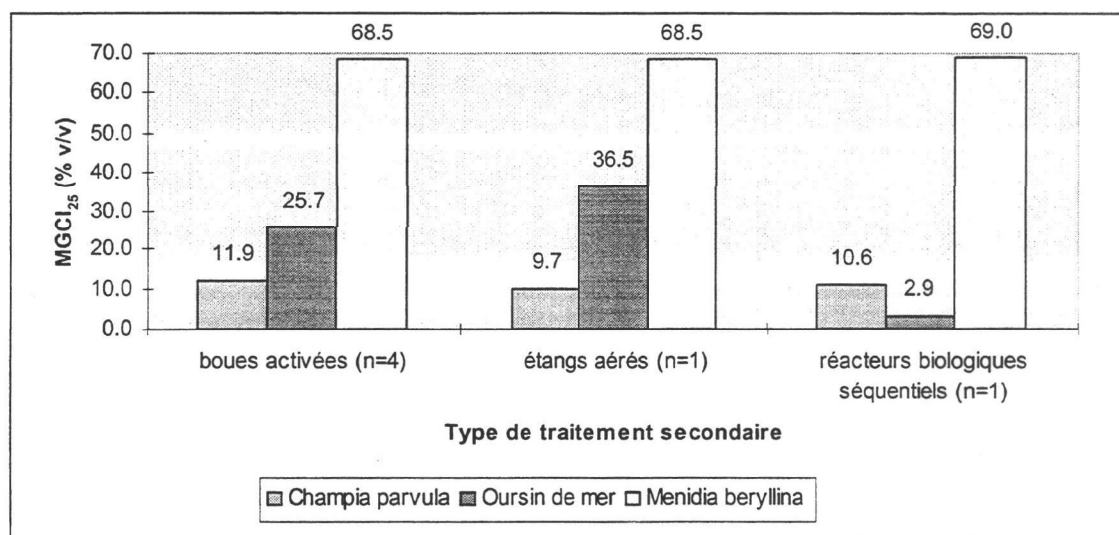
Figure 5 Toxicité sous-létale moyenne selon le type de traitement secondaire appliqué aux effluents en milieu marin.
