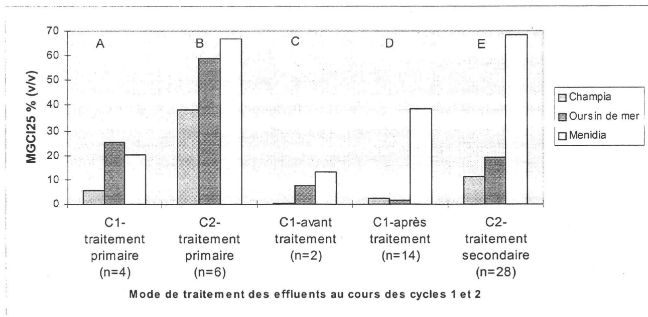
Figure 9 Toxicité sous-létale moyenne pour chaque organisme d'essai en fonction du mode de traitement des effluents aux usines dont l'effluent se déverse en milieu marin.
