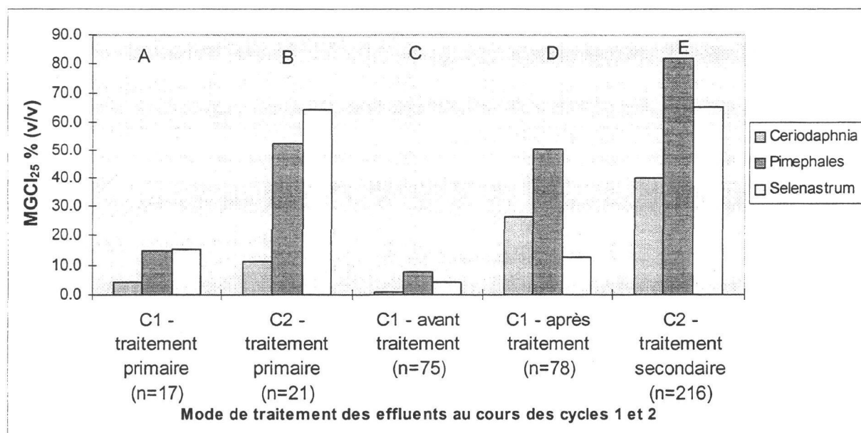
Figure 8 Toxicité sous-létale moyenne pour chaque organisme d'essai en fonction du mode de traitement des effluents aux usines dont l'effluent se déverse en eau douce.
