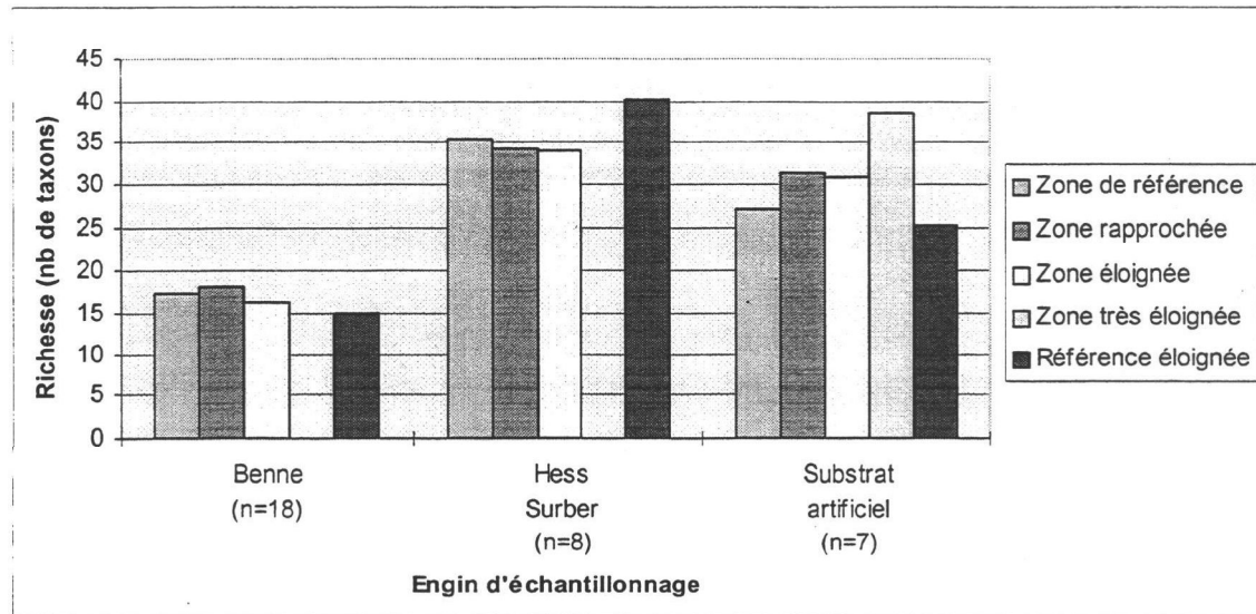
Figure 14 Nombre moyen de taxons d'invertébrés benthiques selon le type d'engin utilisé et la zone d'étude au cycle 2
