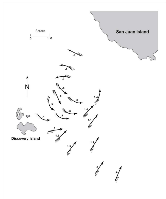
FIGURE 3.1 : TOURBILLON CRÉÉ PAR LE COURANT DE FLOT DANS LA PARTIE SUD DU HARO STRAIT
