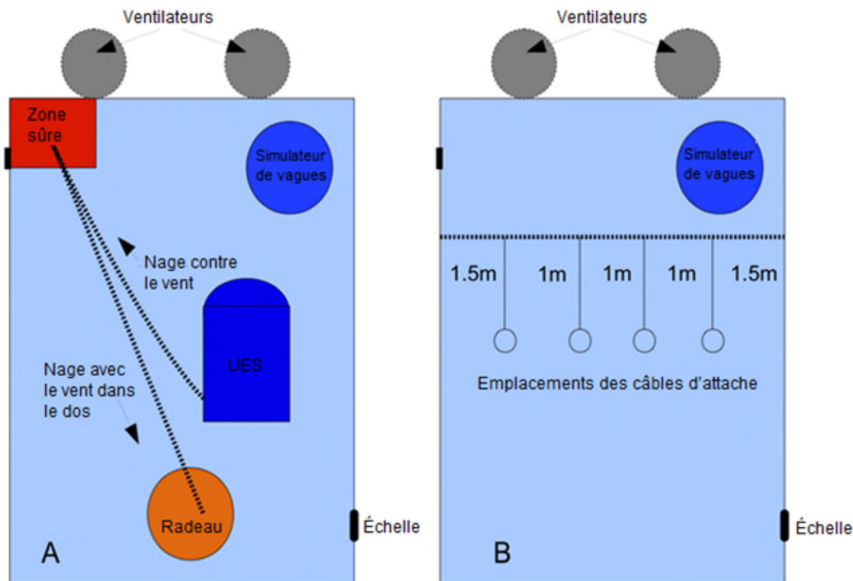
Figure R.1 — Disposition de l'équipement pour les essais d'infiltration d'eau (UES et immersion pendant la phase de survie)
