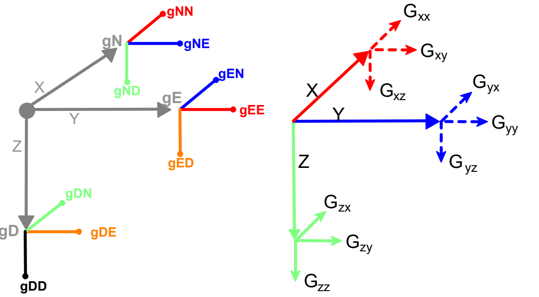
FALCON ® airborne gravity gradiometer and the gravity gradient tensor components convention / Système gradio-gravimétrique aéroporté FALCON ® et convention des composantes du tenseur de gradient de gravité
