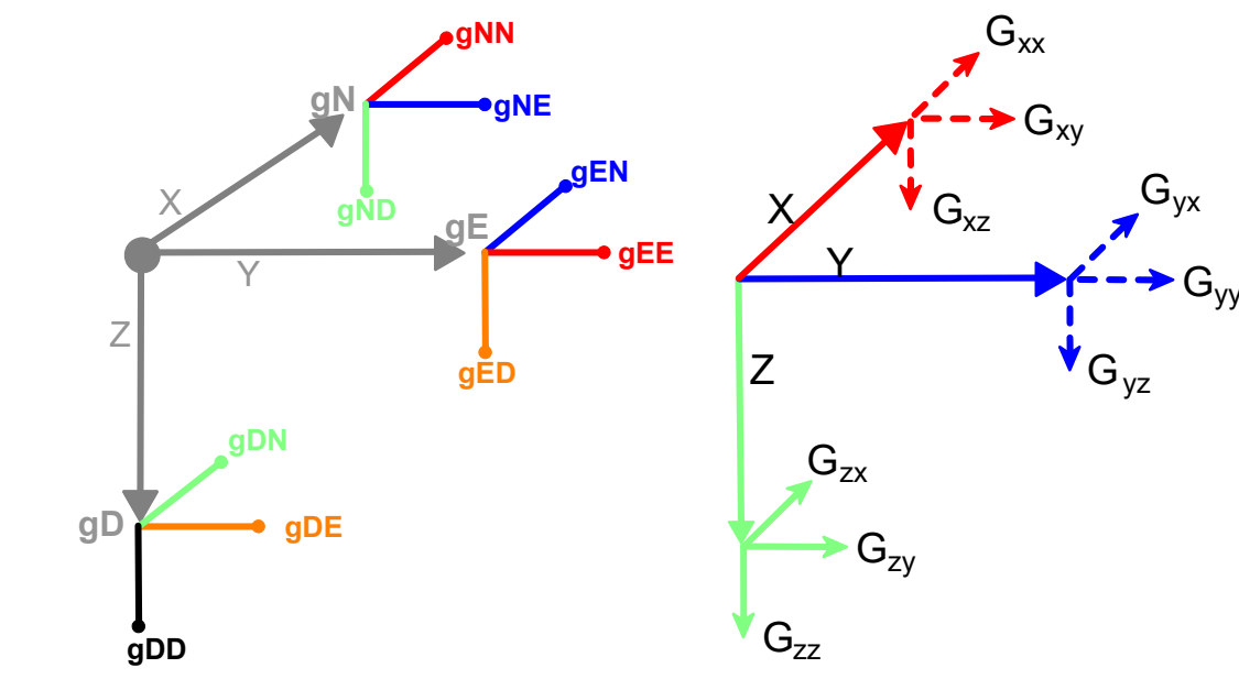
FALCON® airborne gravity gradiometer and the gravity gradient tensor components convention / Système gradio-gravimétrique aéroporté FALCON® et convention des composantes du tenseur de gradient de gravité
