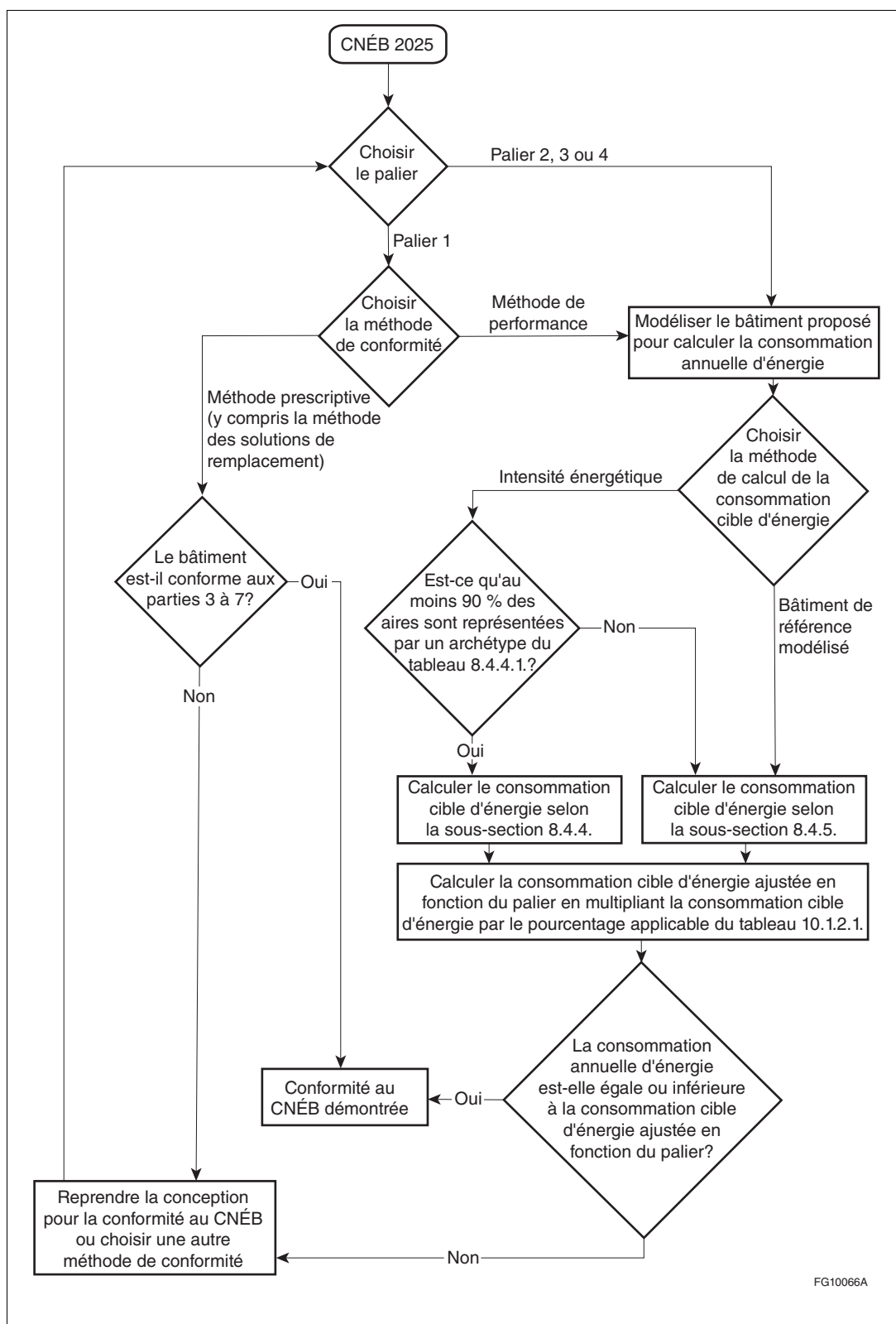
Figure A-1.1.2.1. Organigramme des méthodes de conformité aux exigences énergétiques
