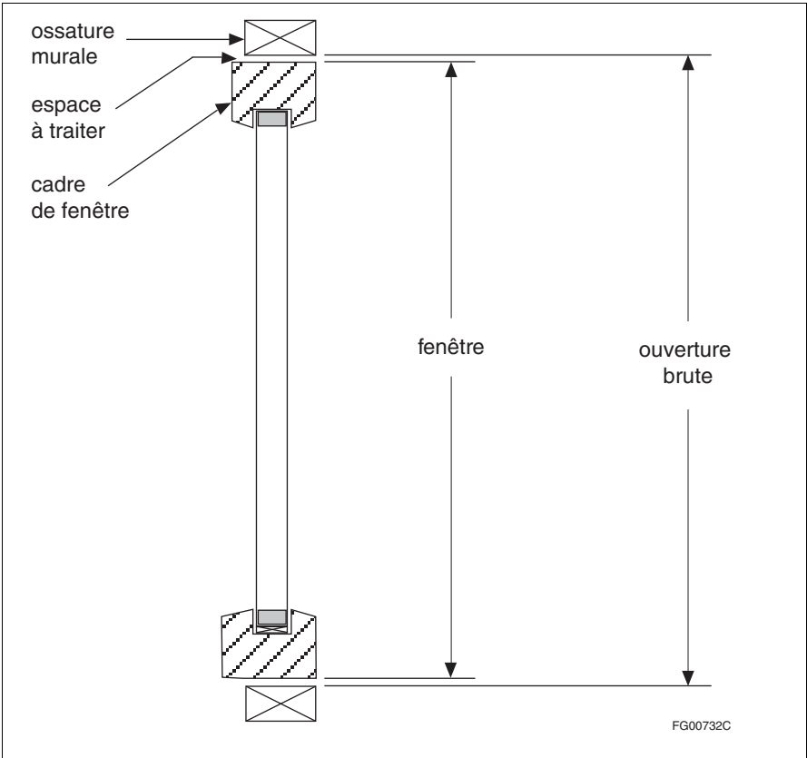
Figure A-3.2.1.2. 2) Espace entre le cadre de fenêtre et l'ouverture brute dans l'ossature murale
