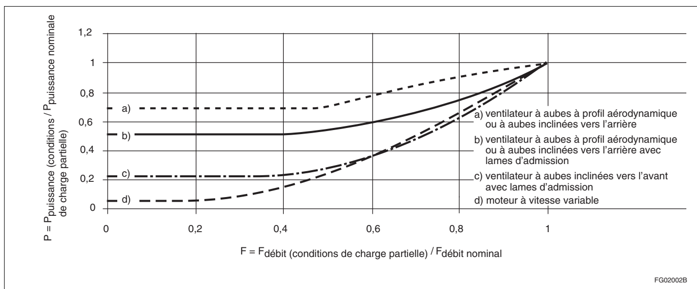
Figure A-8.4.5.17. 2) Courbes des charges partielles des ventilateurs
