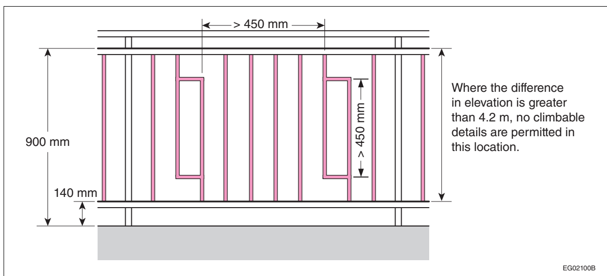
Figure A-9.8.8.6.(1)-A
