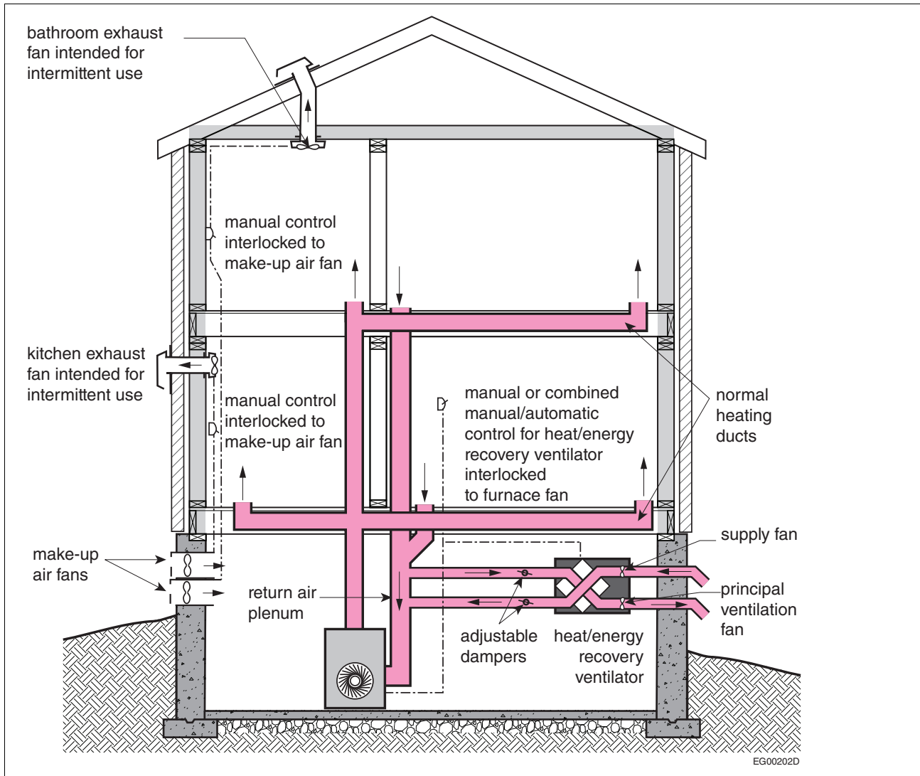
Figure A-9.32.3.3.-B
