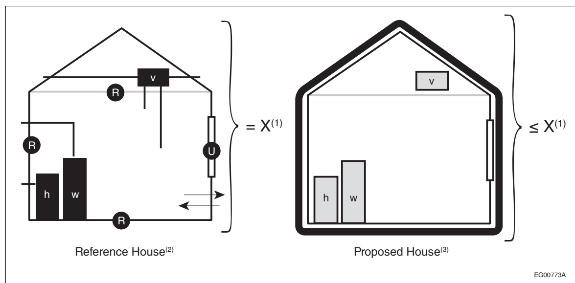
Figure A-9.36.6.3.(2)
