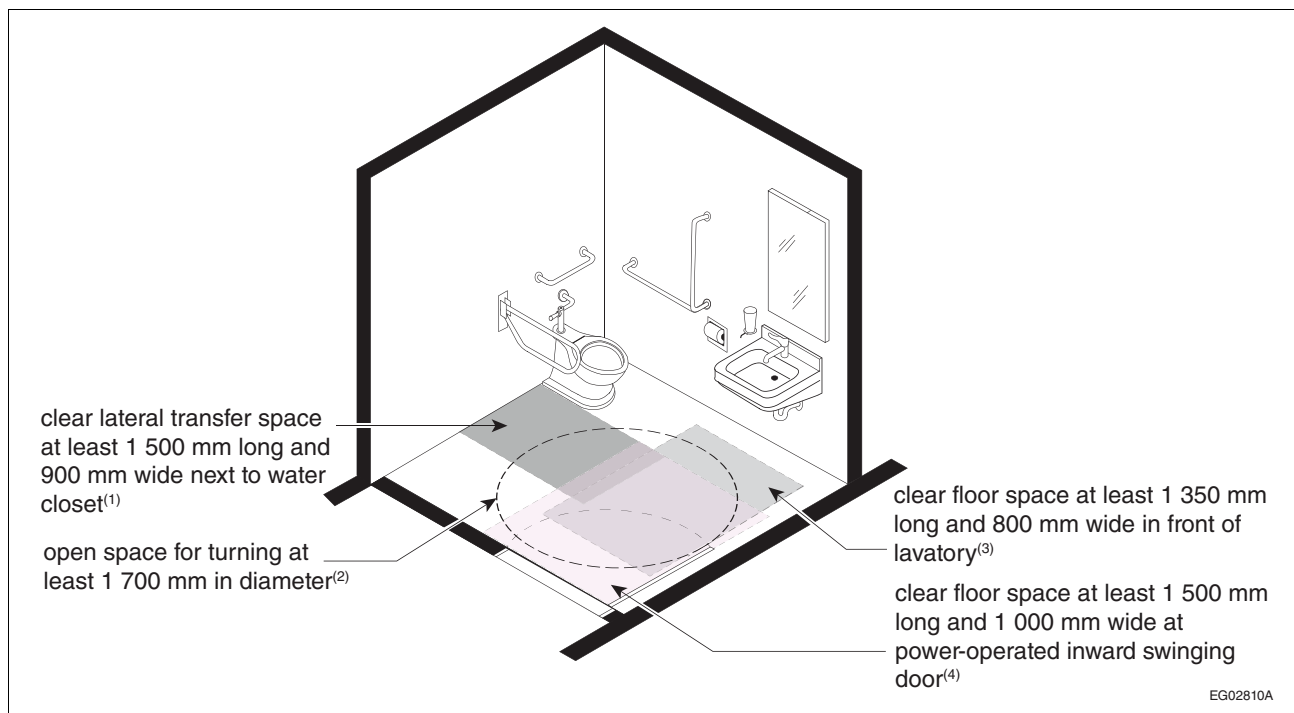
Figure A-3.8.3.13.-B
