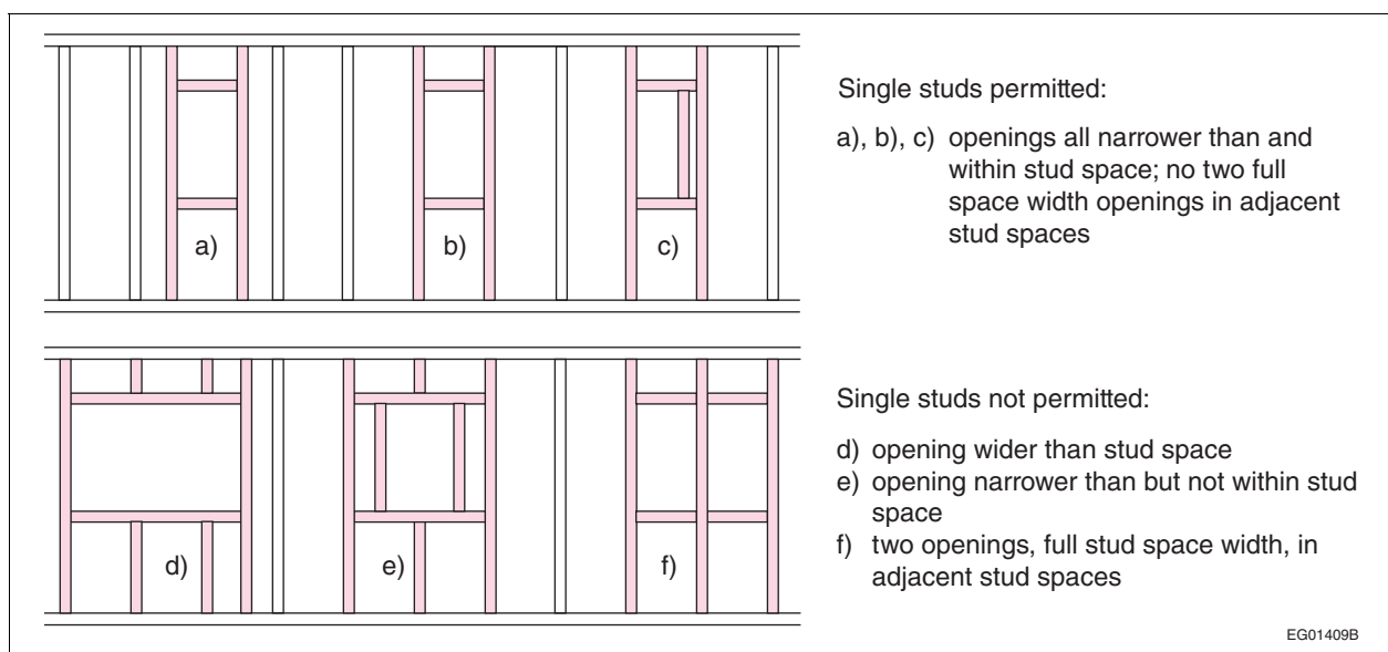
Figure A-9.23.10.6.(3)-B
