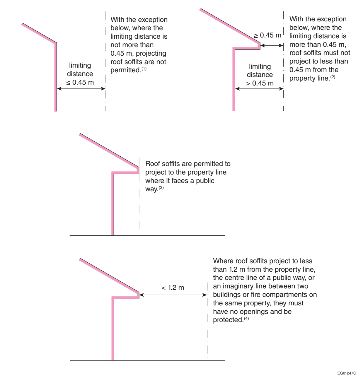
Figure A-9.10.14.5.(11) and 9.10.15.5.(10)
