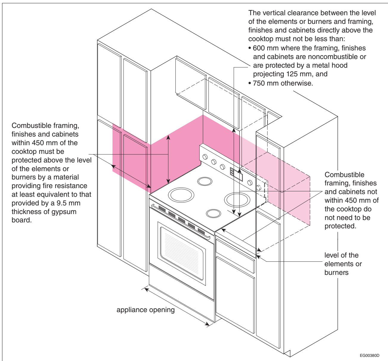
Figure A-9.10.22.
