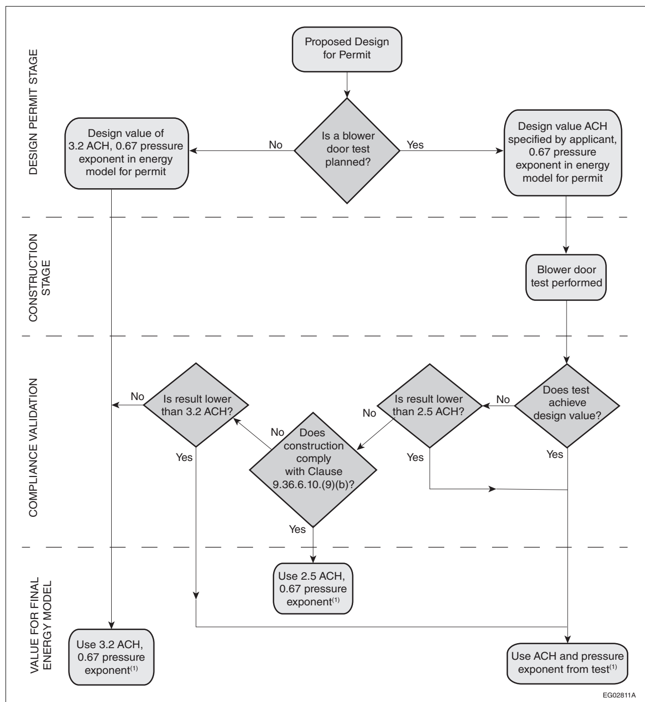
Figure A-9.36.7.3.(7)
