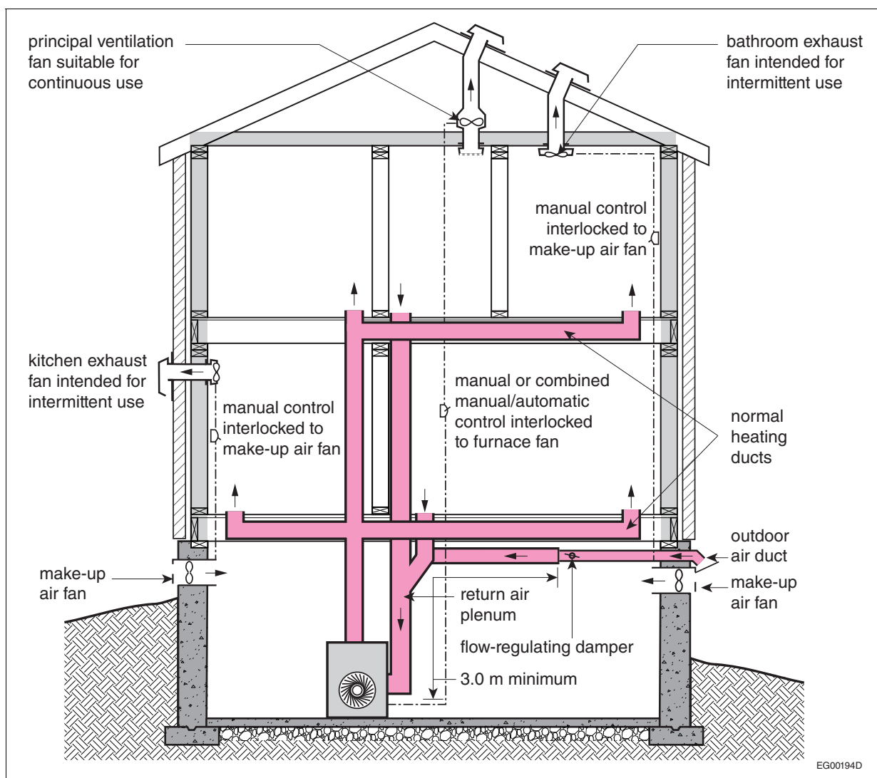
Figure A-9.32.3.3.-A
