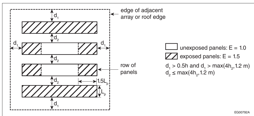
Figure A-4.1.7.13.
