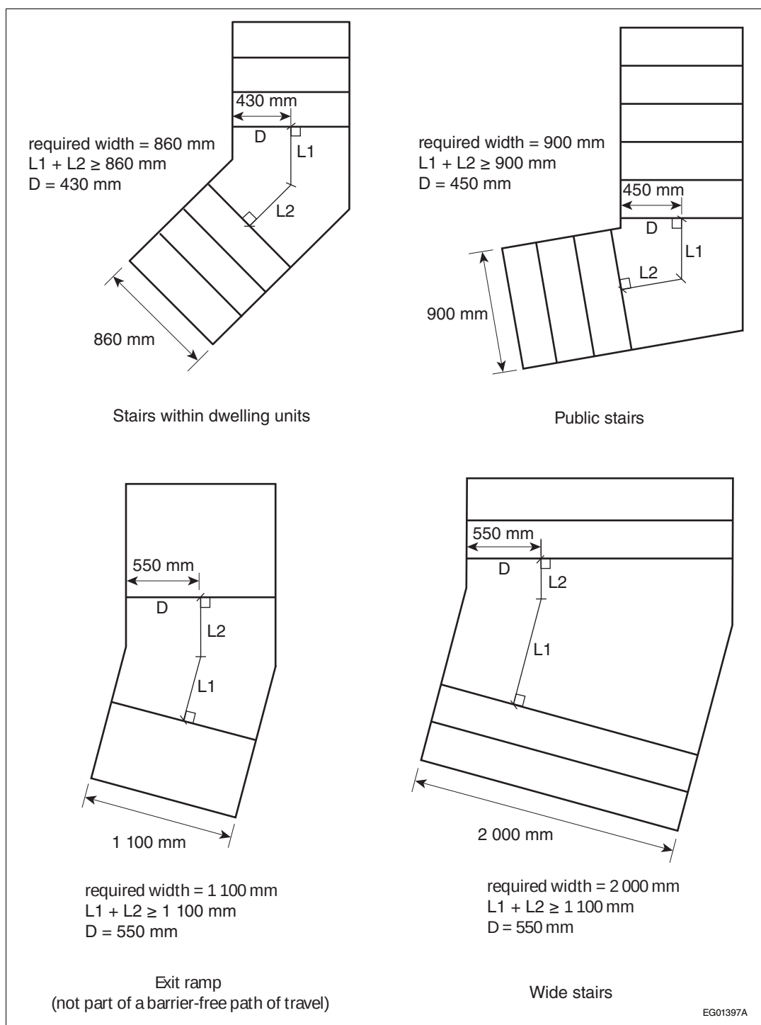
Figure A-3.4.6.4.
