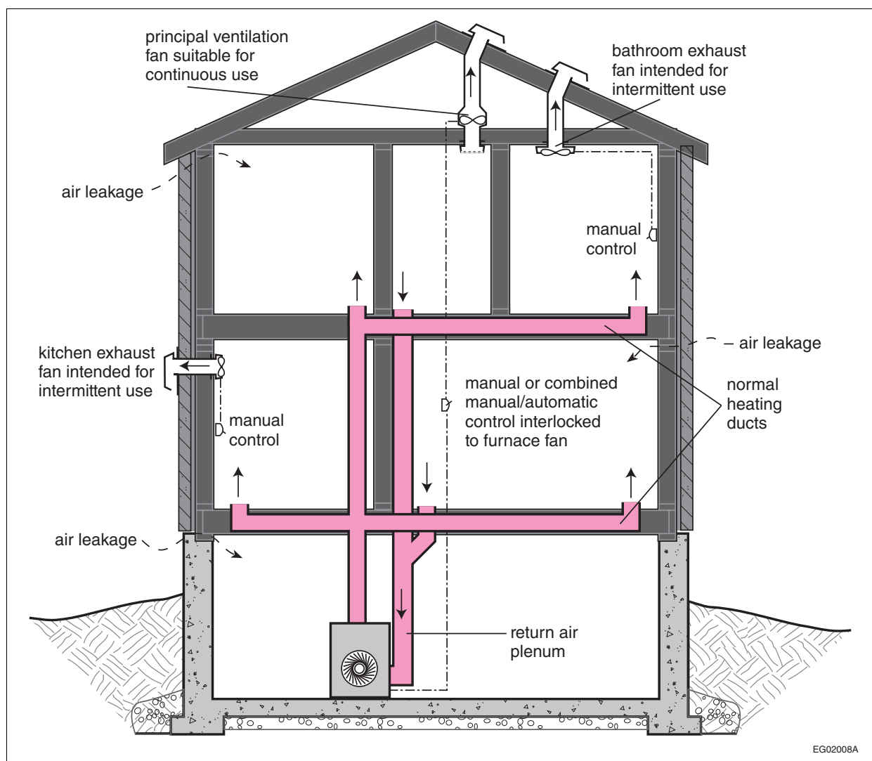
Figure A-9.32.3.6.
