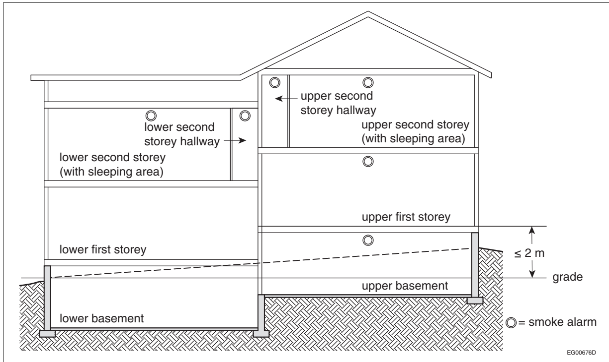
Figure A-9.10.19.3.(1)
