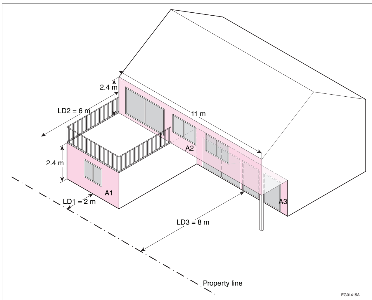
Figure A-9.10.15.4.(2)-D
