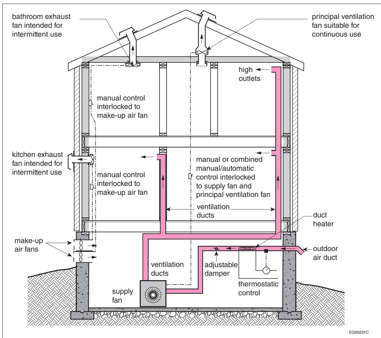
Figure A-9.32.3.3.-C
