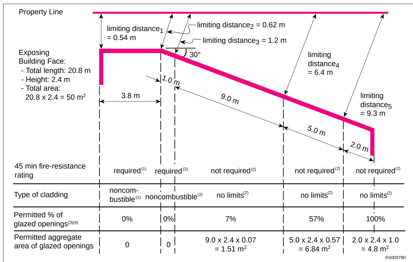
Figure A-9.10.15.4.(2)-C
