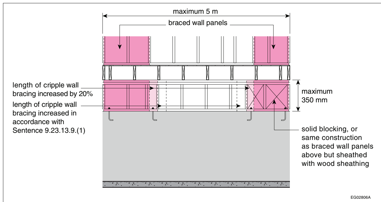
Figure A-9.23.13.10.(3).
