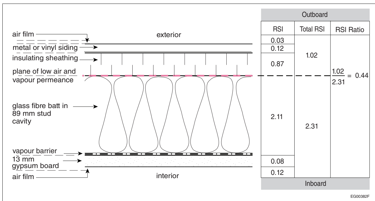
Figure A-9.25.5.2.
