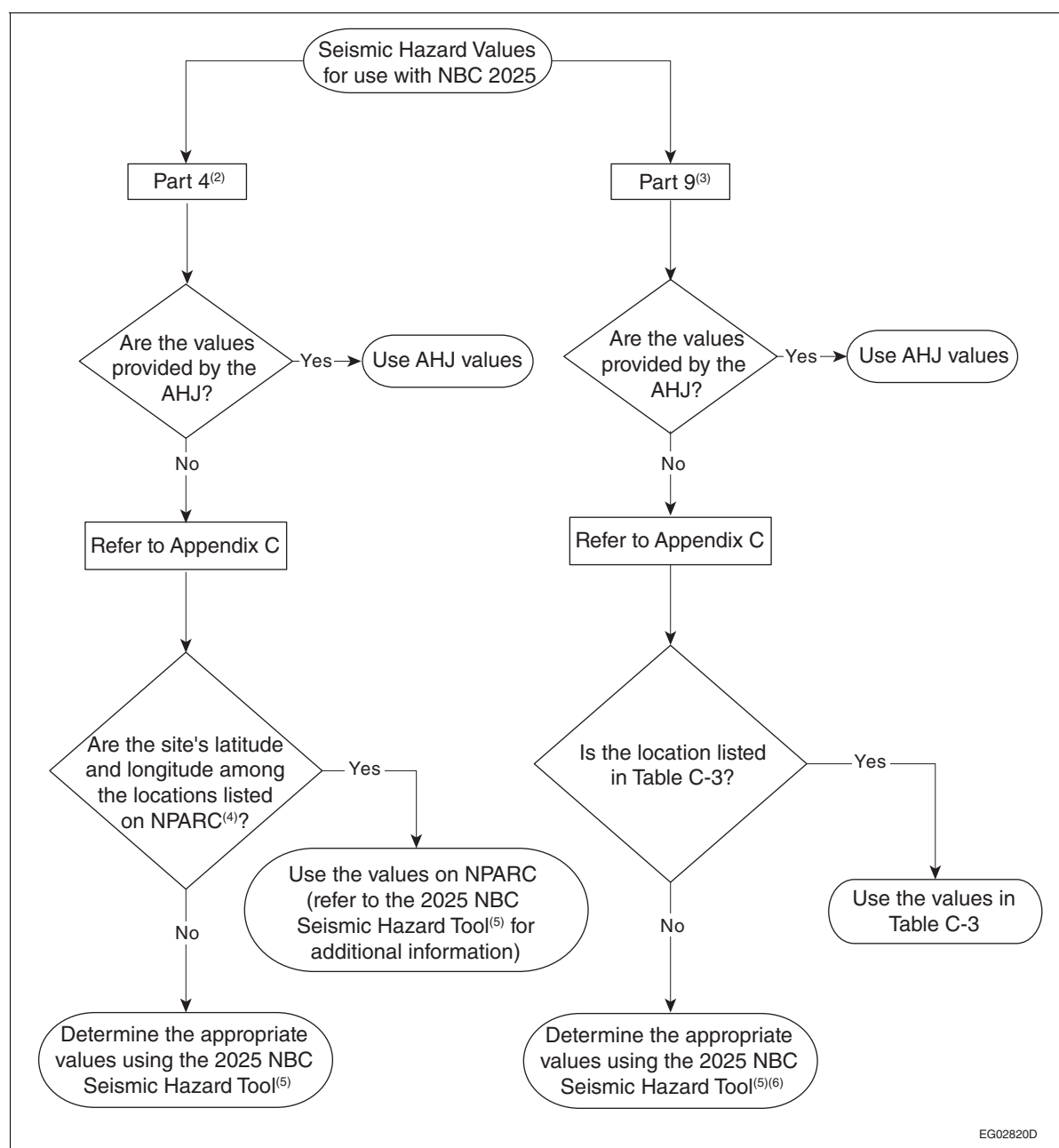
Figure A-1.1.3.1.(4)
