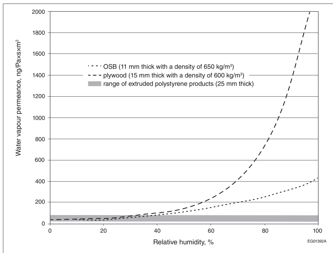
Figure A-9.25.5.1.(3)
