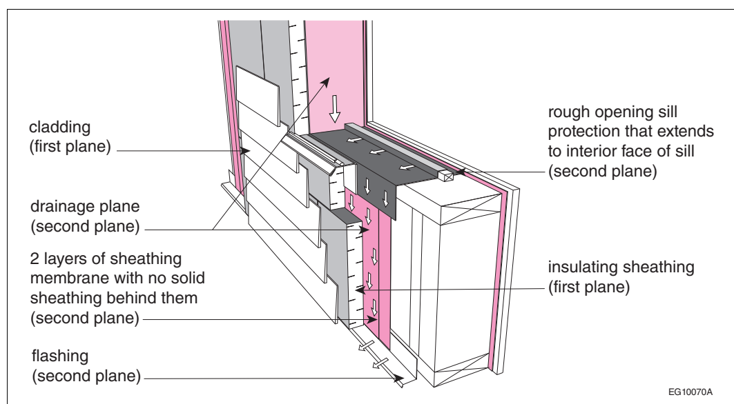
Figure A-9.27.2.-D
