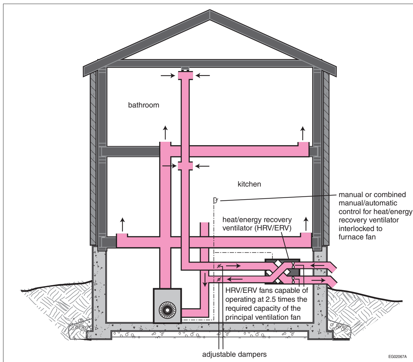
Figure A-9.32.3.3.-F
