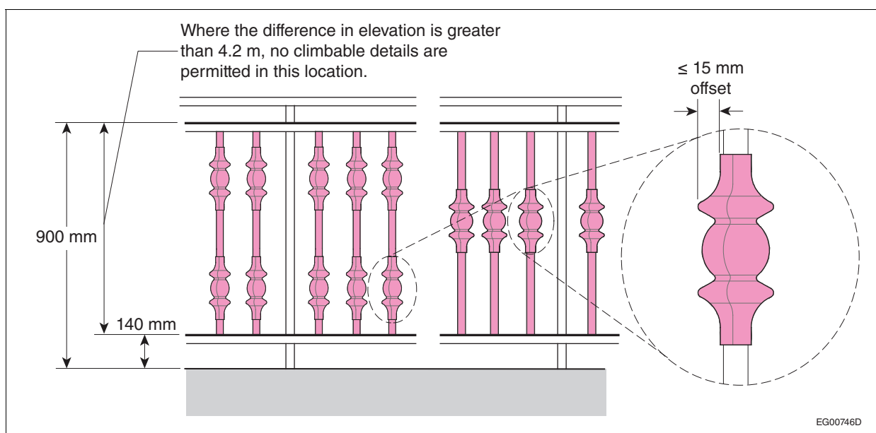
Figure A-9.8.8.6.(1)-B
