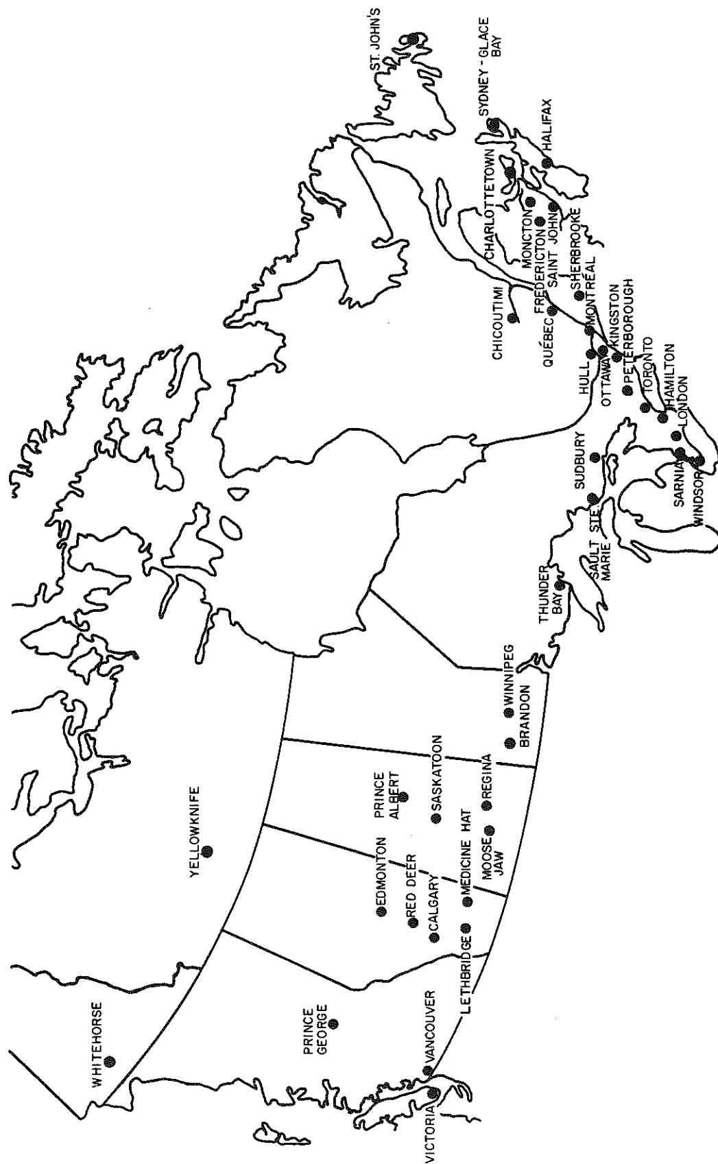
NATIONAL AIR POLLUTION SURVEILLANCE NETWORK ( JANUARY, 1974 ) RÉSEAU NATIONAL DE SURVEILLANCE DE LA POLLUTION ATMOSPHÉRIQUE ( JANVIER, 1974 )
