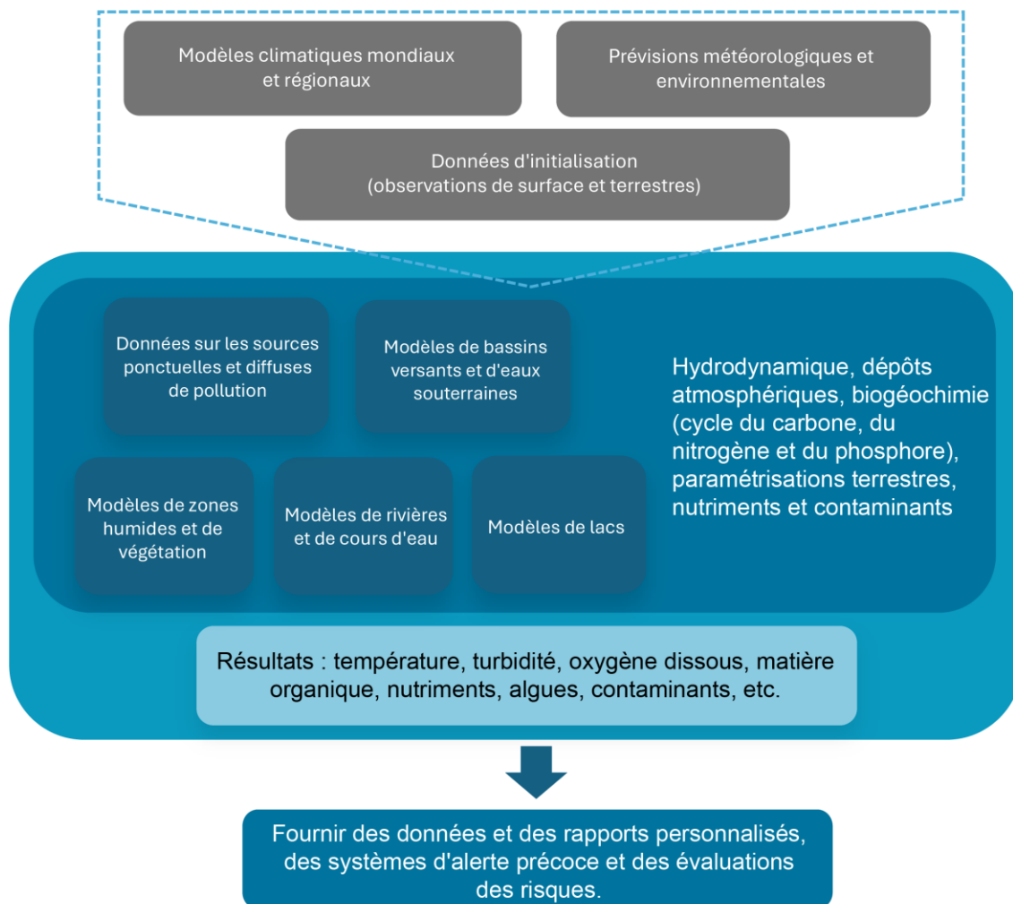
Figure 8-2: Les composants de base d'une stratégie de modélisation de la qualité de l'eau douce.
