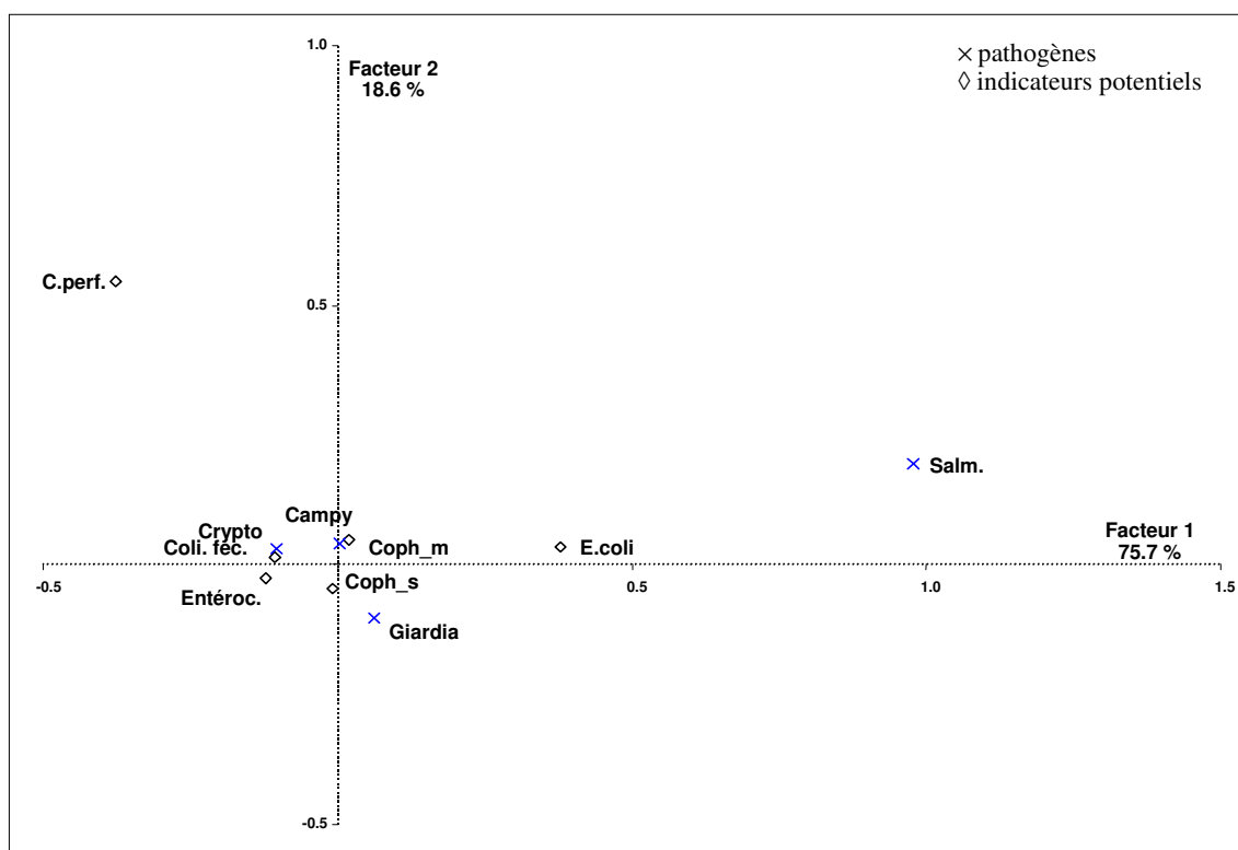
Figure 4.2 Projection des coordonnées des indicateurs potentiels et des pathogènes sur les deux premiers facteurs de l'analyse des correspondances
