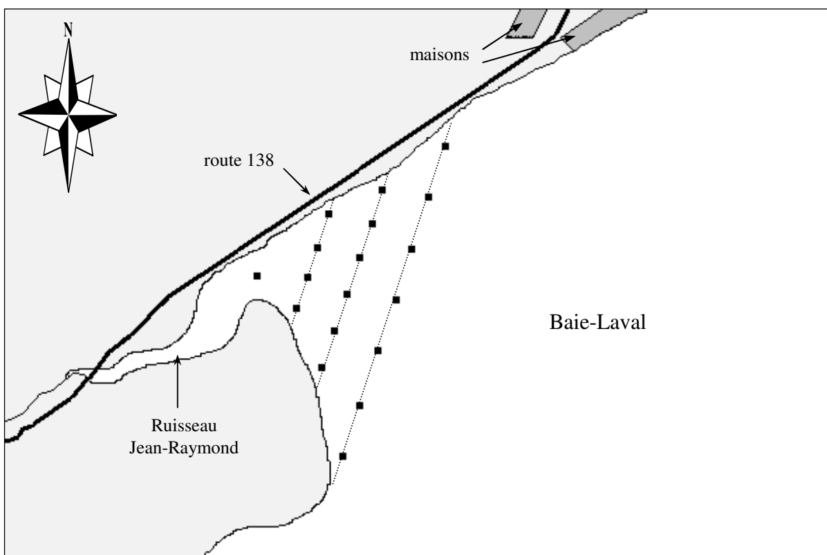
Figure 3.2 Carte de Baie-Laval illustrant les dix-huit points d'échantillonnage de l'eau
