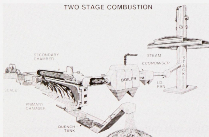
Schéma d'un incinérateur municipal de déchets solides
