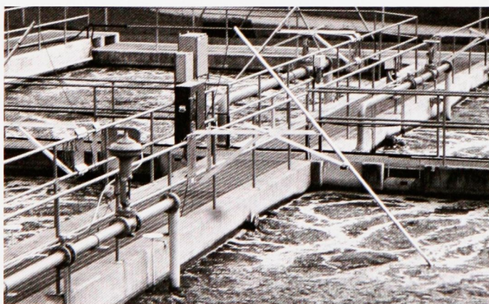
Le contrôle des teneurs en oxygène dissous indique jusqu'à 30 % d'économie sur les coûts énergétiques des usines de traitement.
