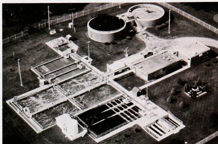
Démonstration réussie d'une commande automatique par ordinateur, avec capteurs, à l'usine de traitement des eaux usées de Tillsonburg
