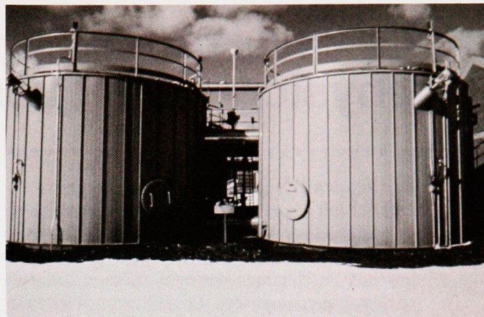
Les systèmes de digestion aérobie autothermique aident les petites communautés à réduire les coûts d'élimination des boues.
