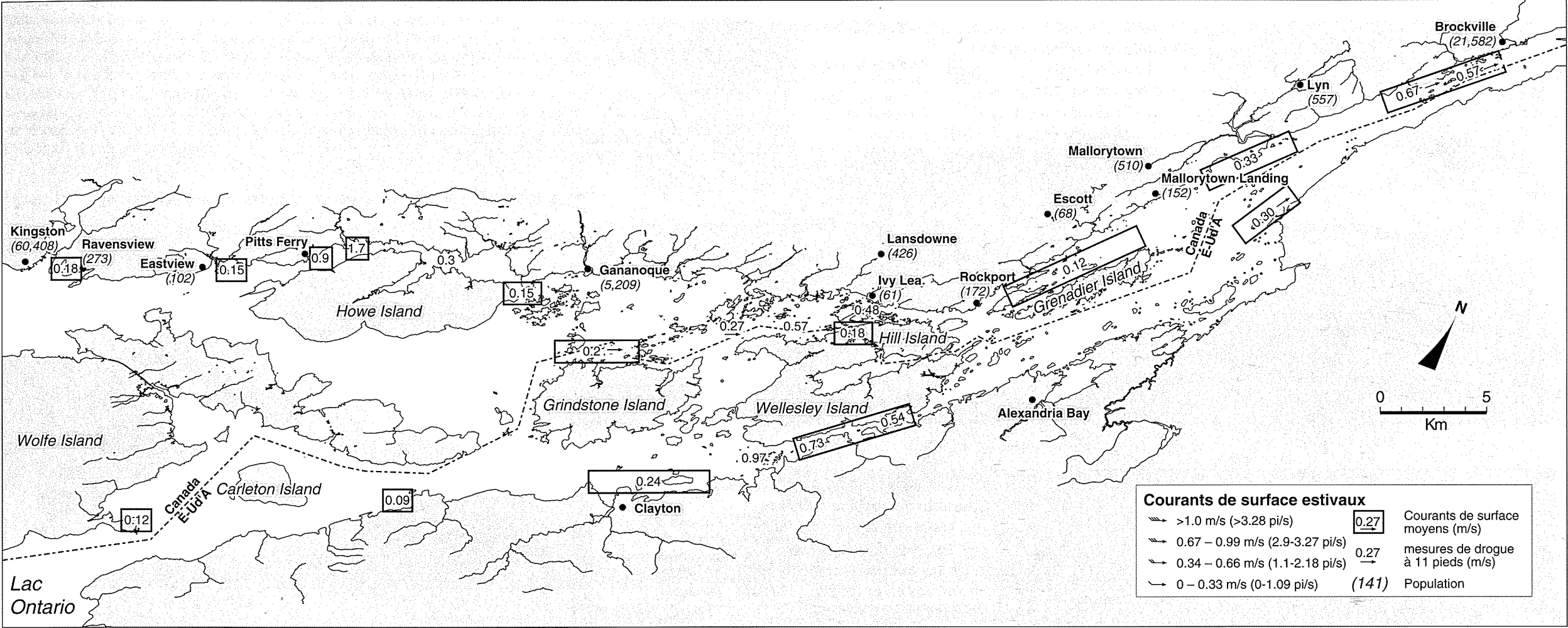
Figure 3. Aperçu de fleuve Saint-Laurent, et courants de surface
