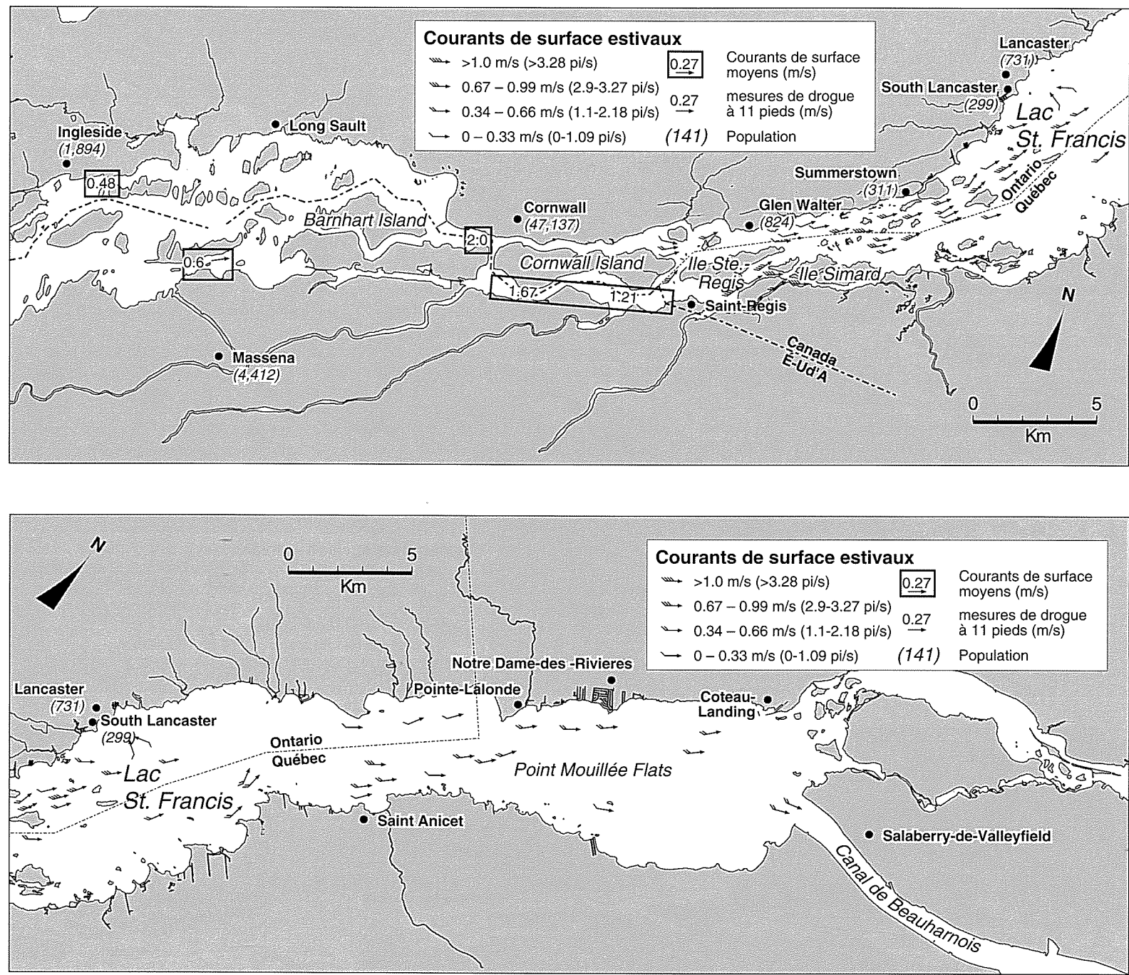
Figure 3. Aperçu de fleuve Saint-Laurent et courants de surface
