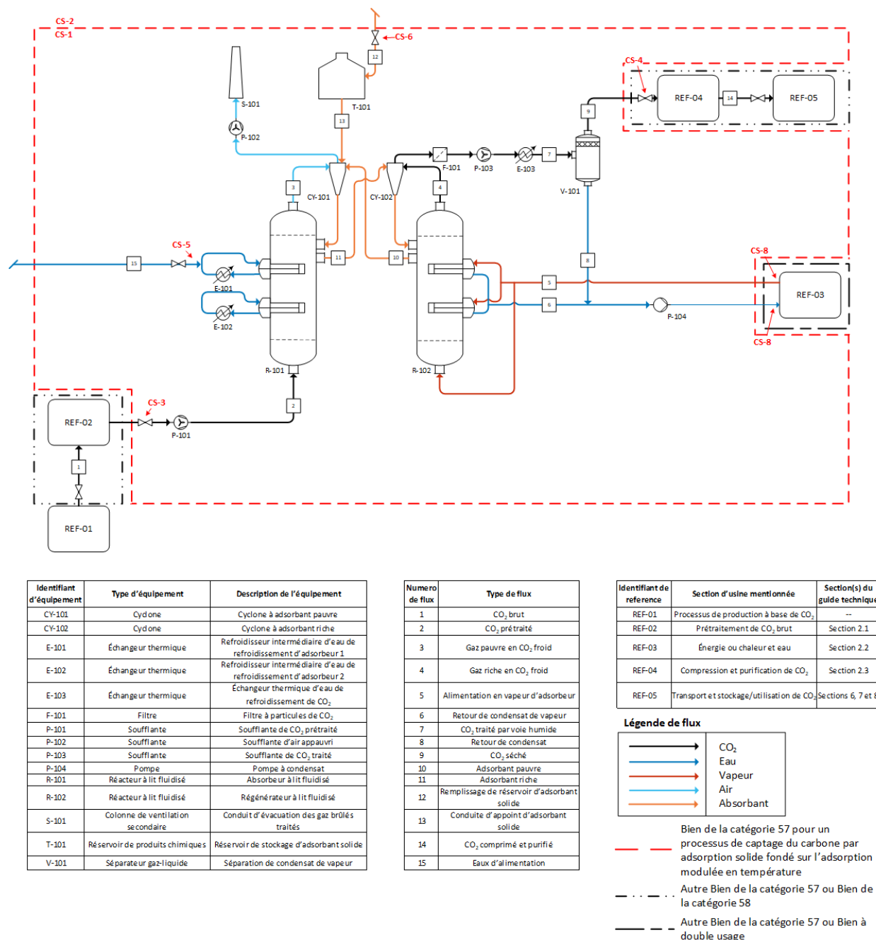
Figure 3.2-2 : Exemple d'un processus de captage du carbone par adsorption solide fondée sur l'adsorption modulée en température.
