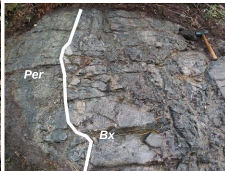
Brèche à matrice d'harzburgite à Pl et enclaves de norite, webstérite et paragneiss, en contact transitionnel avec péridotites (secteur du Lac Nadeau)
