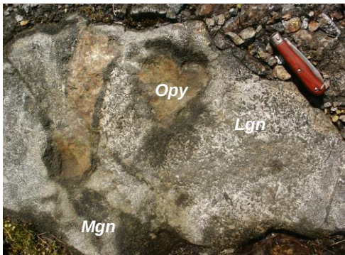
Enclaves d'orthopyroxénite à Pl et enclaves de leucogabbro-norite dans des mélagabbro-norites (intrusion Rochette Ouest)
