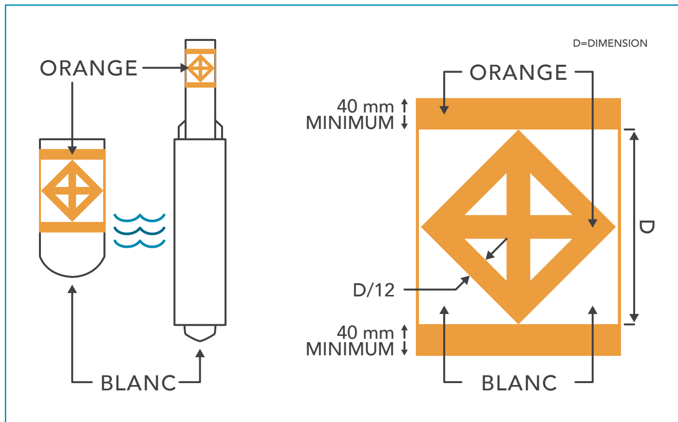
FIGURE 9 BOUÉE D'ENDROIT INTERDIT
