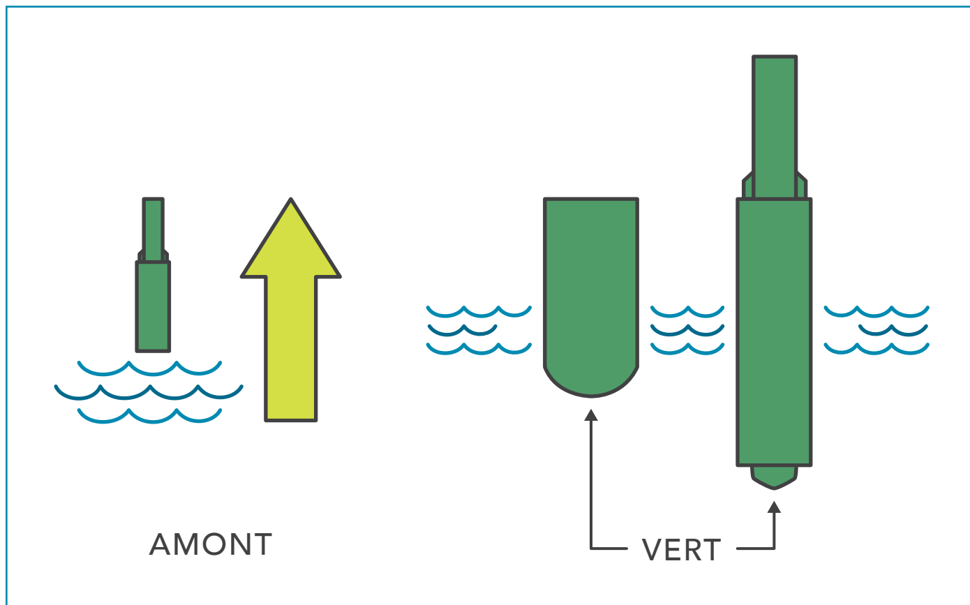
FIGURE 1 BOUÉE DE BÂBORD
