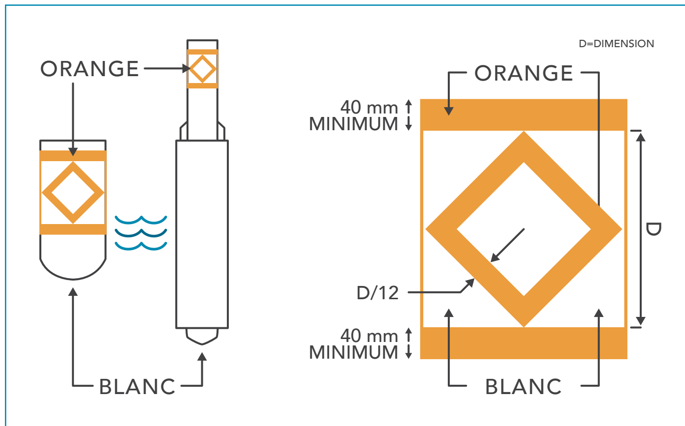
FIGURE 4 BOUÉE D'OBSTACLE
