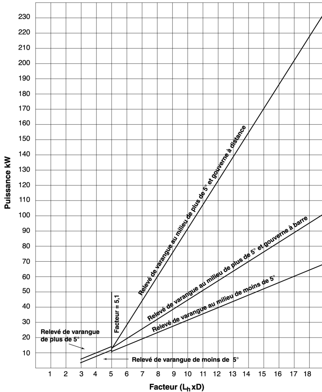
Figure 4-2 GRAPHIQUE PERMETTANT D'INTERPOLER LA PUISSANCE MAXIMALE RECOMMANDÉE POUR LA CONSTRUCTION DES MONOCOQUES
