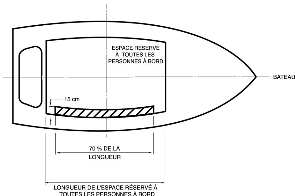
Figure 4-5 EMPLACEMENT DU CENTRE DE GRAVITÉ DES POIDS (essai de stabilité)
