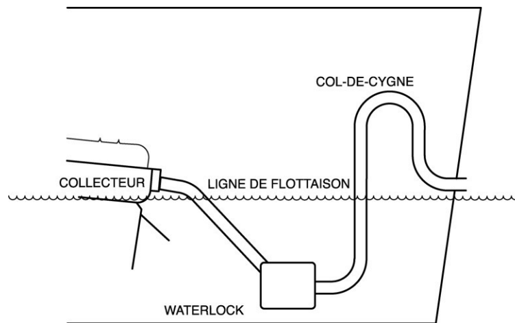
Figure 3-2 ÉCHAPPEMENT TYPIQUE À « WATERLOCK » SANS SILENCIEUX
