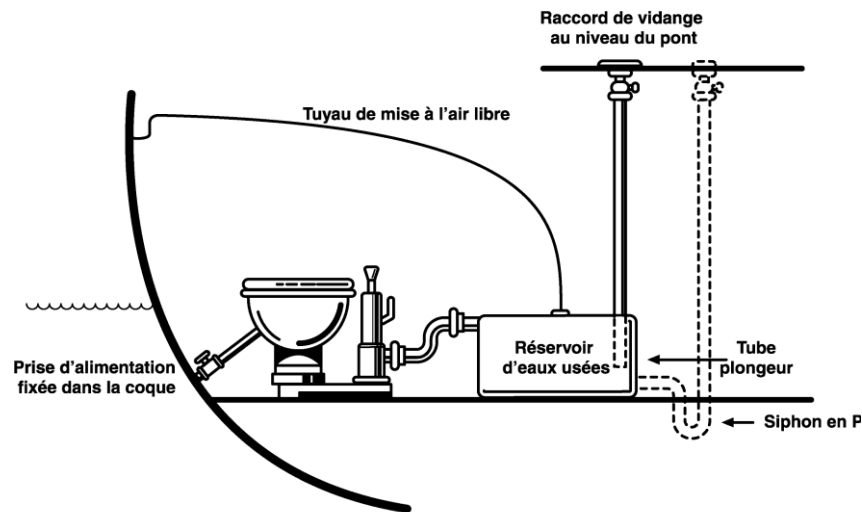
Figure 2-1 VIDANGE AU NIVEAU DU PONT SEULEMENT
