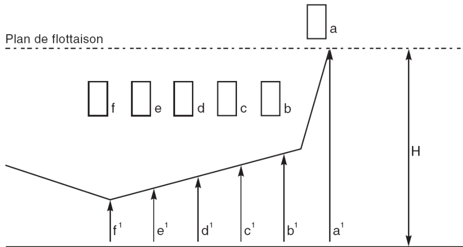
Figure 4-5 MESURE DE LA PROFONDEUR DU PETIT BÂTIMENT
