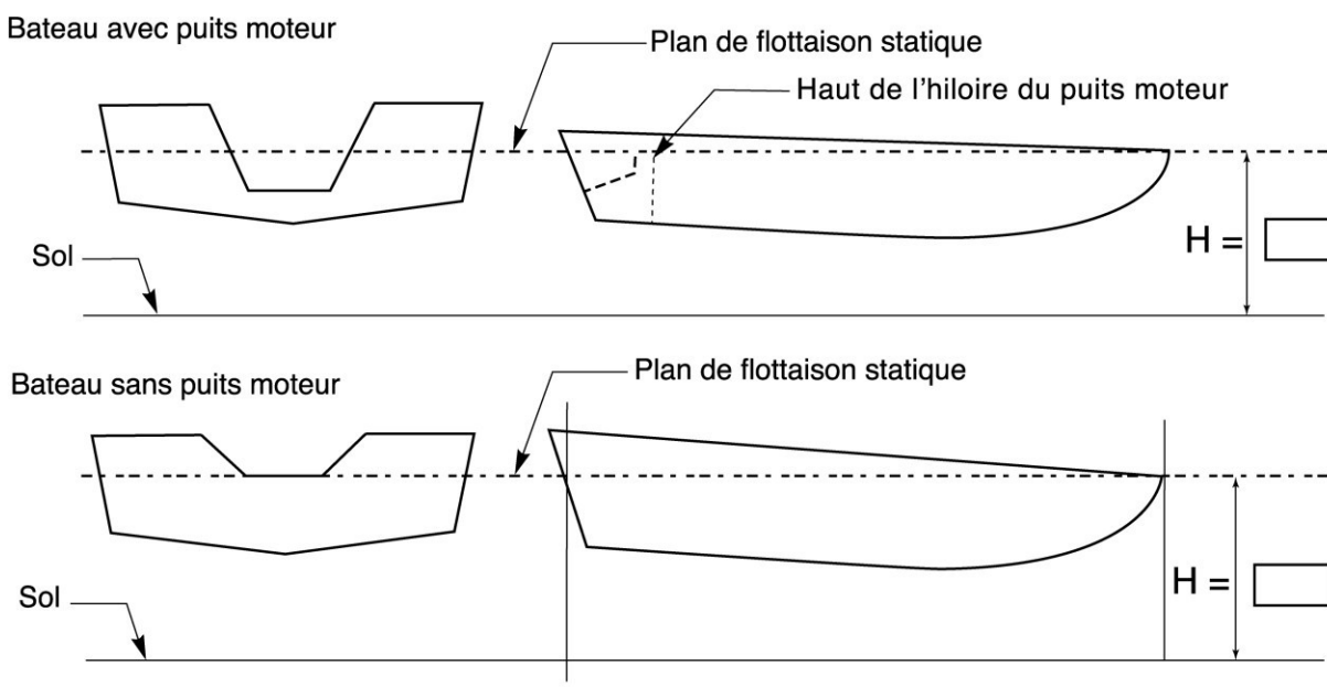
Figure 4-1 MESURAGE DES PETITS BÂTIMENTS MONOCOQUES
