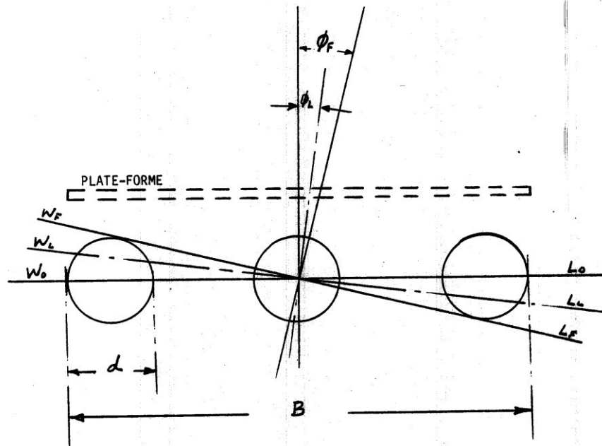
Figure 5-2 FRANC-BORD ET ANGLE DE GÎTE LIMITE
