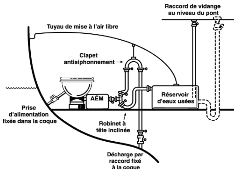
Figure 2-3 APPAREIL D'ÉPURATION MARINE AVEC DÉCHARGE À LA MER EN AMONT DU RÉSERVOIR D'EAUX USÉES
