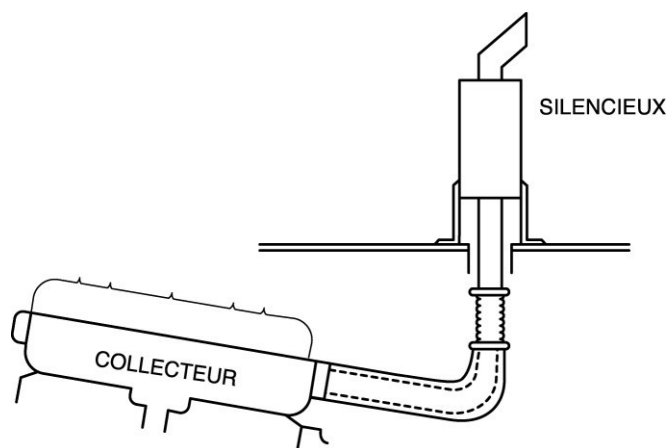
Figure 3-1 ÉCHAPPEMENT SEC TYPIQUE
