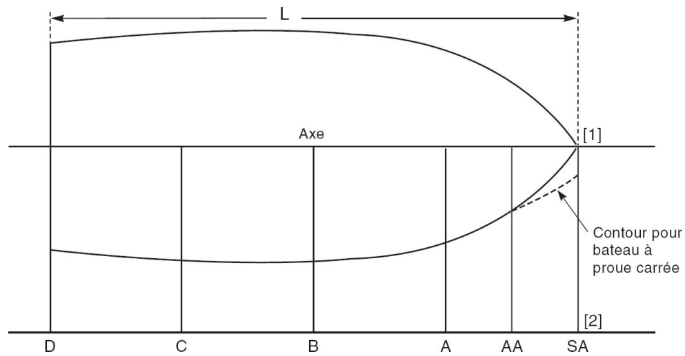
Figure 4-4 DEMI-SECTION TYPIQUE (AA, A, B, C, D) DES BÂTIMENTS
