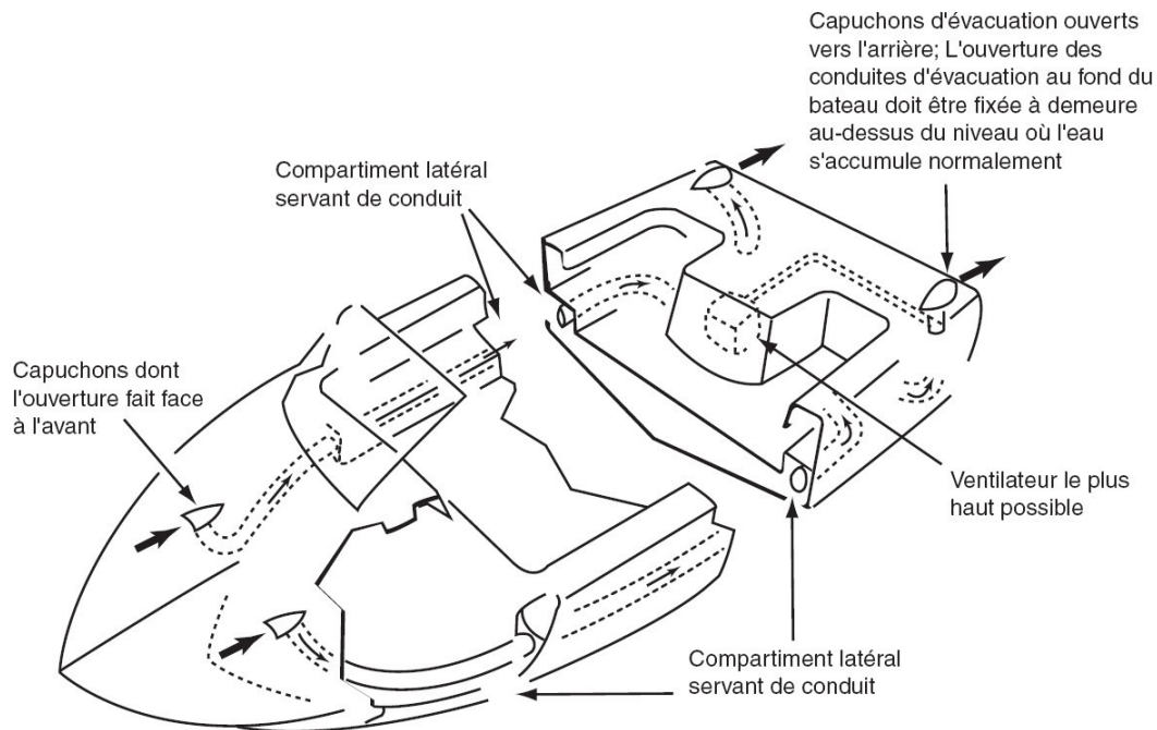
Figure 6-3 VENTILATION DES COMPARTIMENTS FERMÉS
