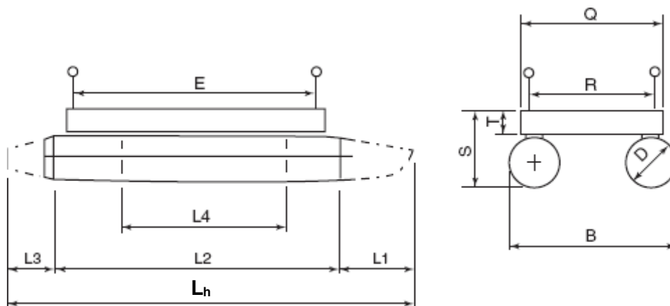
Figure 4-6 Dimensions des bâtiments de type ponton
