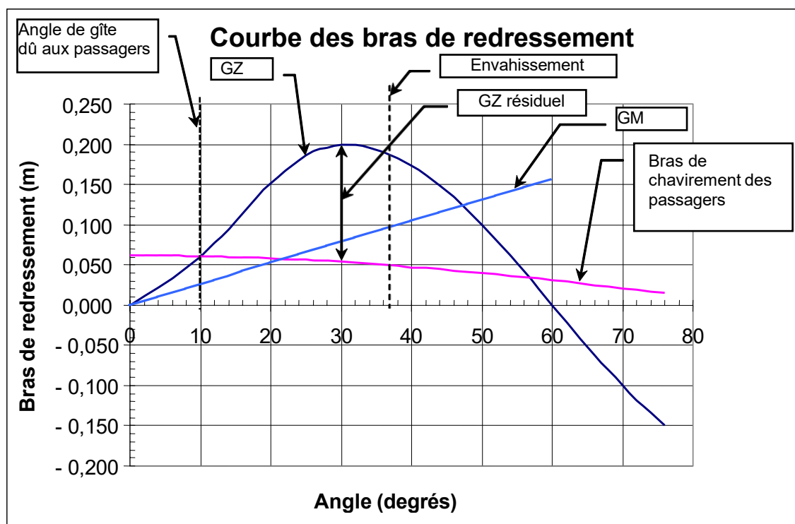
Figure 5-1 COURBE DES BRAS DE REDRESSEMENT
