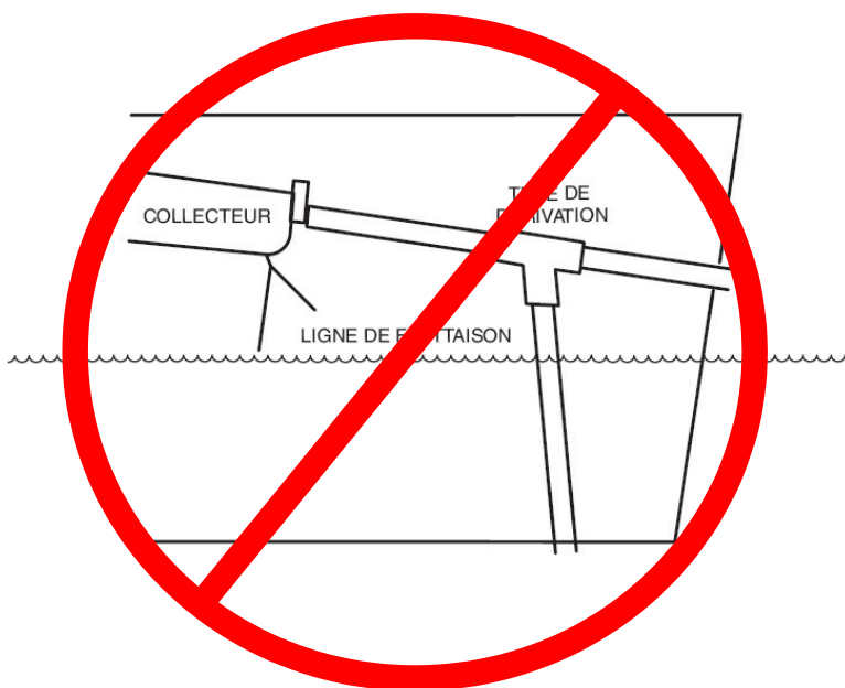
Figure 3-4 ÉCHAPPEMENT À HAUTE PERFORMANCE TYPIQUE AVEC TUYAU DE DÉRIVATION
