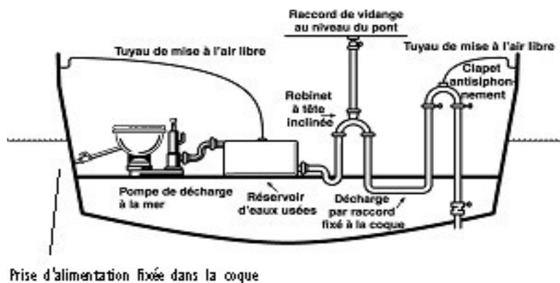
Figure 2-2 DÉCHARGE À LA MER EN AVAL DU RÉSERVOIR D'EAUX USÉES
