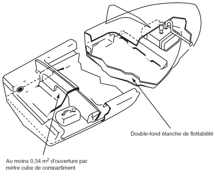
Figure 6-2 CARACTÉRISTIQUES DES COMPARTIMENTS OUVERTS
