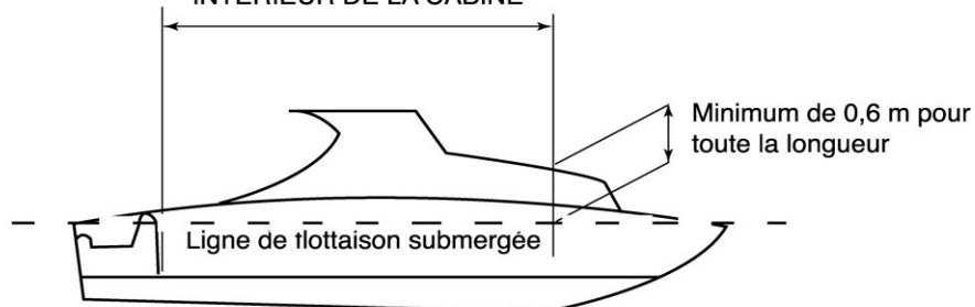
BATEAU AVEC CABINE
