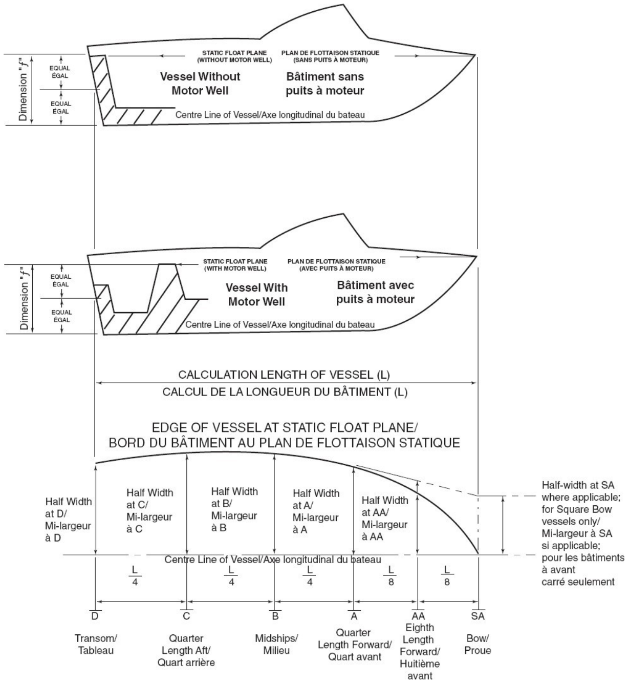
Figure 4-2 CALCUL DU MESURAGE DE LA LONGUEUR
