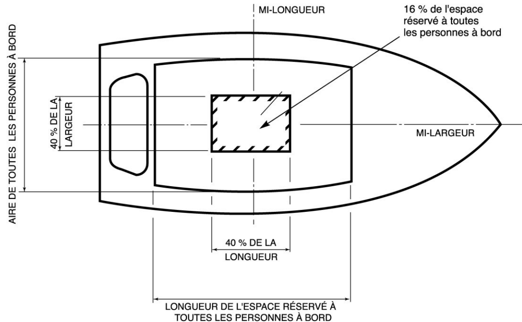
Figure 4-4 EMPLACEMENT DU CENTRE DE GRAVITÉ DES POIDS (flottaison à fleur d'eau)
