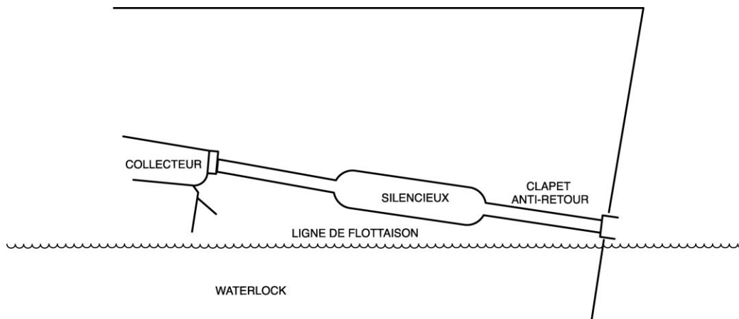
Figure 3-3 ÉCHAPPEMENT À HAUTE PERFORMANCE TYPIQUE
