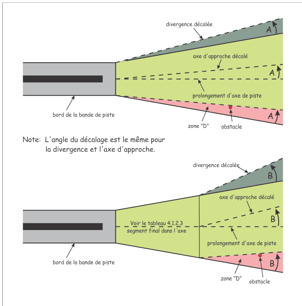
Figure 4-3 (b) : Surface d'approche décalée (piste a vue)
