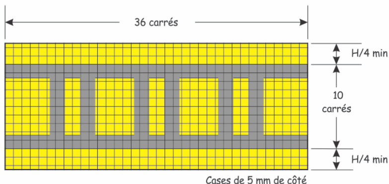
(a) Dégagement de piste - Cat I
