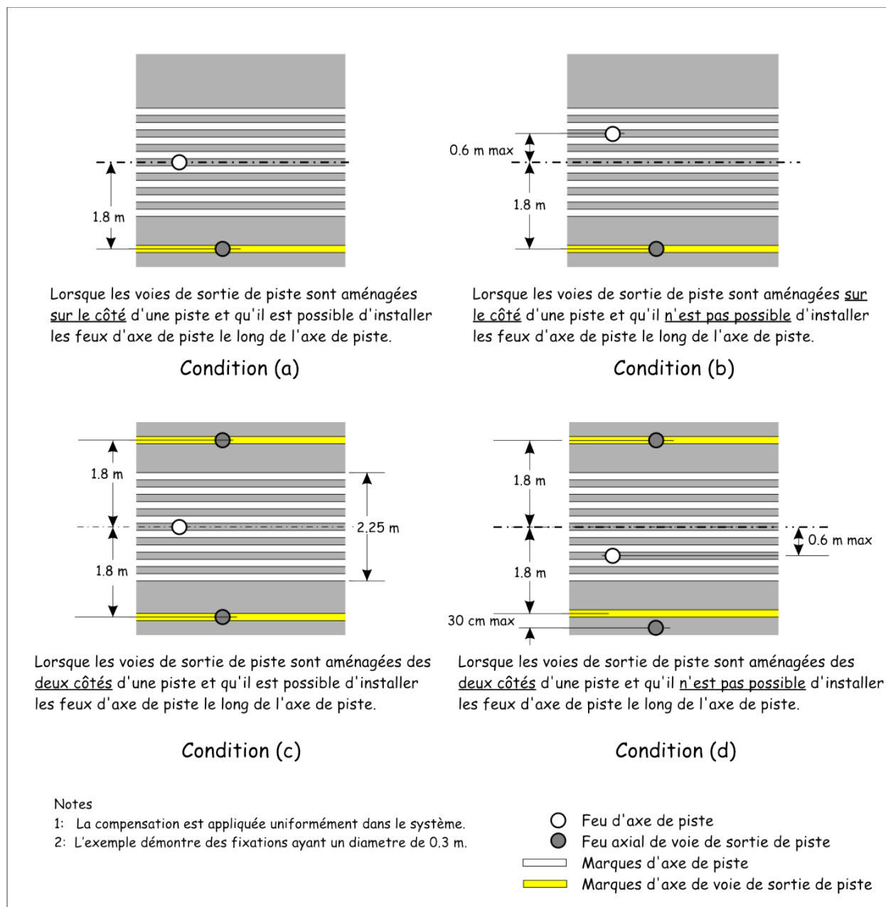
Figure 5-50 : Décalage des feux de piste et des feux d'axe de voie de circulation
