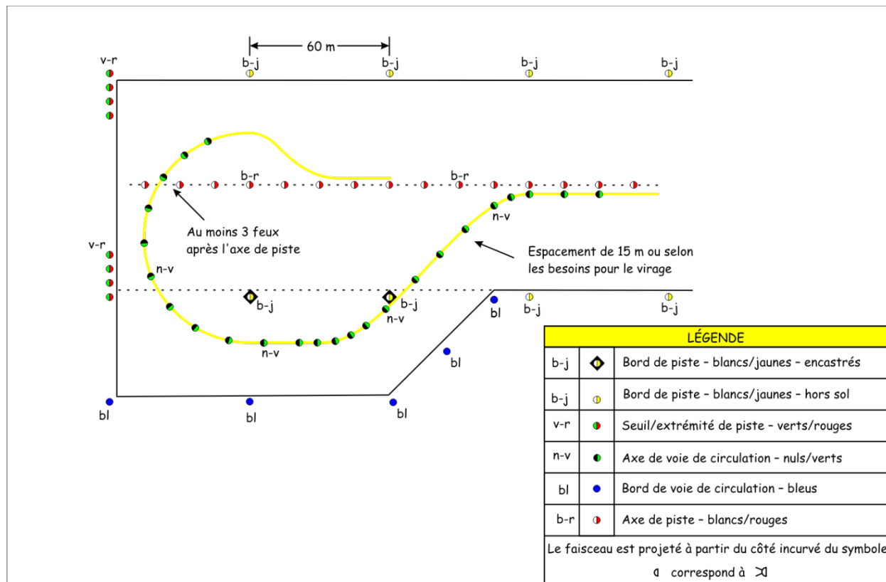
Figure 5-52 : Feux d'aire de retournement de piste
