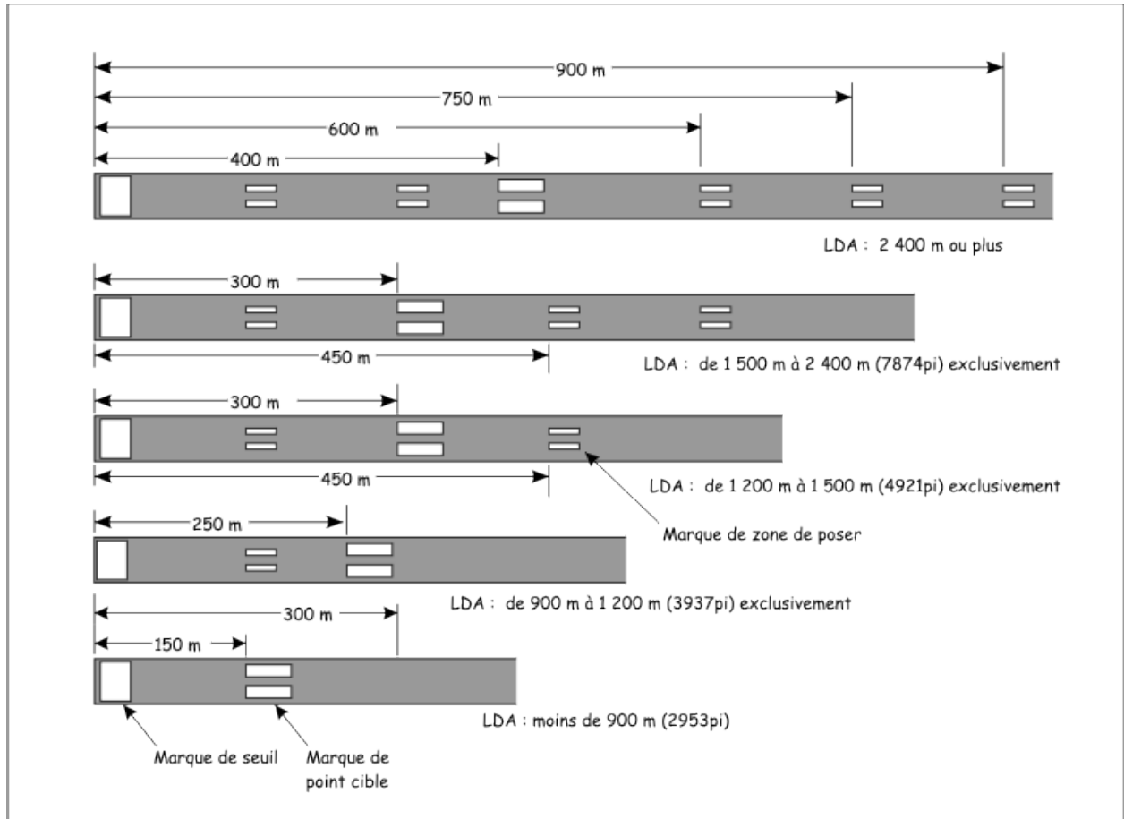
Figure 5-6 (b) : Marques de point de cible et zone de poser des roues
