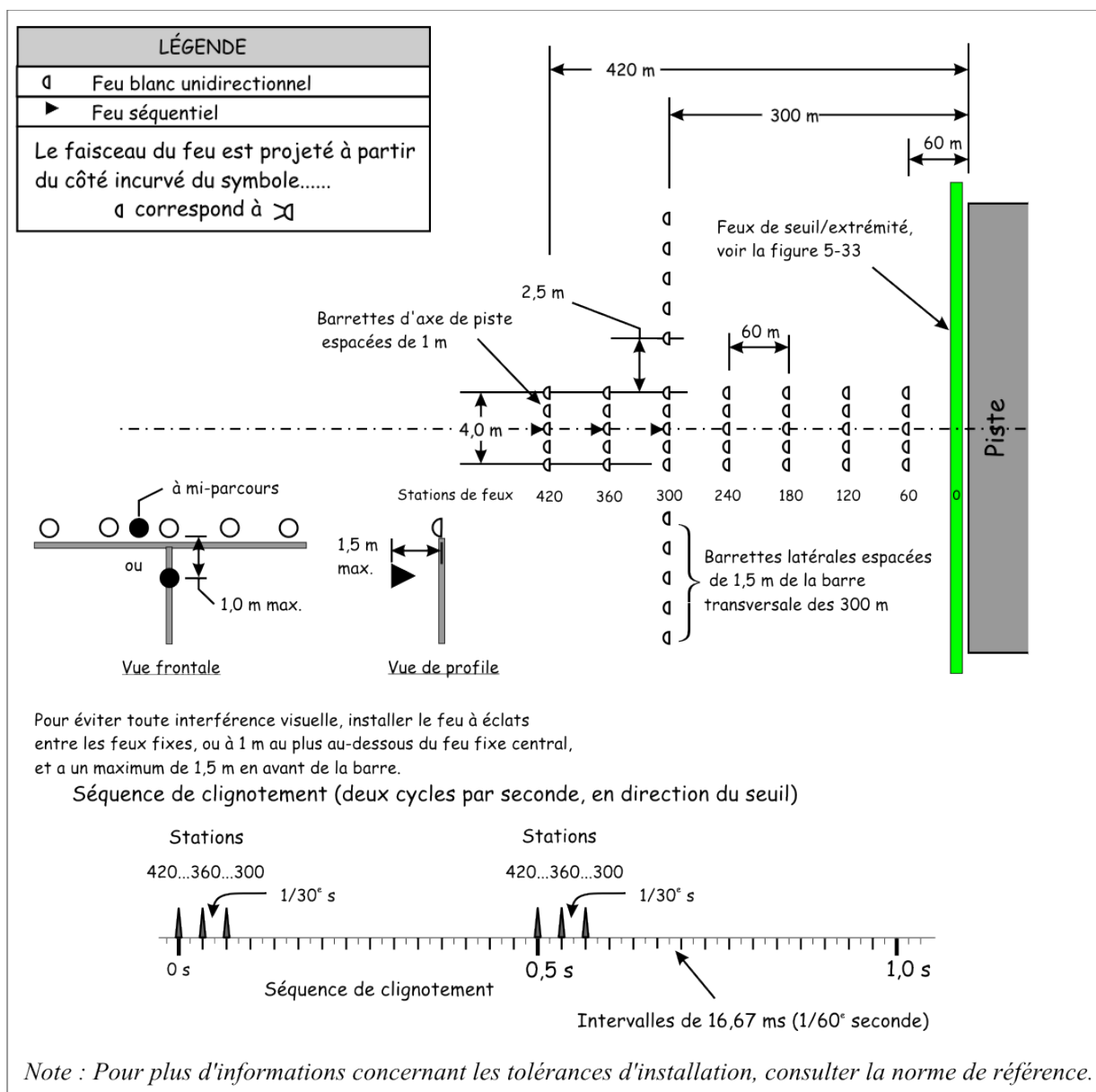
Figure 5-30 : Configuration du dispositif MALSF
