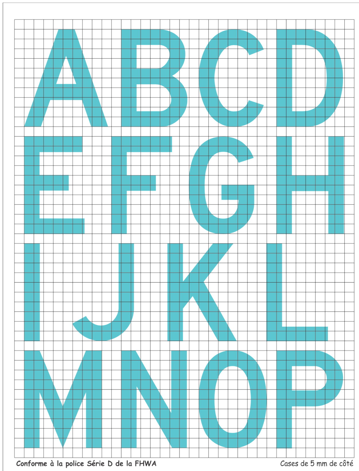
Figure 5-69 (a) : Proportions des caractères
