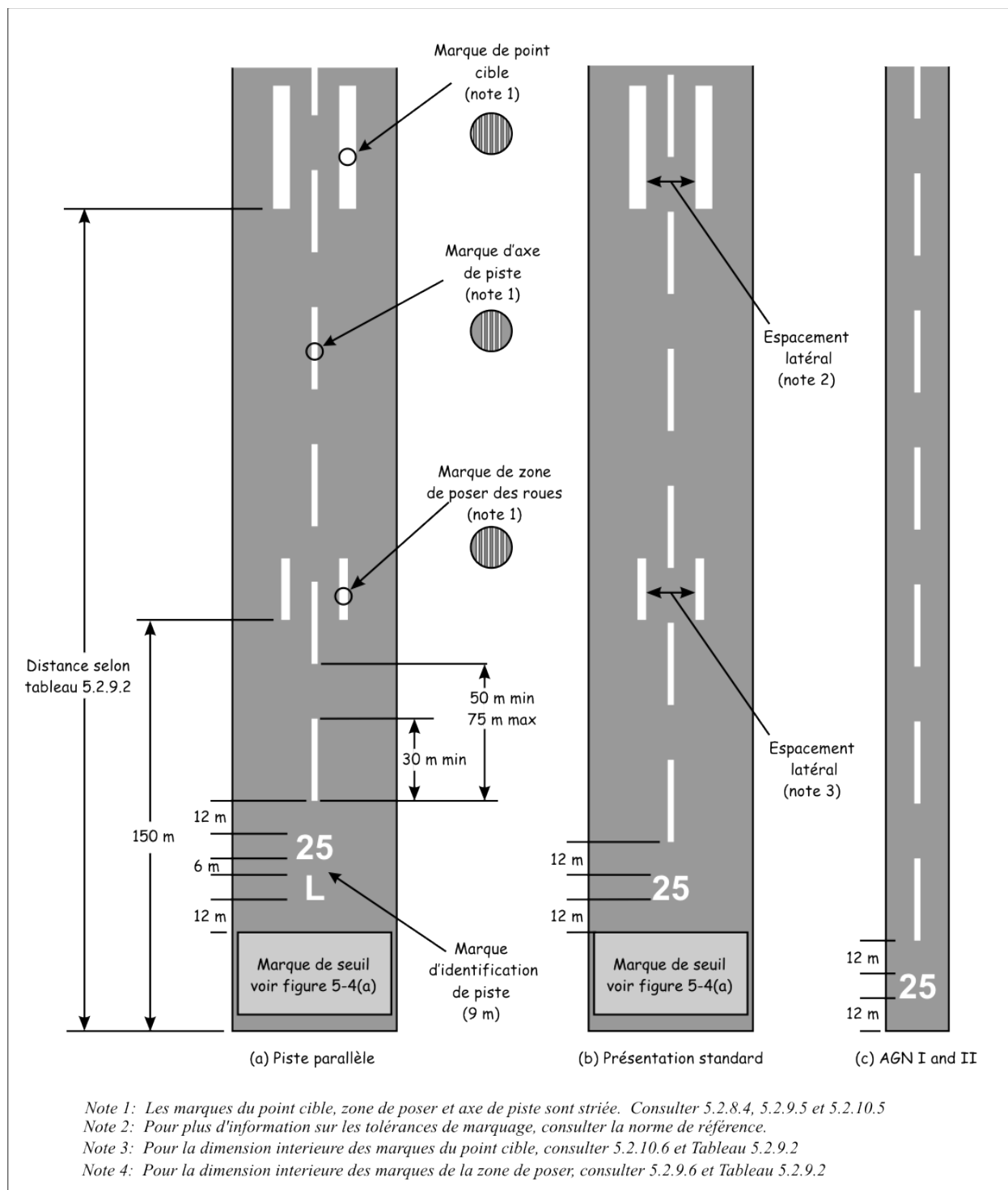
Figure 5-2 : Marques d'identification, d'axe et de seuil de piste
