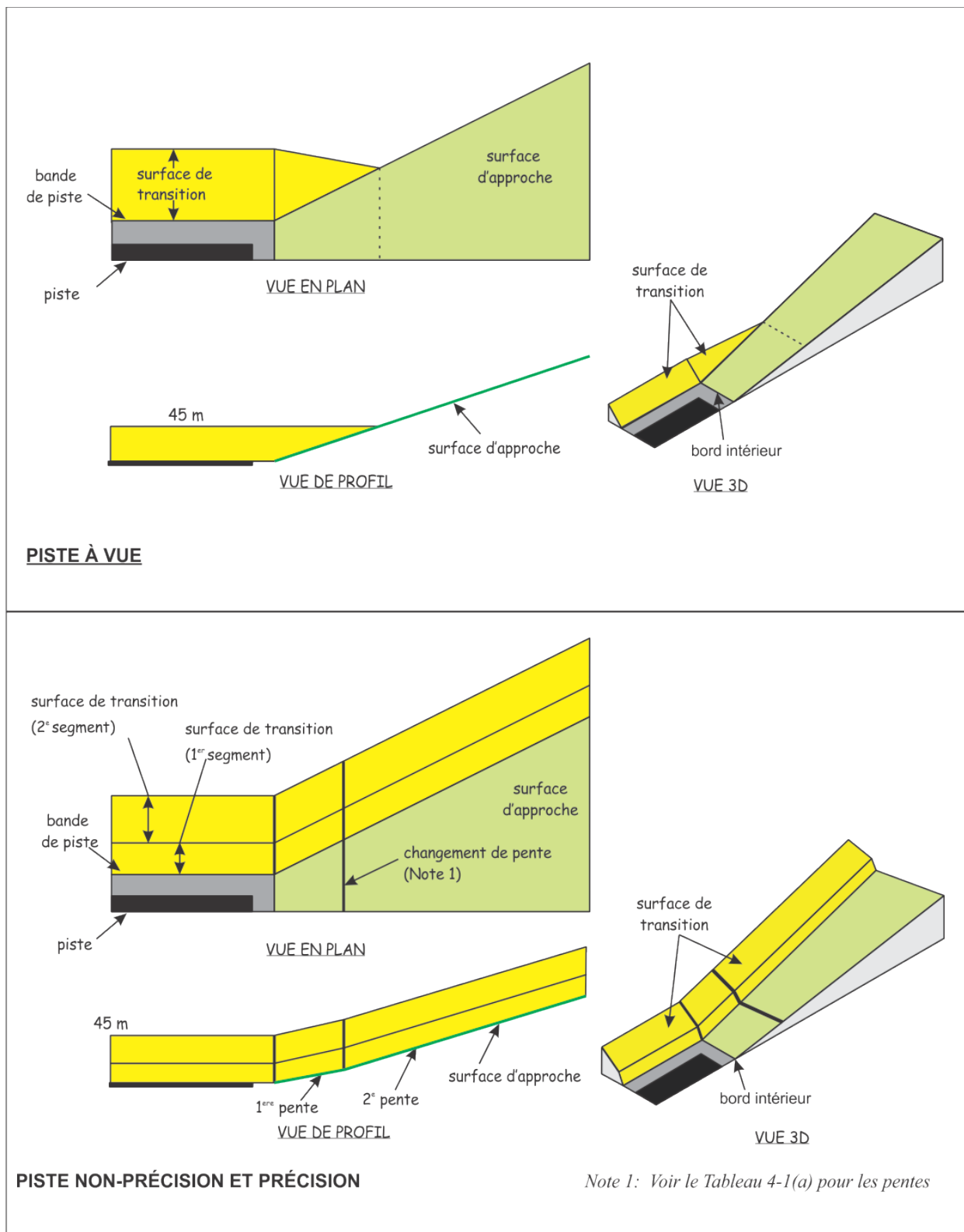
Figure 4-1 (a) : Surfaces de limitation d'obstacles (OLS)
