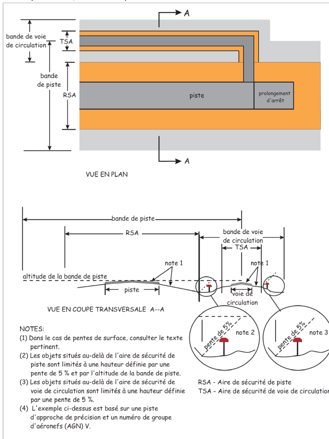
Figure 3-2 : Aire de sécurité de piste/voie de circulation
