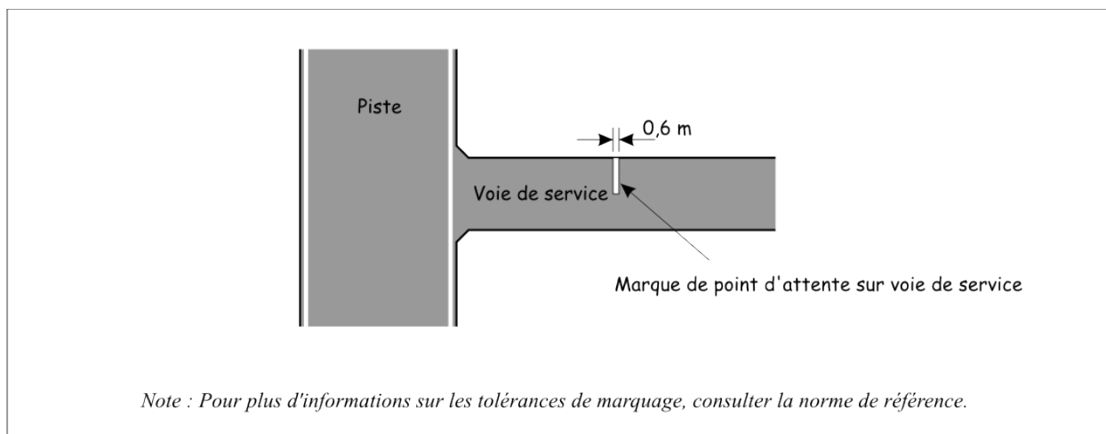
Figure 5-15 : Marques de point d'attente sur voie de service
