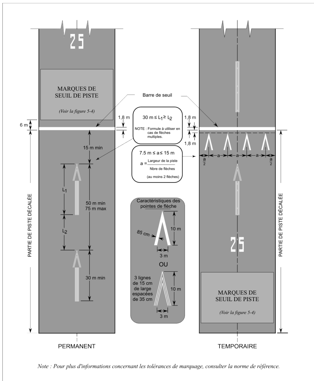
Figure 5-6 (a) : Marques de flèche
