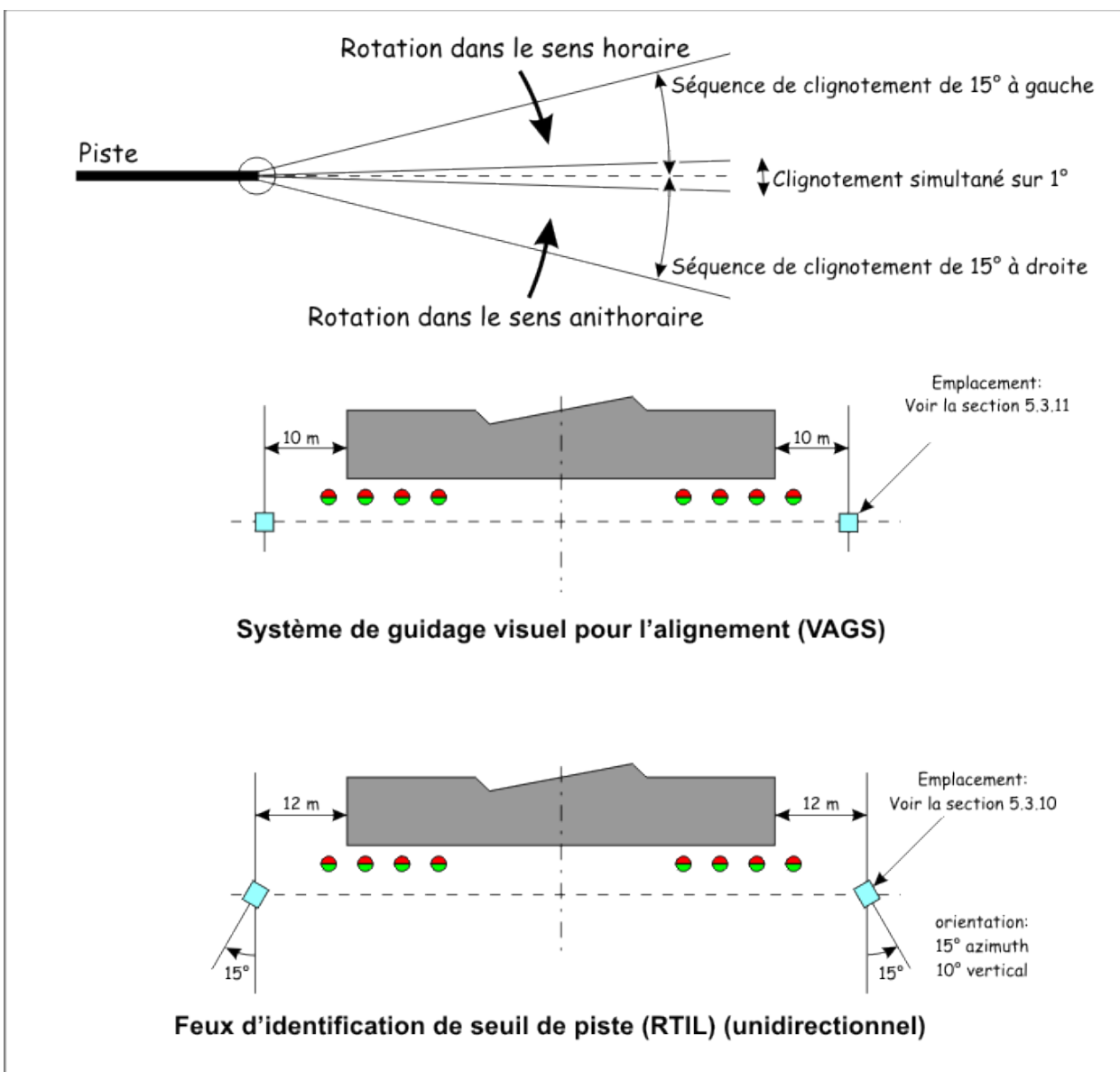
Figure 5-36 : Configuration des VAGS et RTIL
