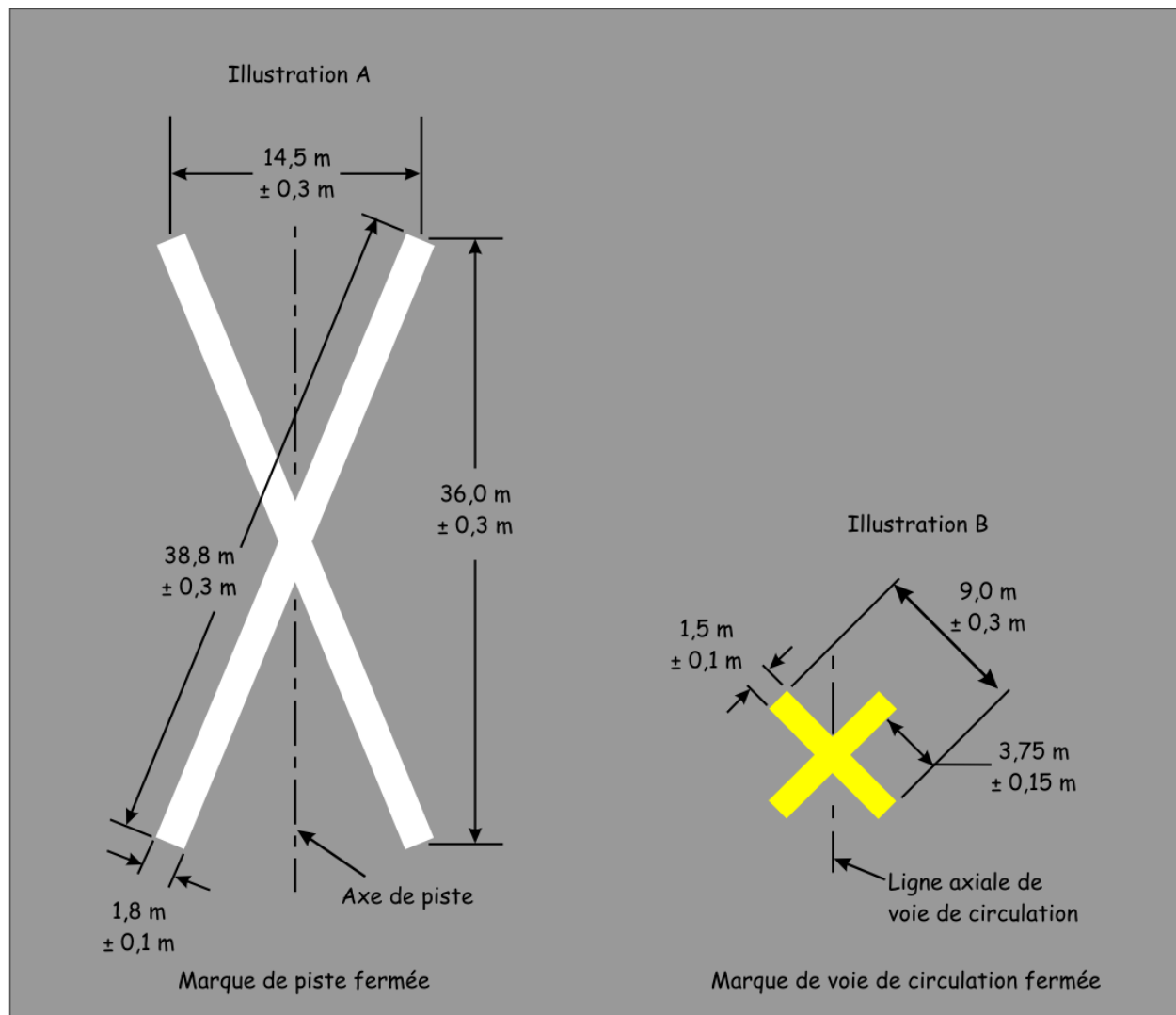
Figure 5-20 : Marques de zone fermée
