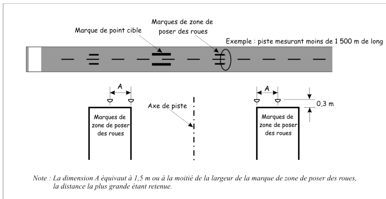
Figure 5-38 : Feux de zone de poser simplifiés
