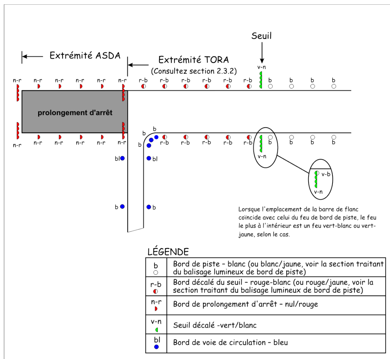
Figure 5-35 : Feux de prolongement d'arrêt (avec décalage)
