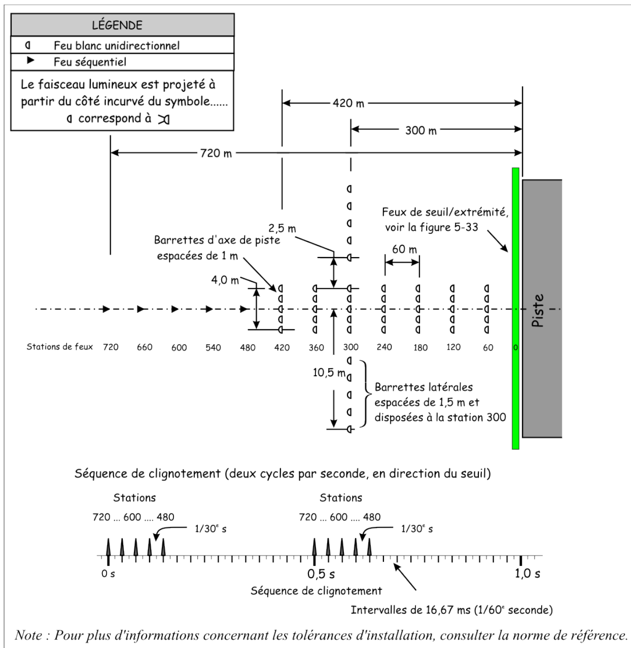
Figure 5-29 : Configuration des dispositifs MALSR/SSALR
