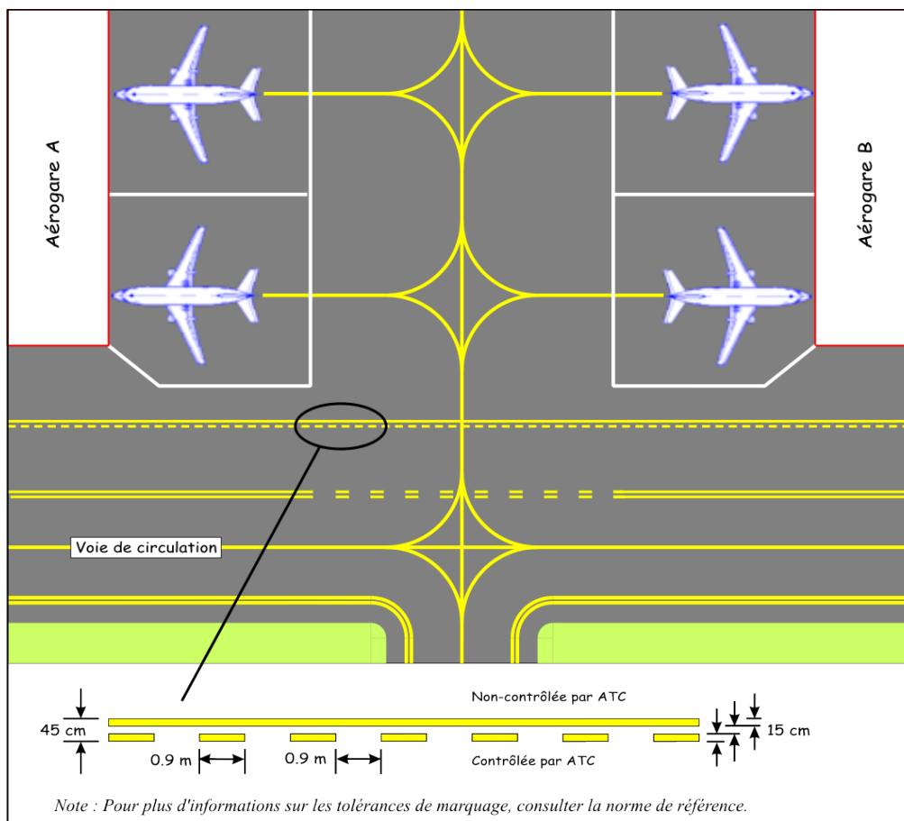
Figure 5-17 : Marques de délimitation de l'aire de manœuvre
