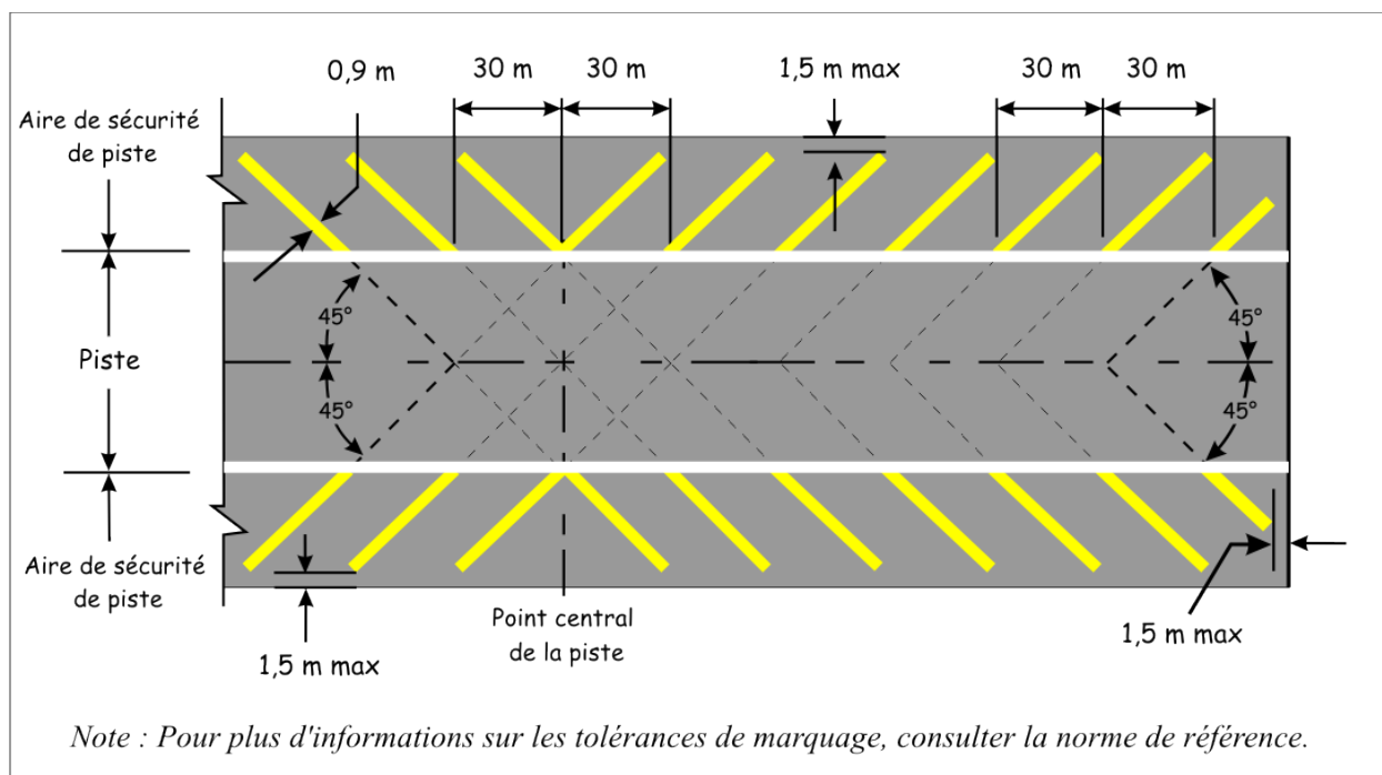
Figure 5-7 : Marques latérales et d'aire de sécurité de piste
