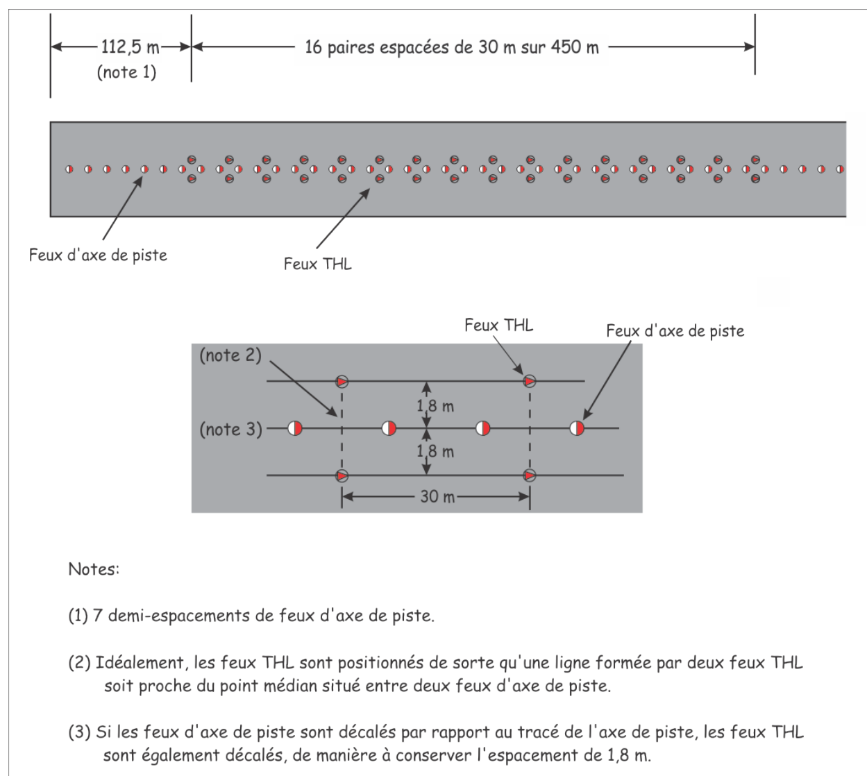
Figure 5-45 : Feux d'état de la piste – Feux d'attente de décollage (THL)
