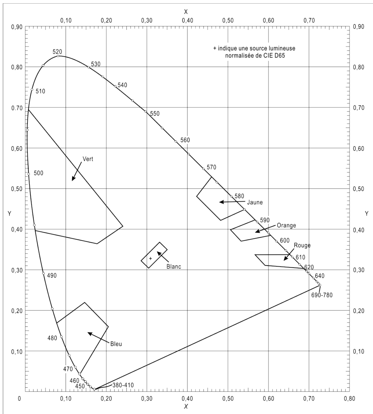
Figure A-3 : Couleurs des matériaux rétro réfléchissants des marques, panneaux et balises
