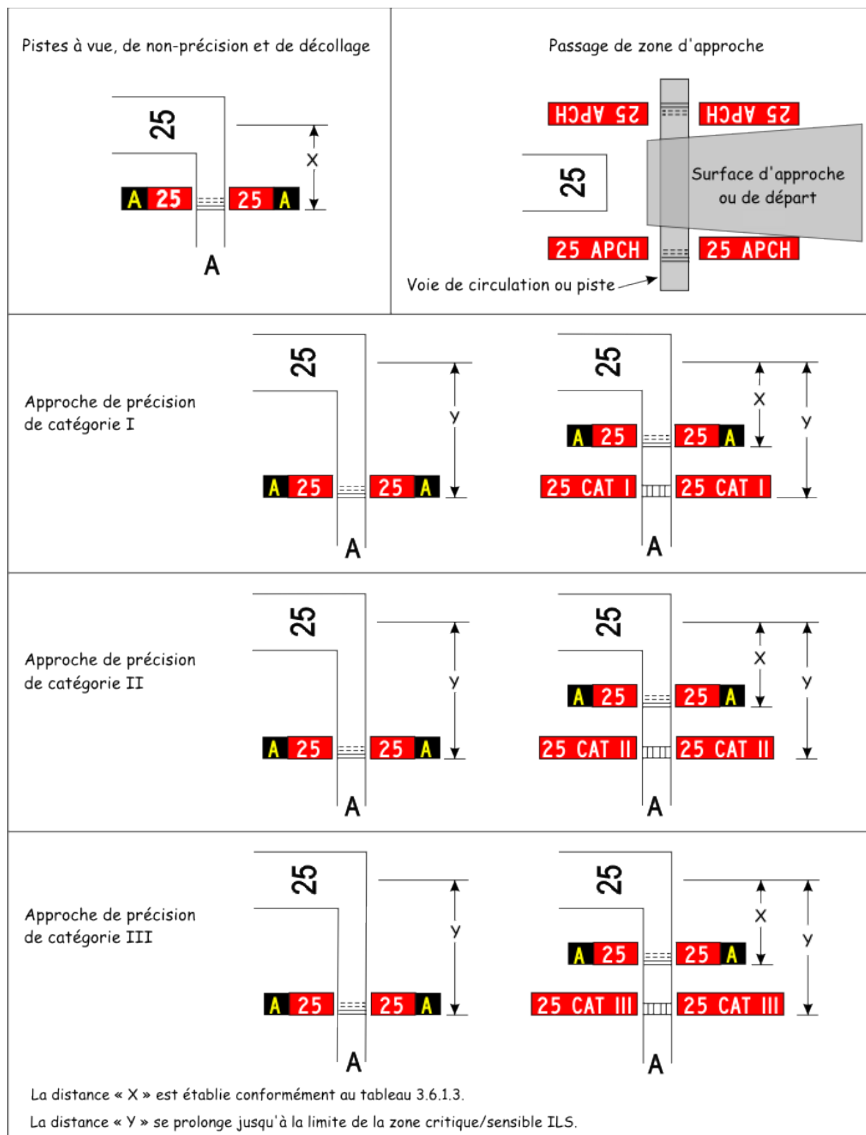
Figure 5-60 : Exemples d'emplacements de panneaux d'instructions obligatoires aux intersections de voie de circulation et de pistes
