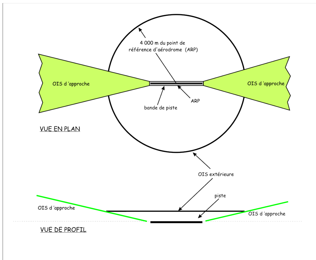
Figure 4-8 : Surfaces d'identification d'obstacles (OIS)
