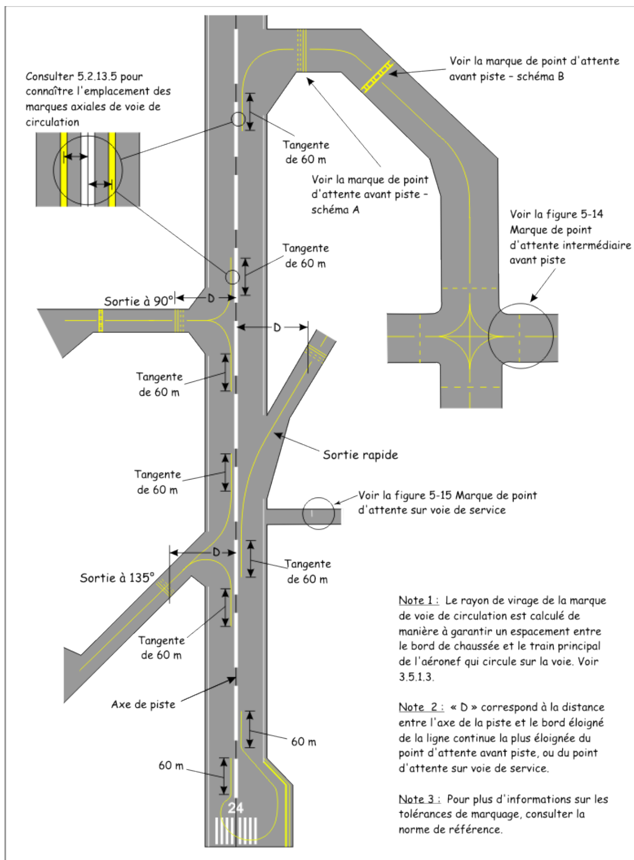
Figure 5-8 : Marques de voie de circulation
