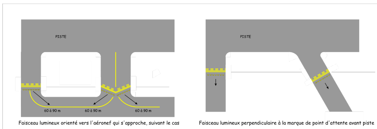
Figure 5-57 : Orientation des feux de protection de piste, Configuration B
