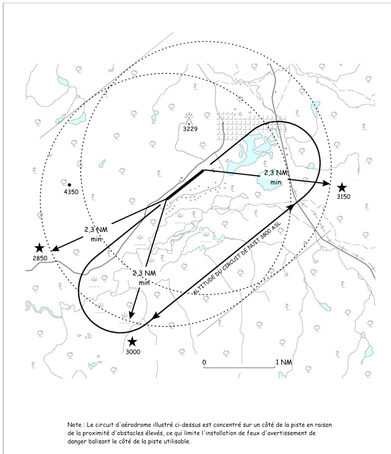
Figure 5-22 : Feux d'avertissement de danger de zone de manœuvre en vol d'un aérodrome
