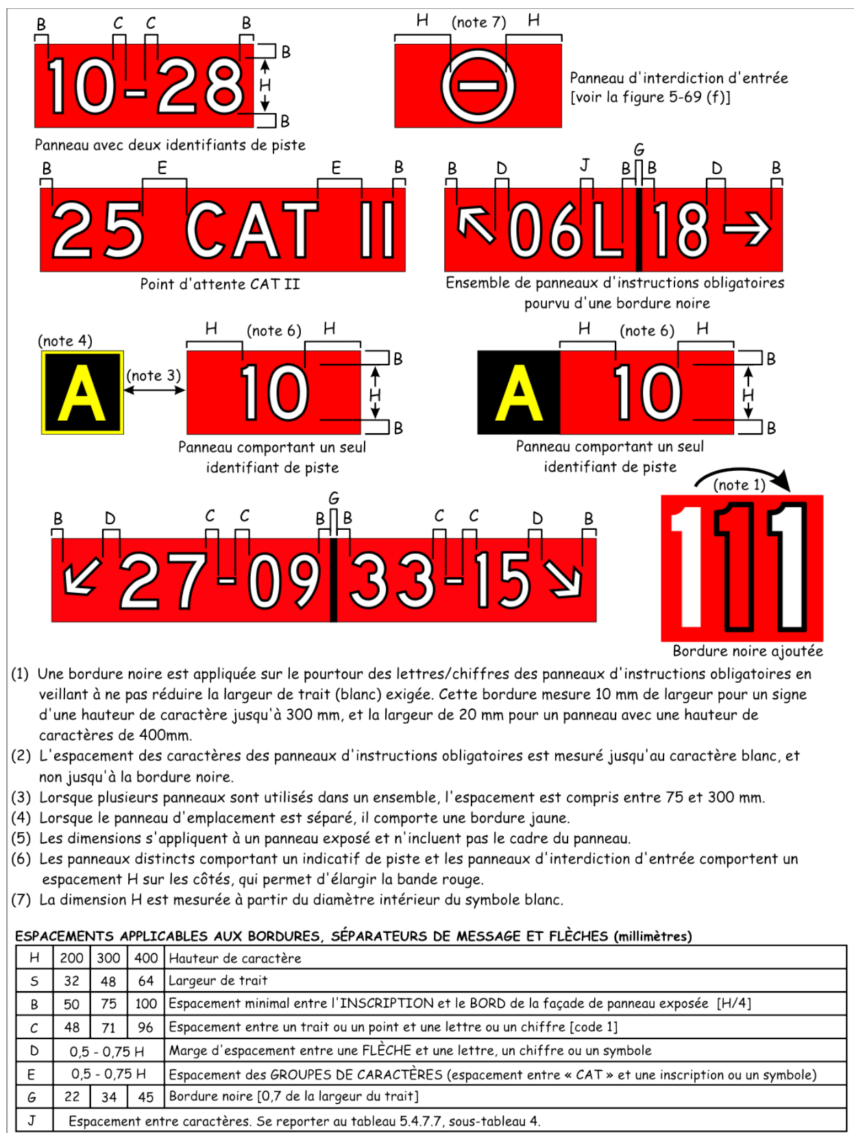
Figure 5-68 (b) : Dimensions des inscriptions
