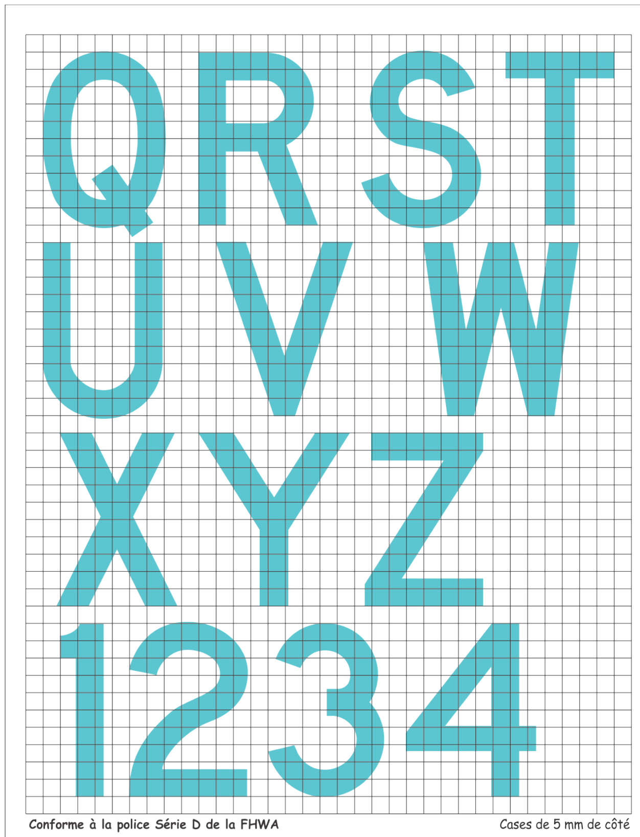
Figure 5-69 (b) : Proportions des caractères
