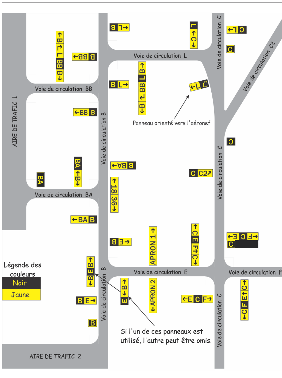
Figure 5-62 : Exemples d'emplacements des panneaux d'indication
