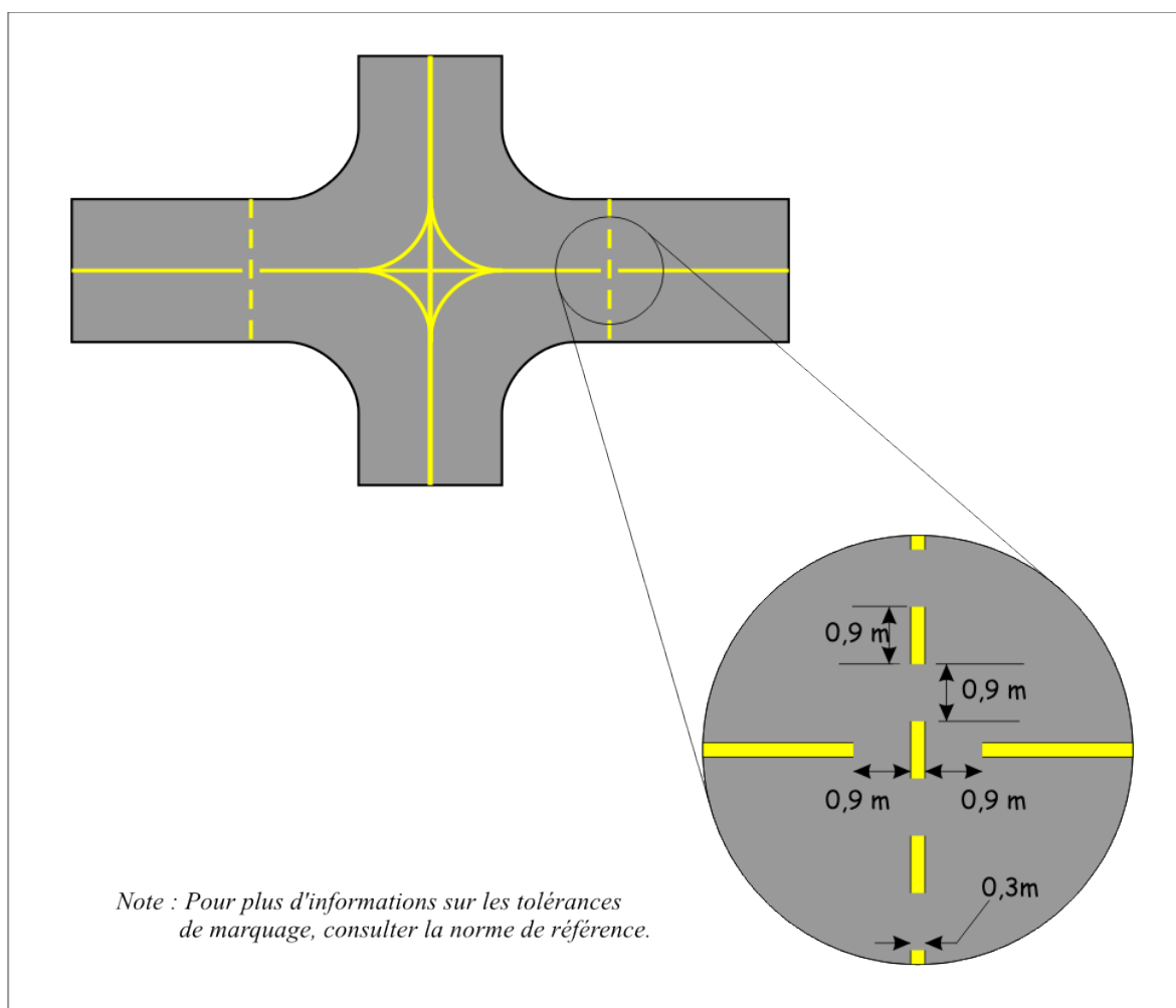
Figure 5-14 : Marques de point d'attente intermédiaire
