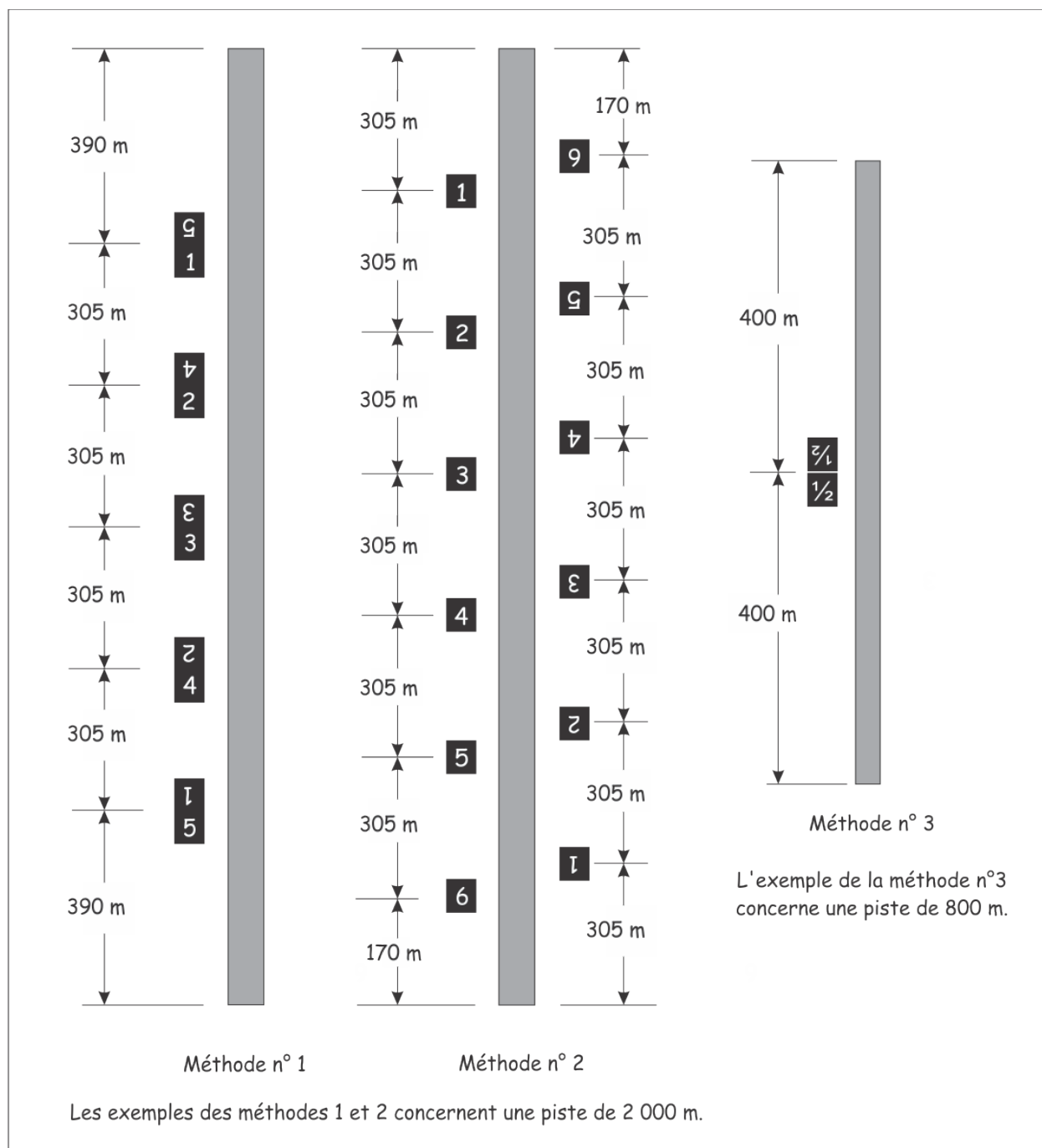
Figure 5-67 : Panneaux de longueur de piste restante
