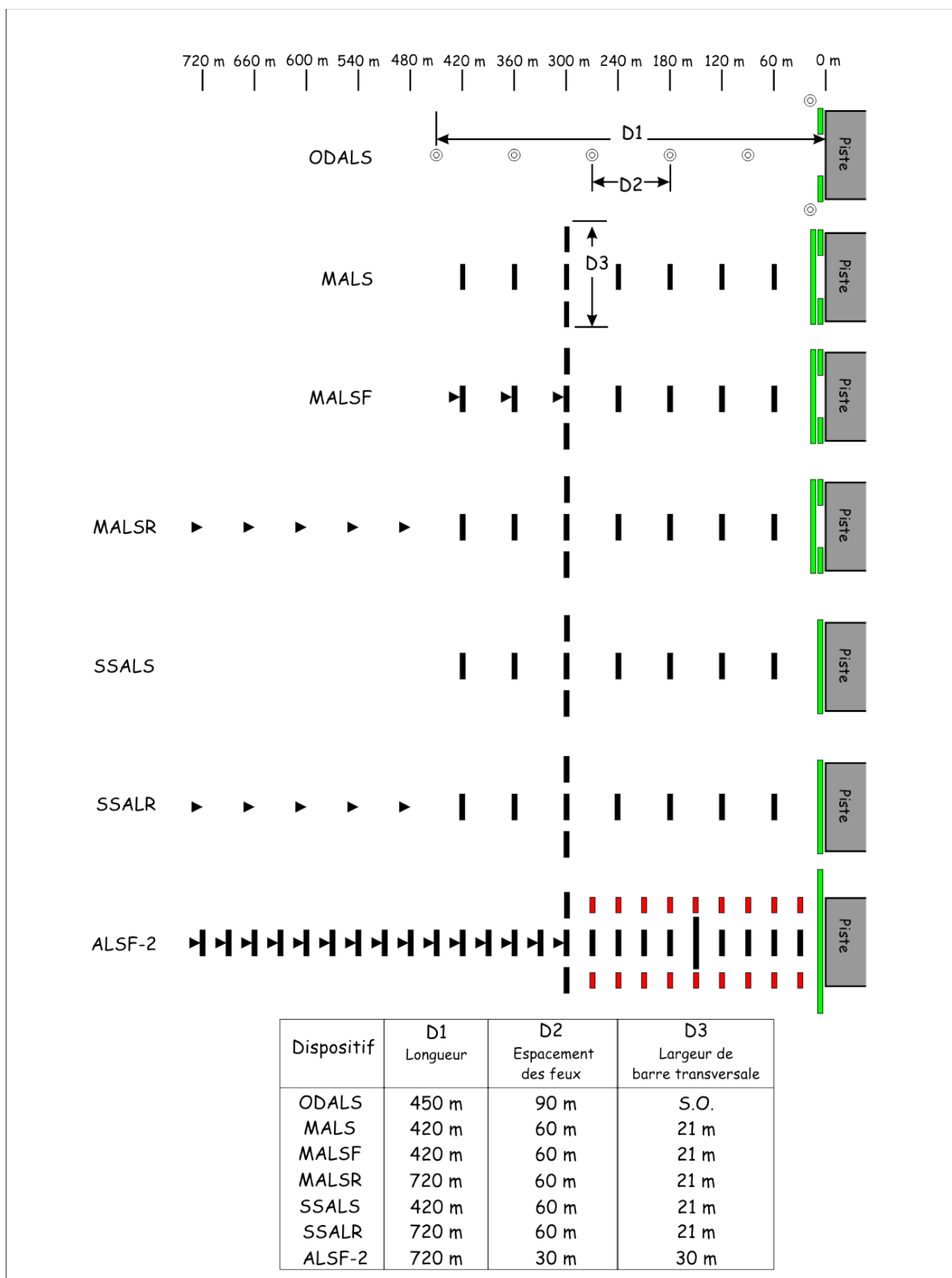
Figure 5-23 : Configuration des dispositifs lumineux d'approche
