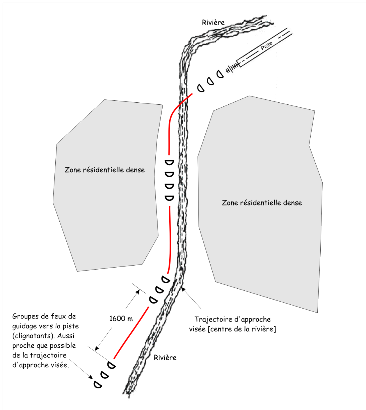
Figure 5-47 : Dispositif lumineux de guidage vers la piste
