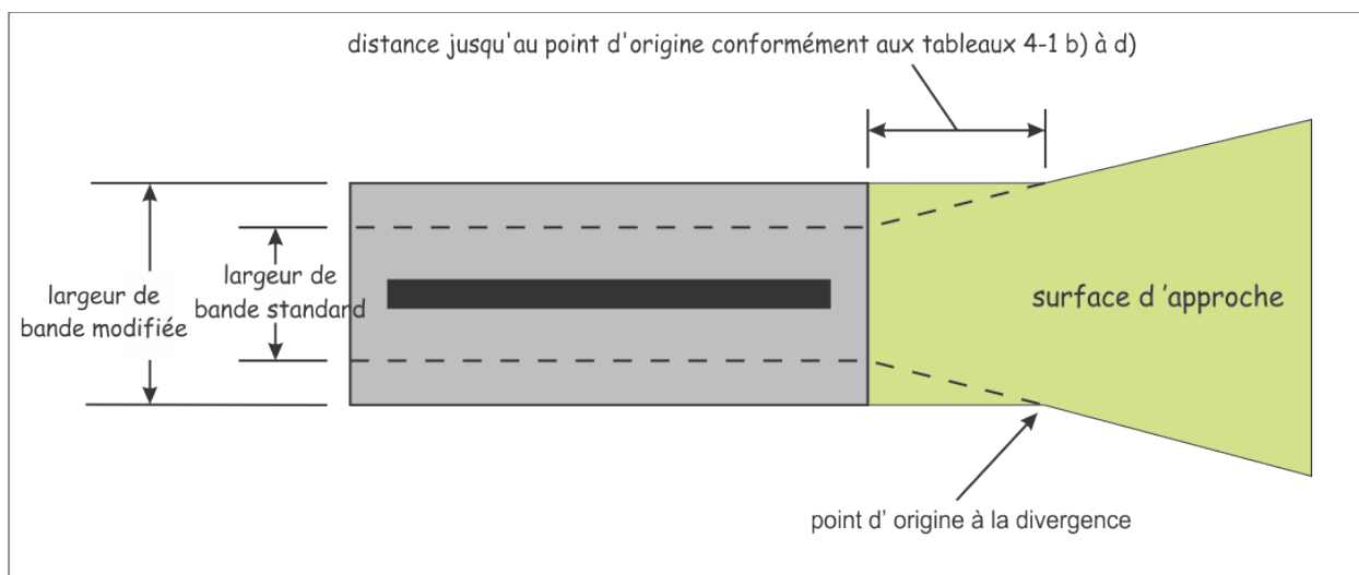
Figure 4-2 (a) : Surface de limitation d'obstacles modifiée
