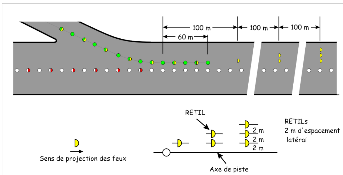
Figure 5-48 : Feux de voie de sortie rapide (RETIL)
