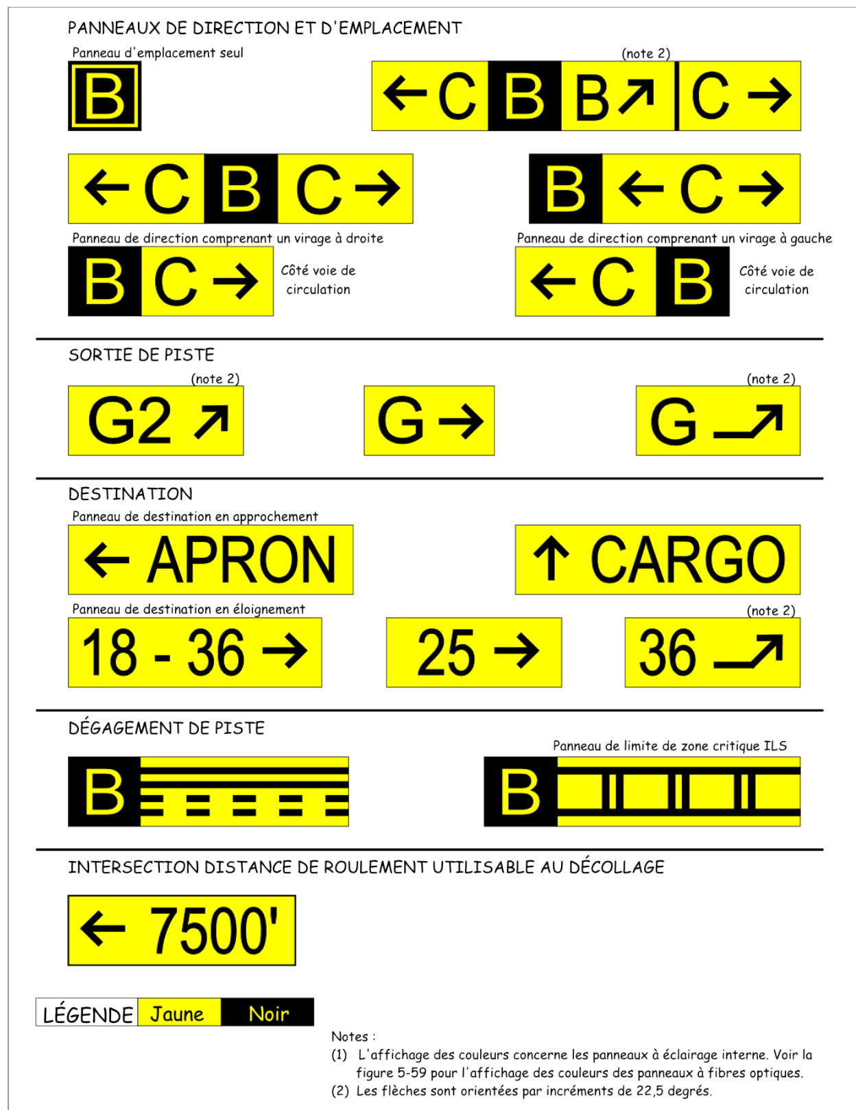
Figure 5-64 : Exemples de panneaux d'indication
