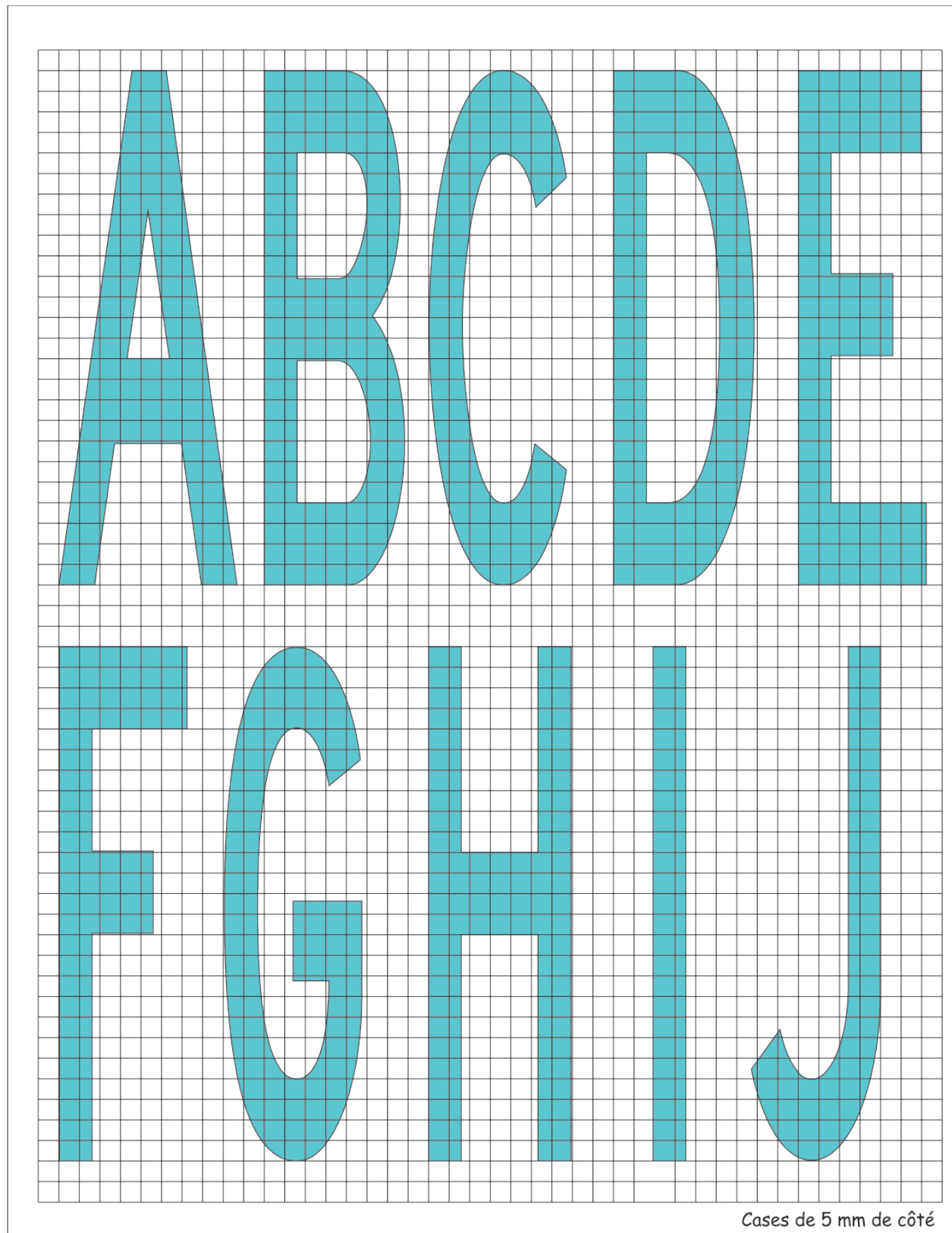
Figure 5-19 (a) : Marques de panneau peint sur la chaussée – Proportions des caractères
