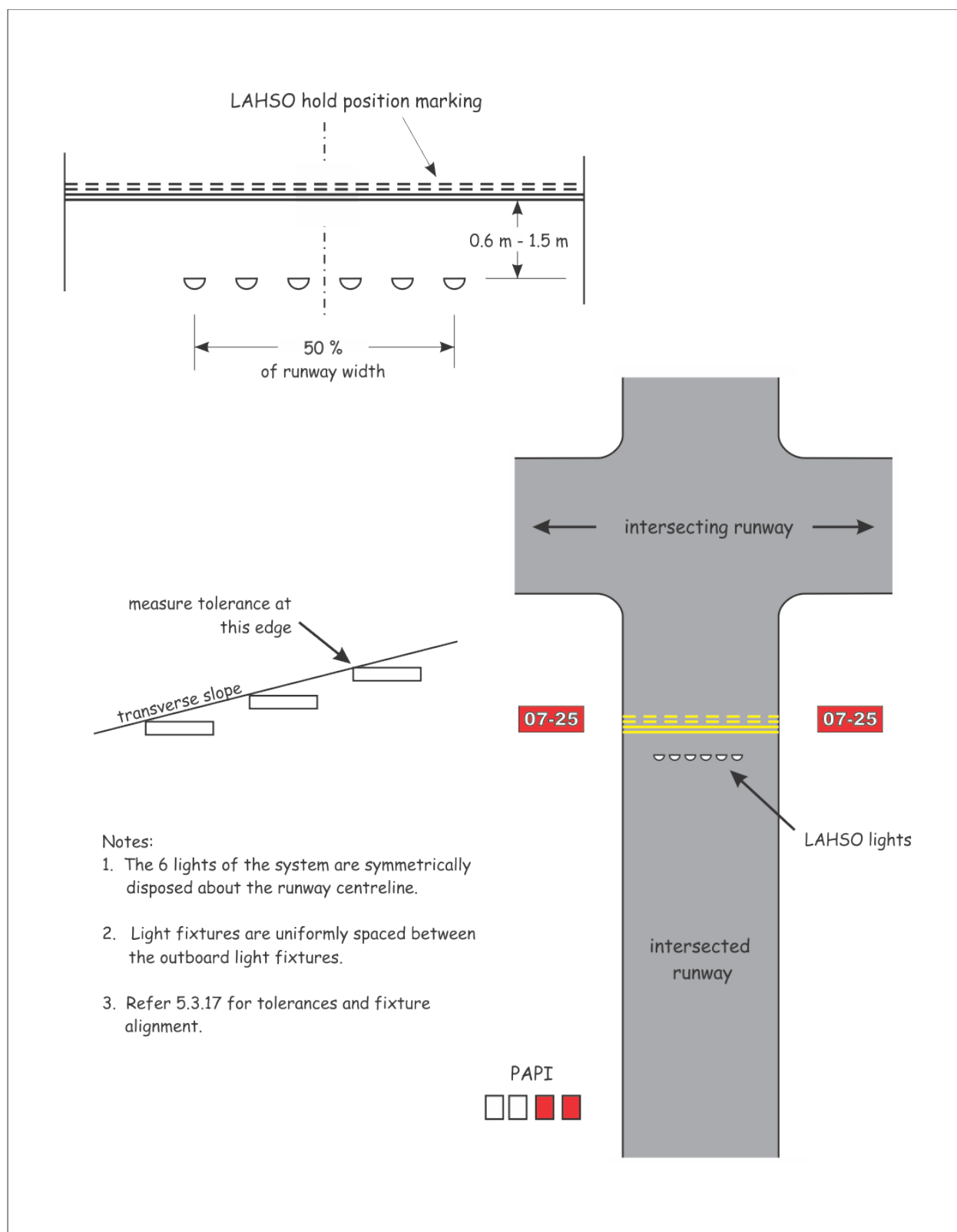
Figure 5-43 : Configuration des aides visuelles LAHSO
