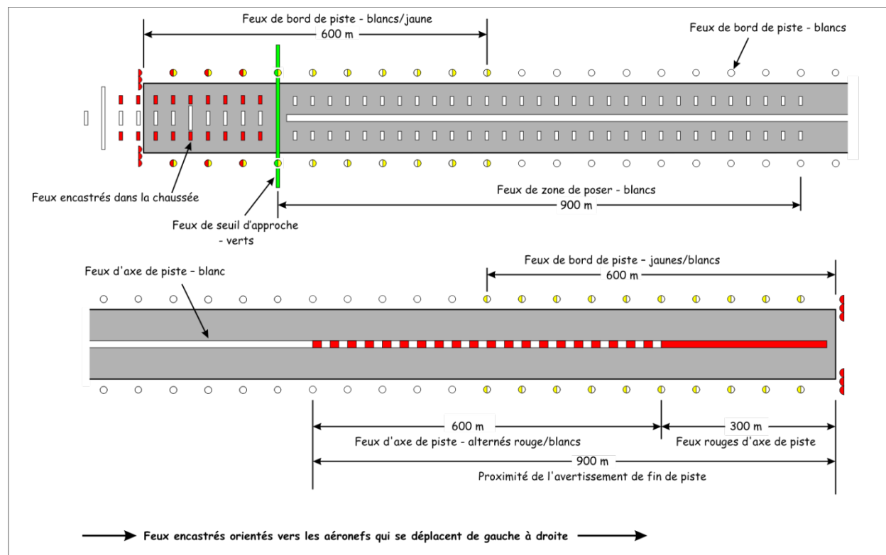
Figure 5-37 : Feux de bord de piste, d'axe de piste et de zone de poser
