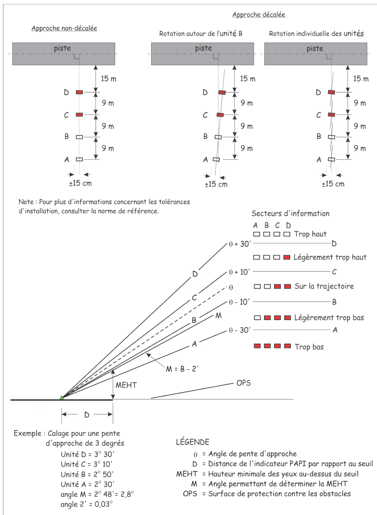
Figure 5-41 : Profil général d'un dispositif PAPI
