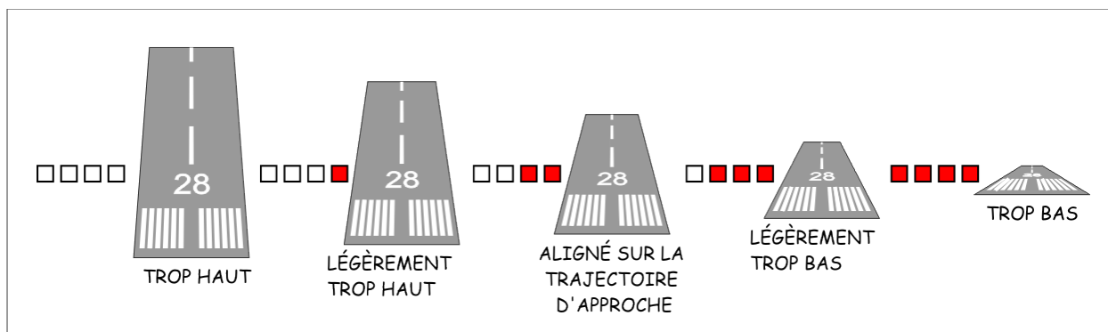
Figure 5-39 : Présentation de la pente d'approche du dispositif PAPI
