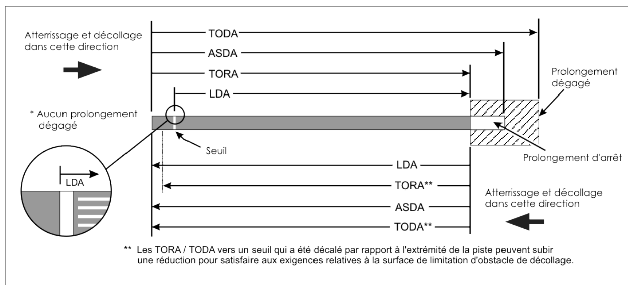
Figure 2-1 : Illustration des distances déclarées
