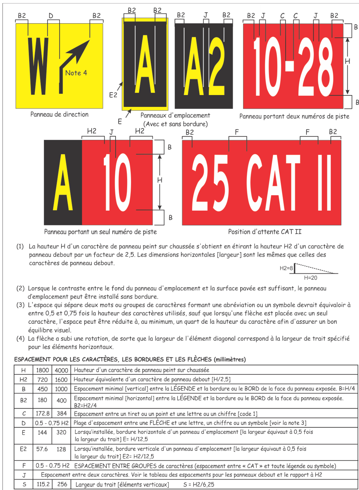
Figure 5-19 (e) : Marques de panneau peint sur la chaussée – Proportions des caractères
