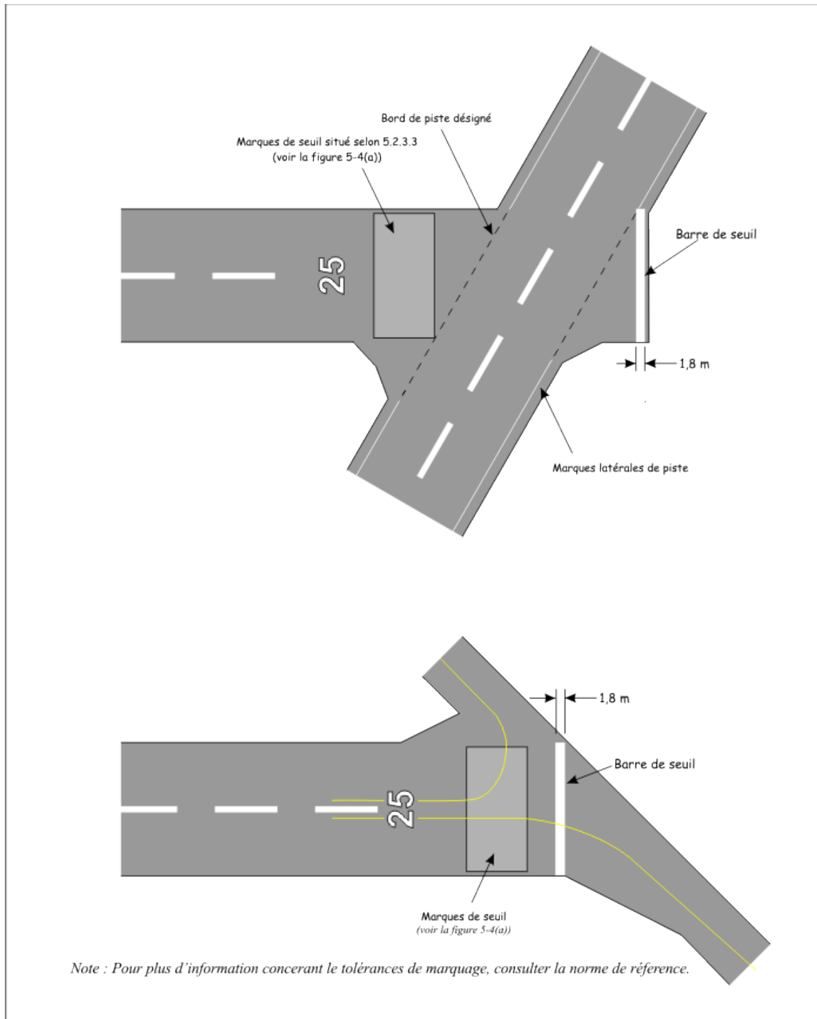
Figure 5-4 (b) : Marques de seuil (avec barre de seuil)
