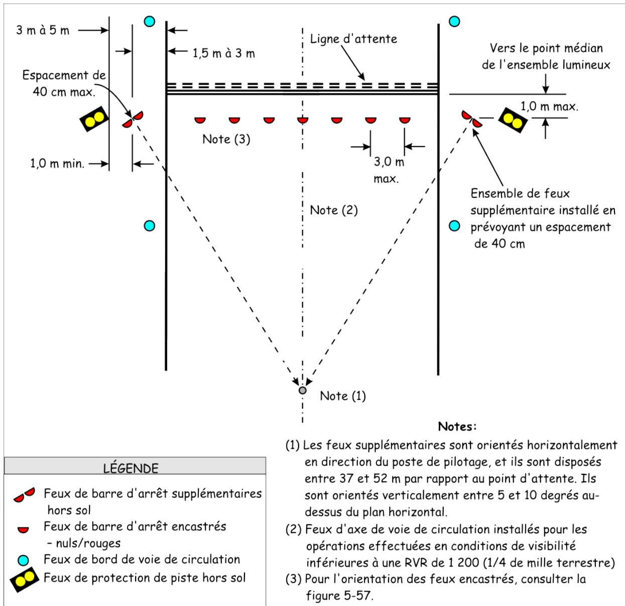
Figure 5-55 : Feux de barre d'arrêt
