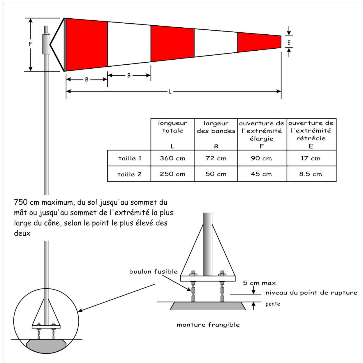
Figure 5-1 : Indicateur de direction du vent standard
