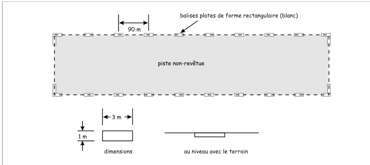
Figure 5-71 (b) : Exemple de balises plates de forme de forme rectangulaire
