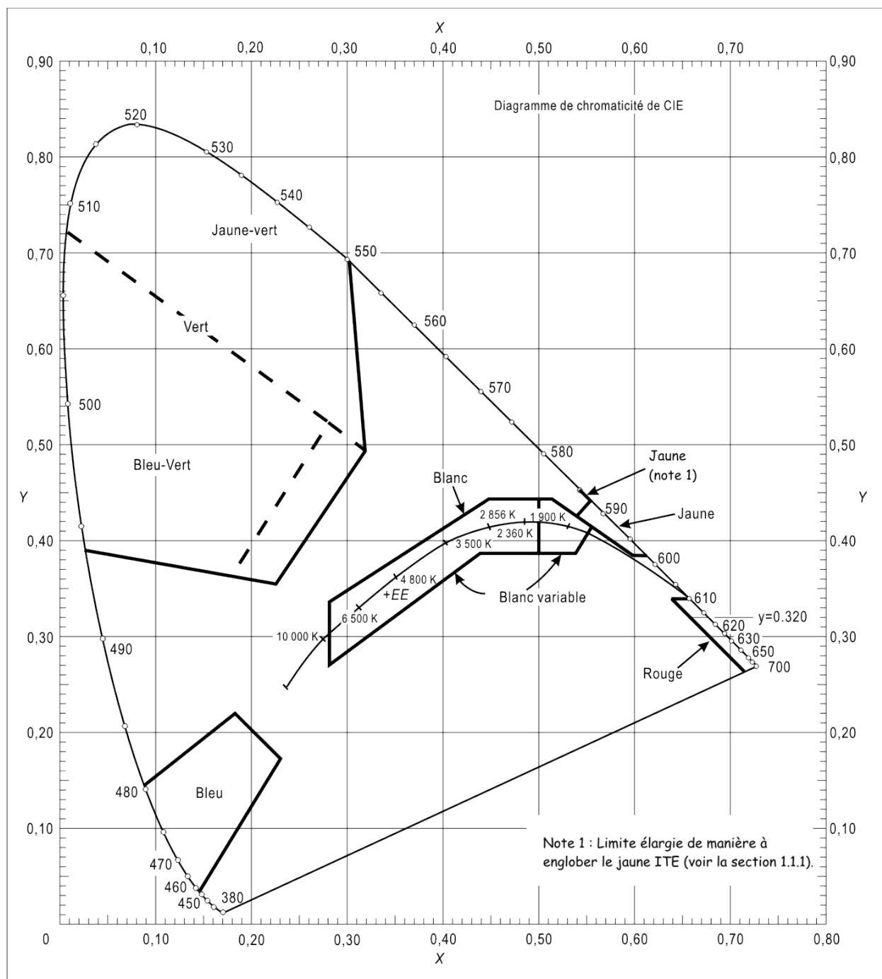
Figure A-1(a) : Couleurs des feux aéronautiques au sol (ampoule à filament)
