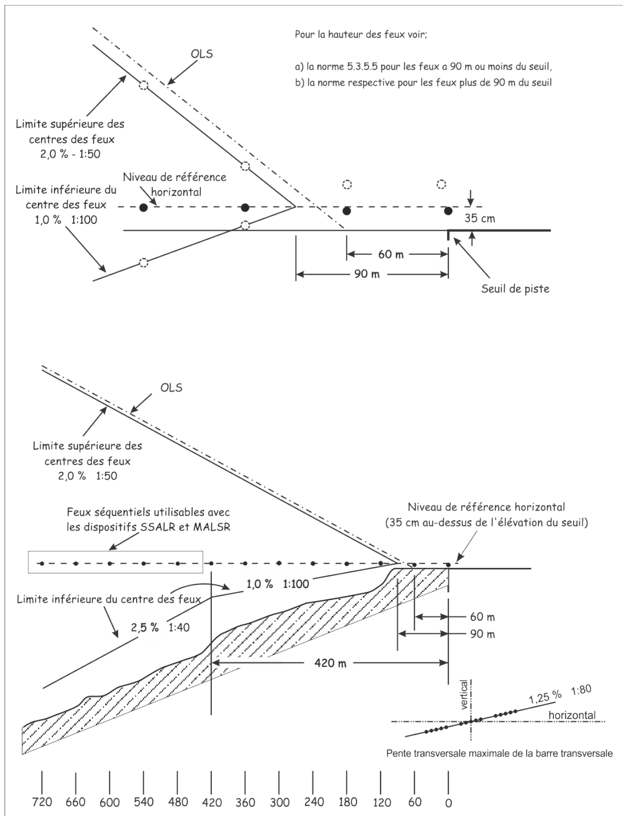
Figure 5-27 : Profil des dispositifs lumineux SSALR/SSALS/MALSR/MALSF/MALS et limites des axes centraux des feux
