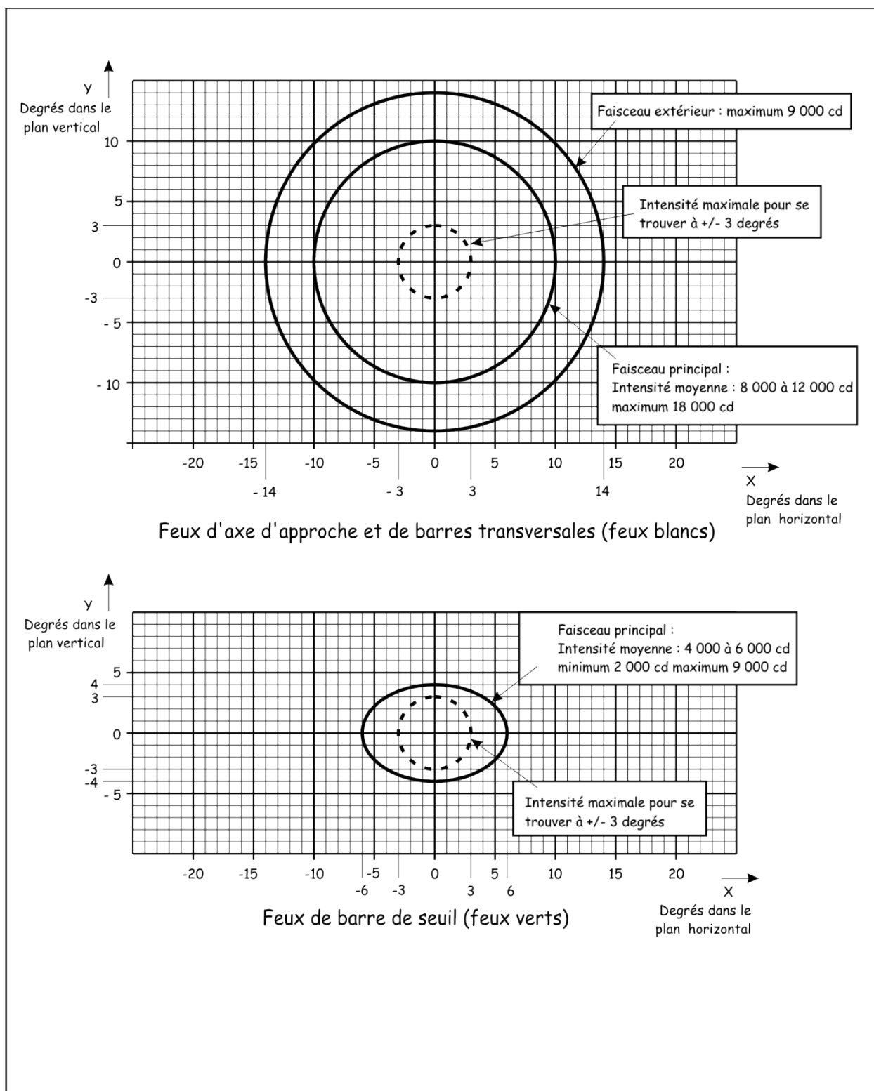
Figure B-22 : Diagramme isocandela des feux d'axe d'approche et de barres transversales (feux blancs) et des feux de seuil (feux verts) hors-sol des dispositifs MALSR, MALSF et MALS
