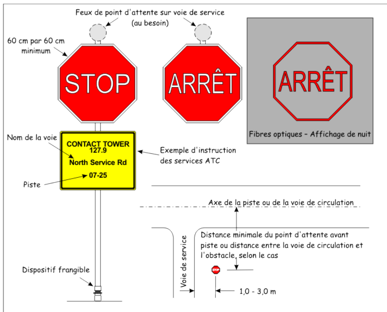
Figure 5-66 : Panneau de point d'attente sur voie de service
