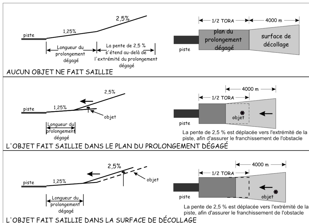
Figure 4-9 : Plan du prolongement dégagé
