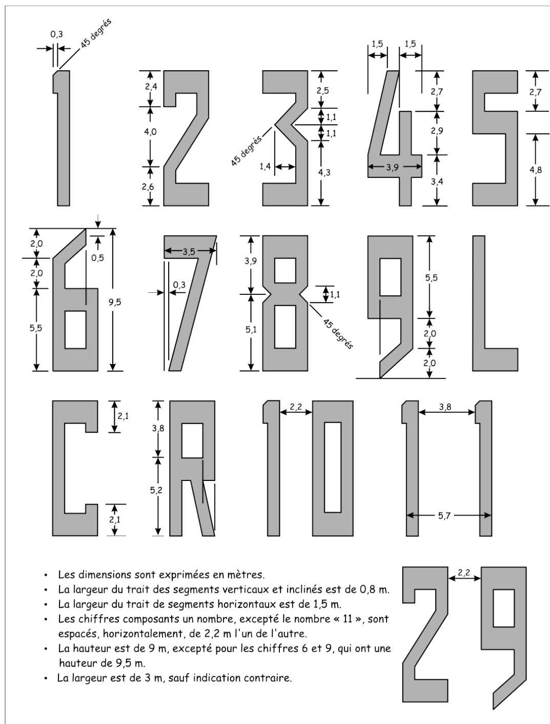
Figure 5-3 : Formes et dimensions des marques d'identification de piste
