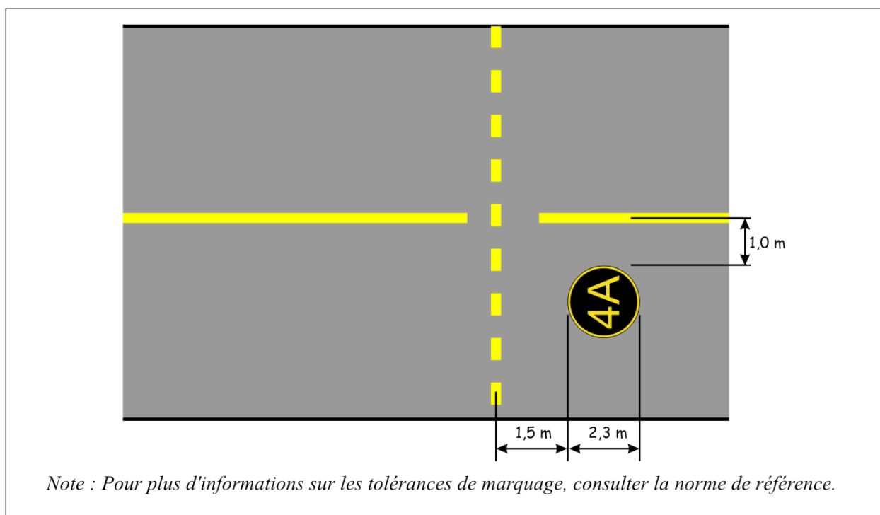
Figure 5-16 : Marques de relevé de position géographique
