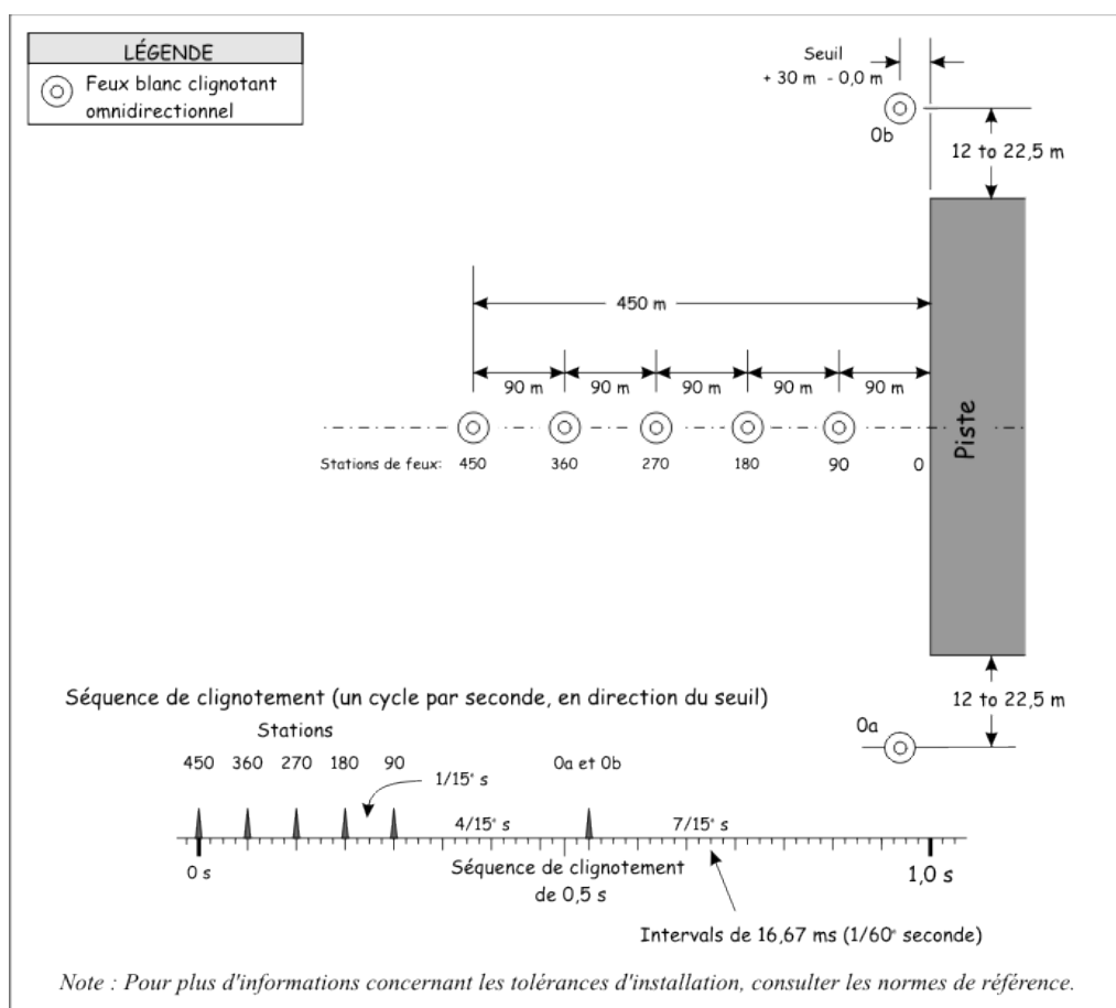
Figure 5-24 : Configuration du dispositif ODALS
