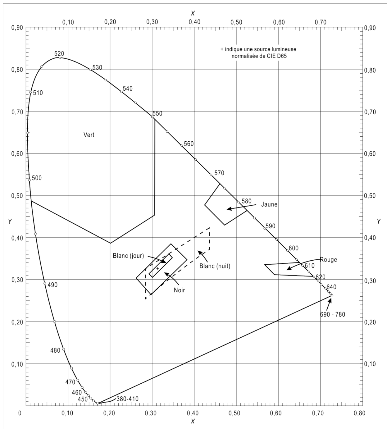
Figure A-4 : Couleurs des panneaux éclairés par transparence (à éclairage interne)
