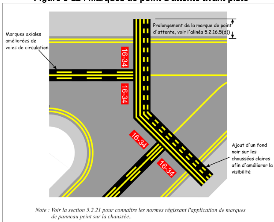
Figure 5-13 : Marques de point d'attente avant piste avec marques axiales améliorées de voie de circulation et prolongement de marque de point d'attente
