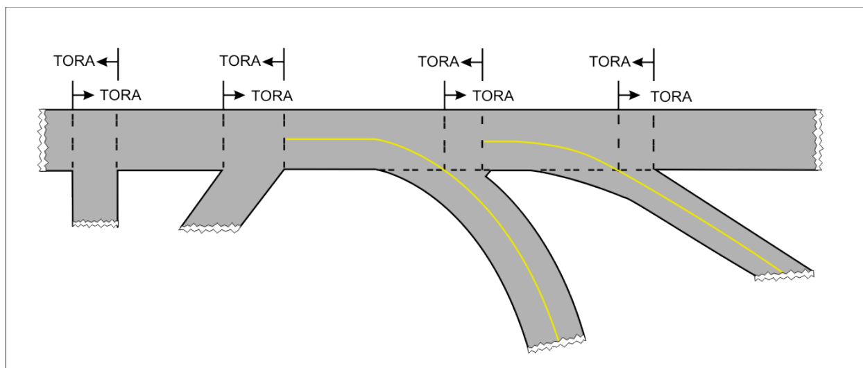
Figure 2-3 : Illustration des distances de roulement au décollage à l'intersection
