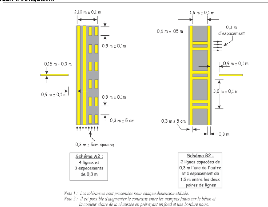
Figure 5-12 : Marques de point d'attente avant piste
