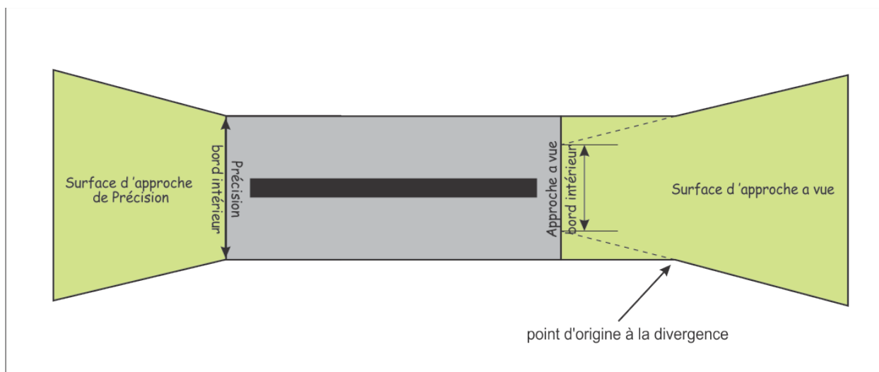
Figure 4-2 (b) Exemple de piste à surface d'approche de précision à une extrémité et à surface d'approche à vue à l'extrémité opposée
