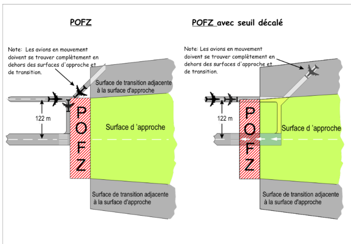
Figure 4-7 : Zone dégagée d'obstacles de précision
