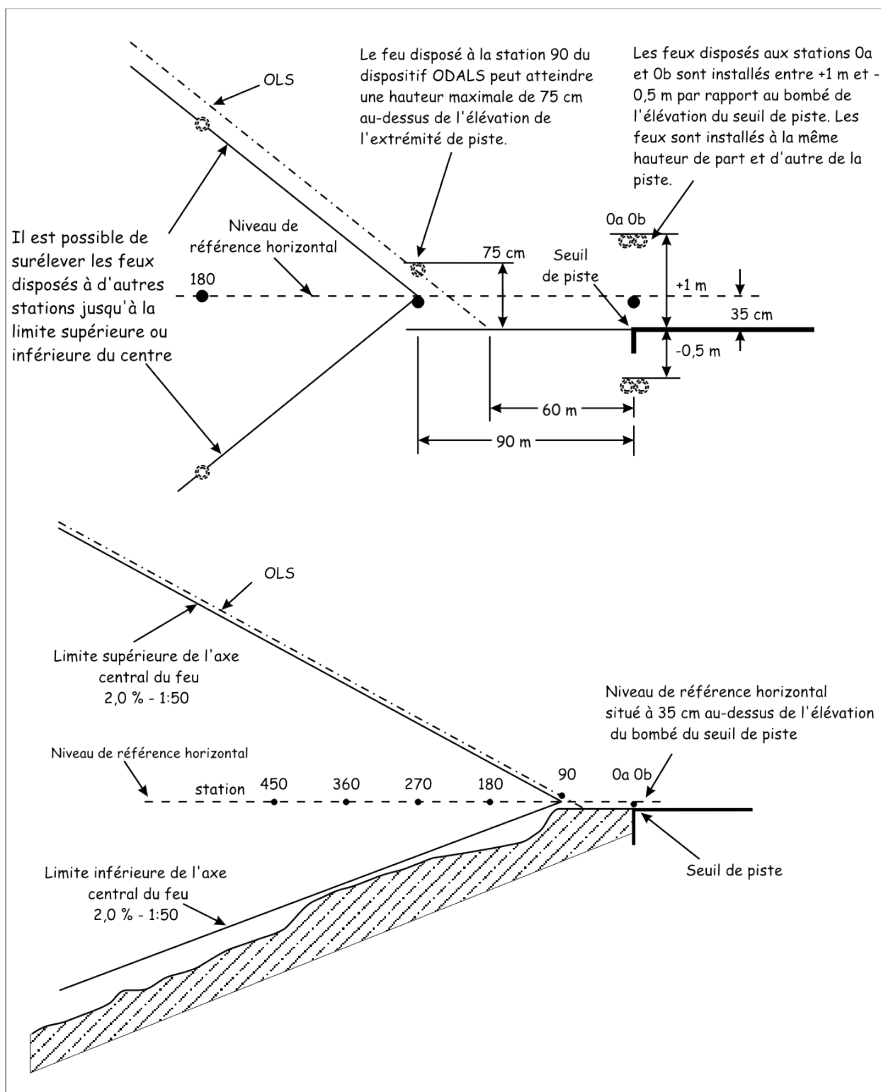
Figure 5-25 : Profil du dispositif ODALS et limites des axes centraux des feux
