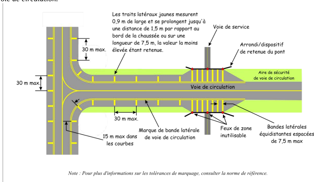
Figure 5-11 : Marques d'aire de sécurité de voie de circulation
