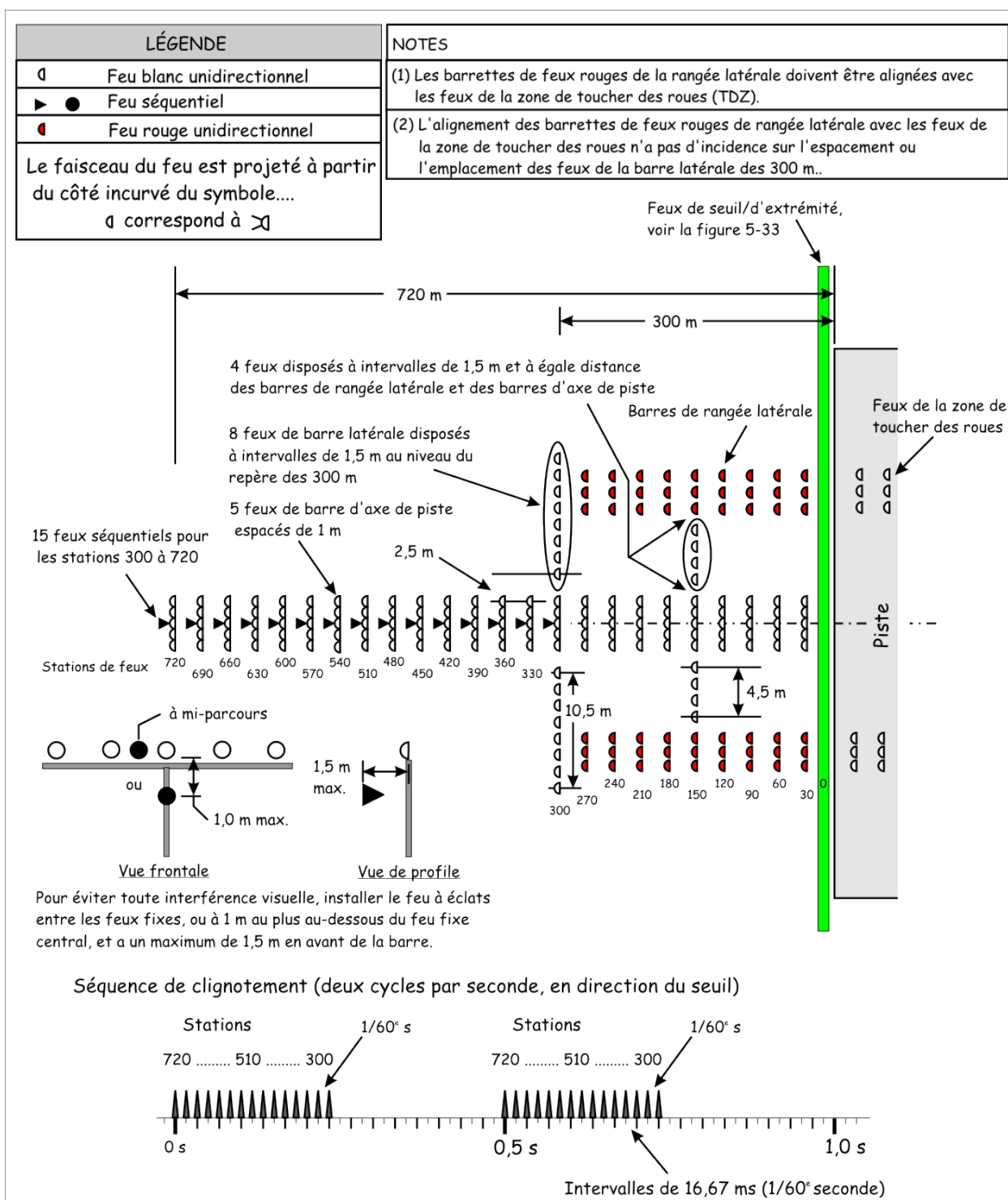
Figure 5-31 : Configuration du dispositif ALSF-2
