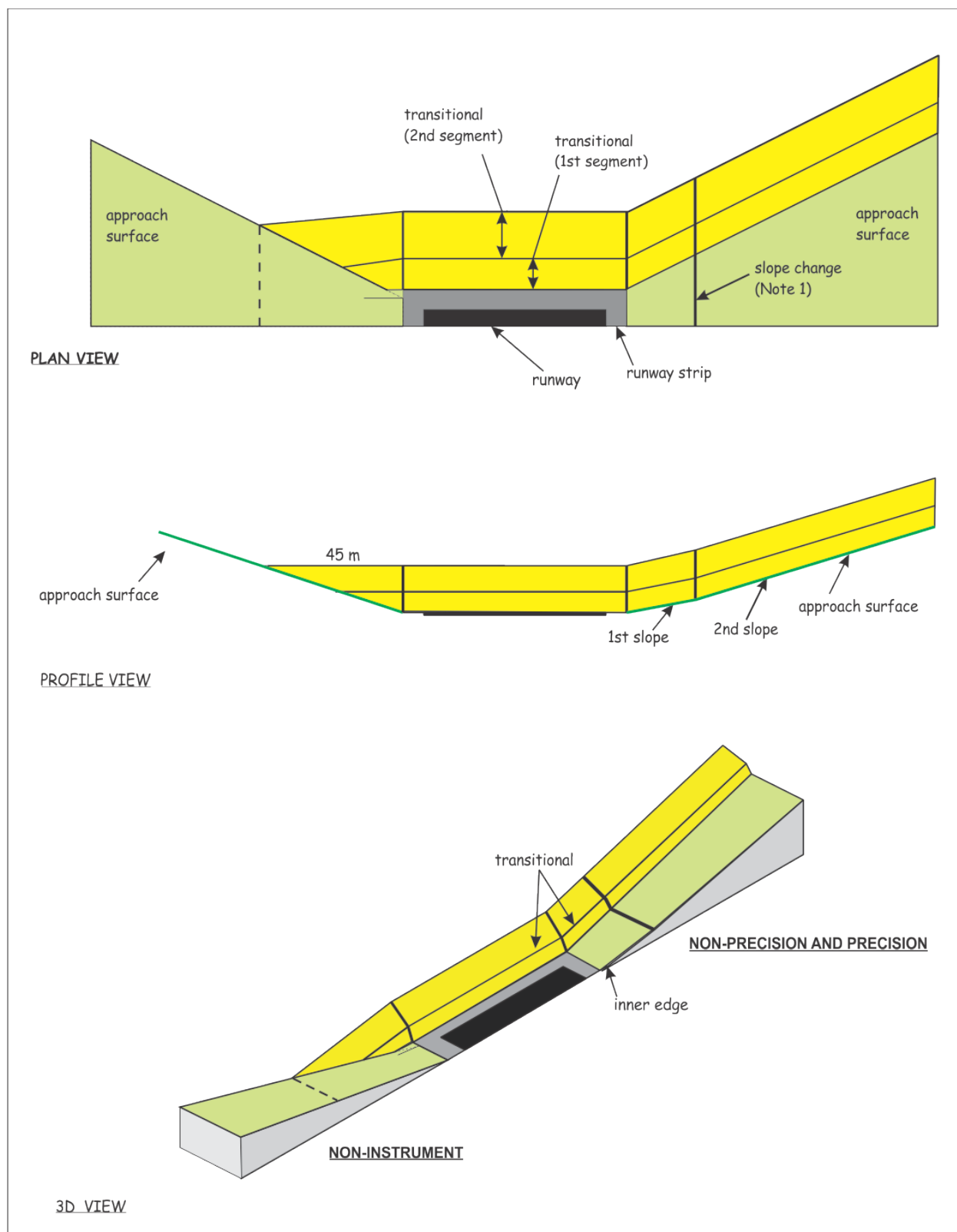
Figure 4-1 (b) : OLS pour une piste aménagée à une extrémité pour les approches de précision/de non-précision et les approches à vue à l'autre extrémité
