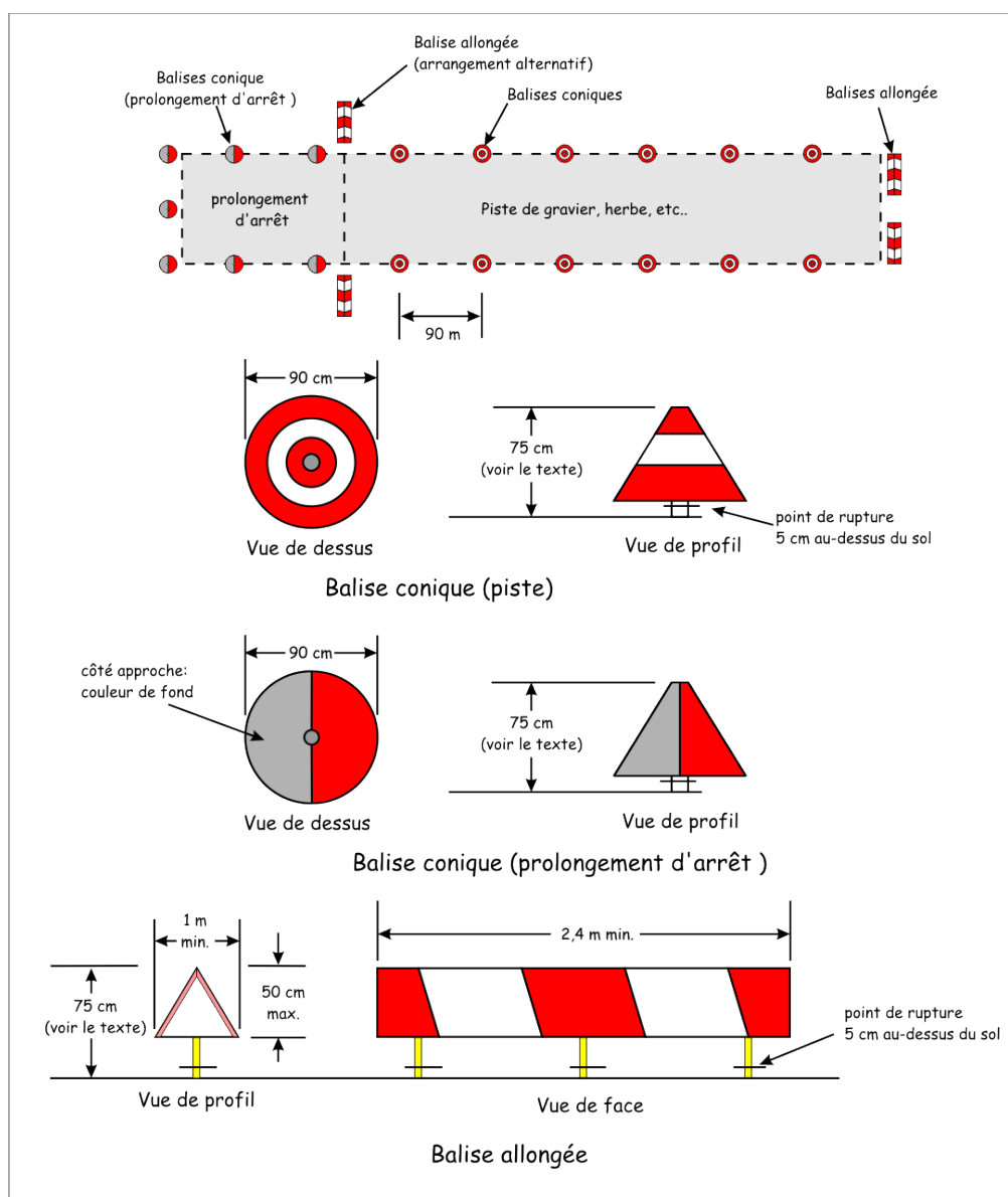
Figure 5-71 (a) : Exemples de balises coniques et pyramidales
