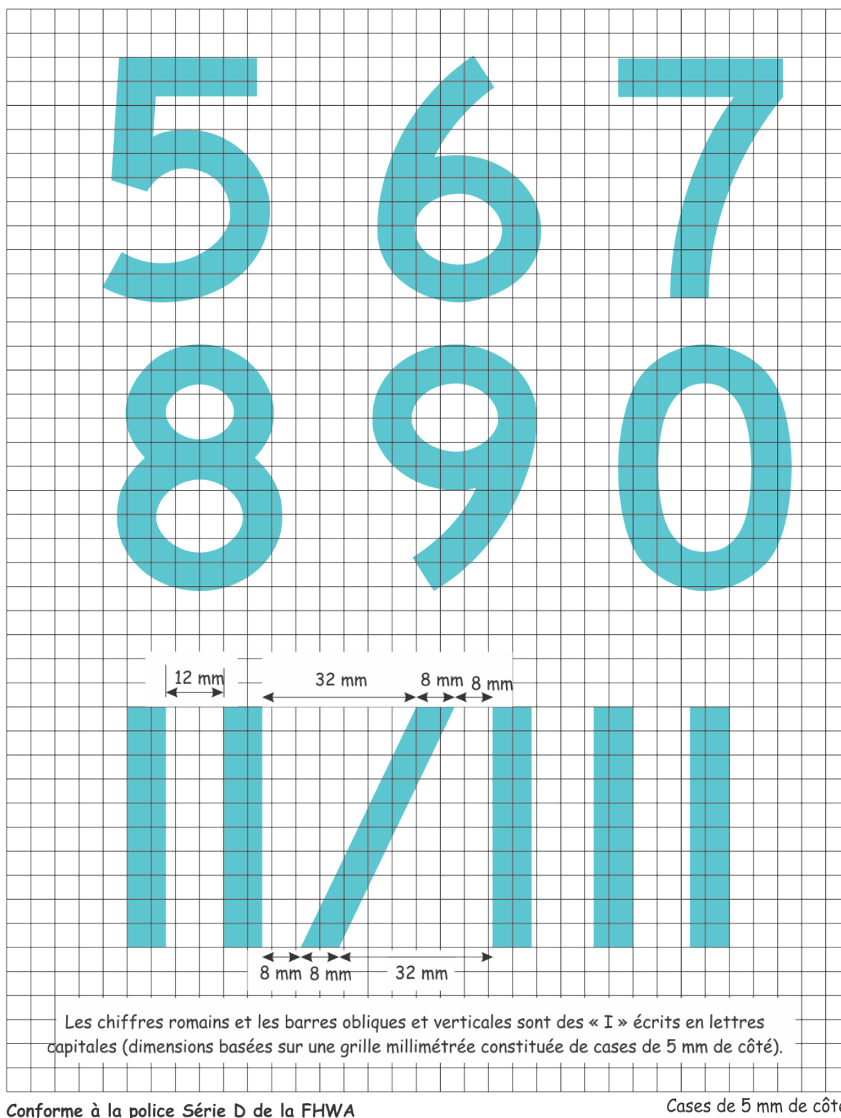
Figure 5-69 (c) : Proportions des caractères
