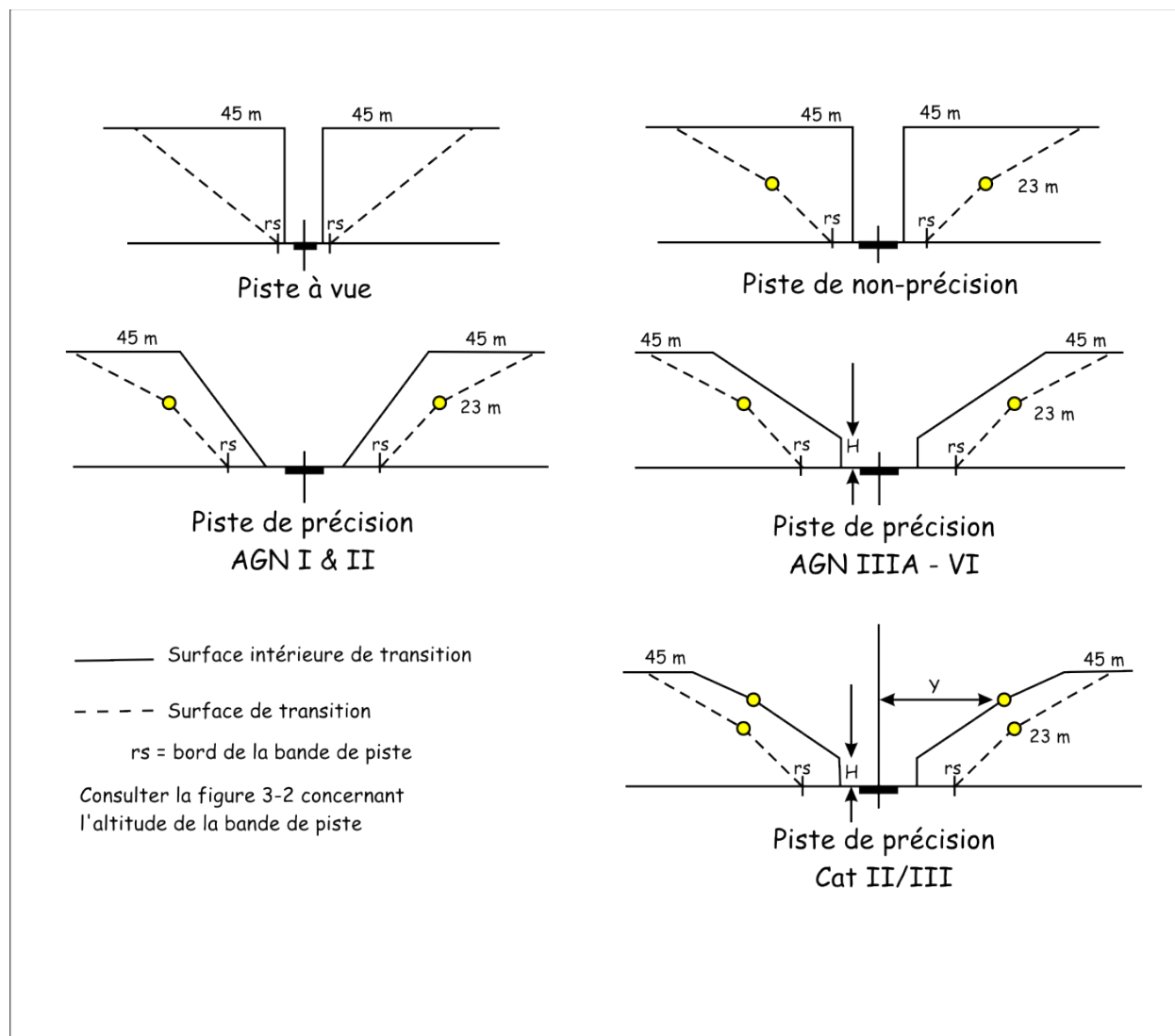
Figure 4-5 : Surface de transition et surface intérieure de transition
