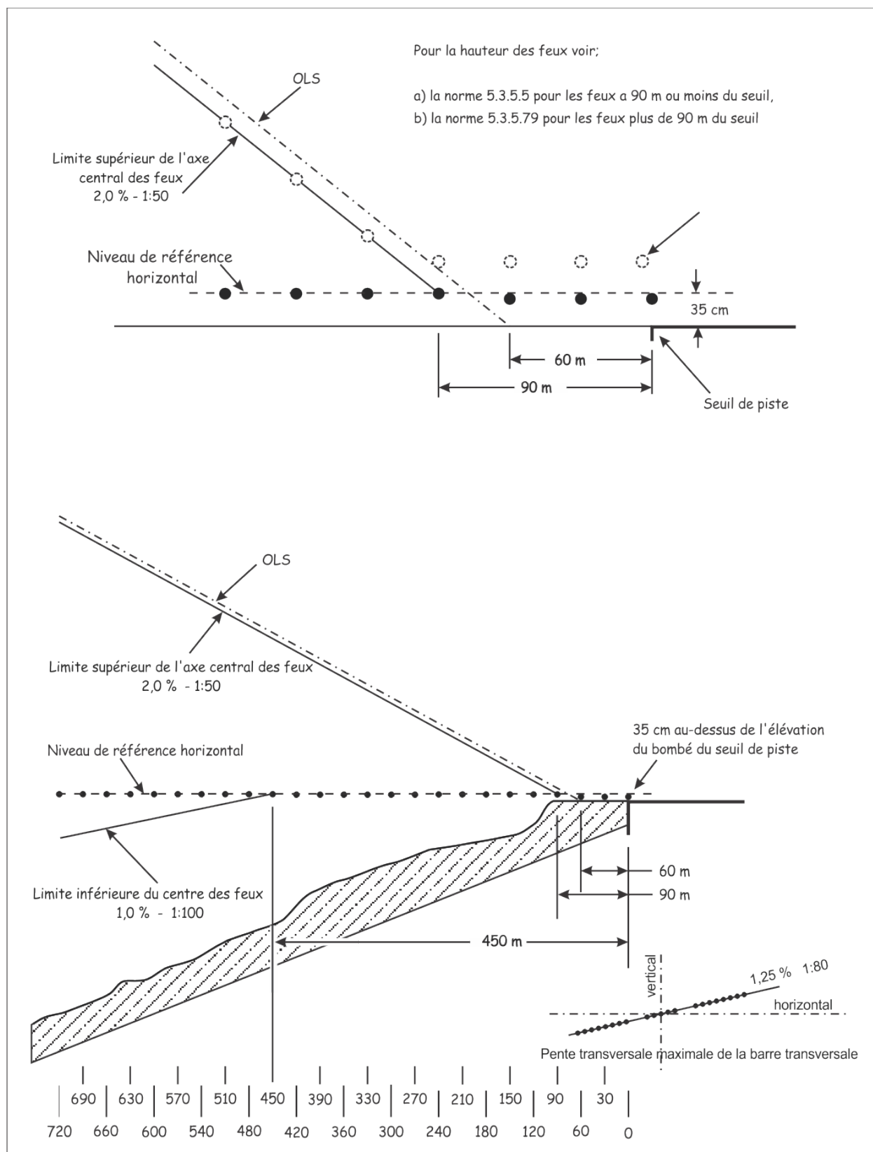
Figure 5-32 : Profil du dispositif ALSF-2 et limites des axes centraux des feux
