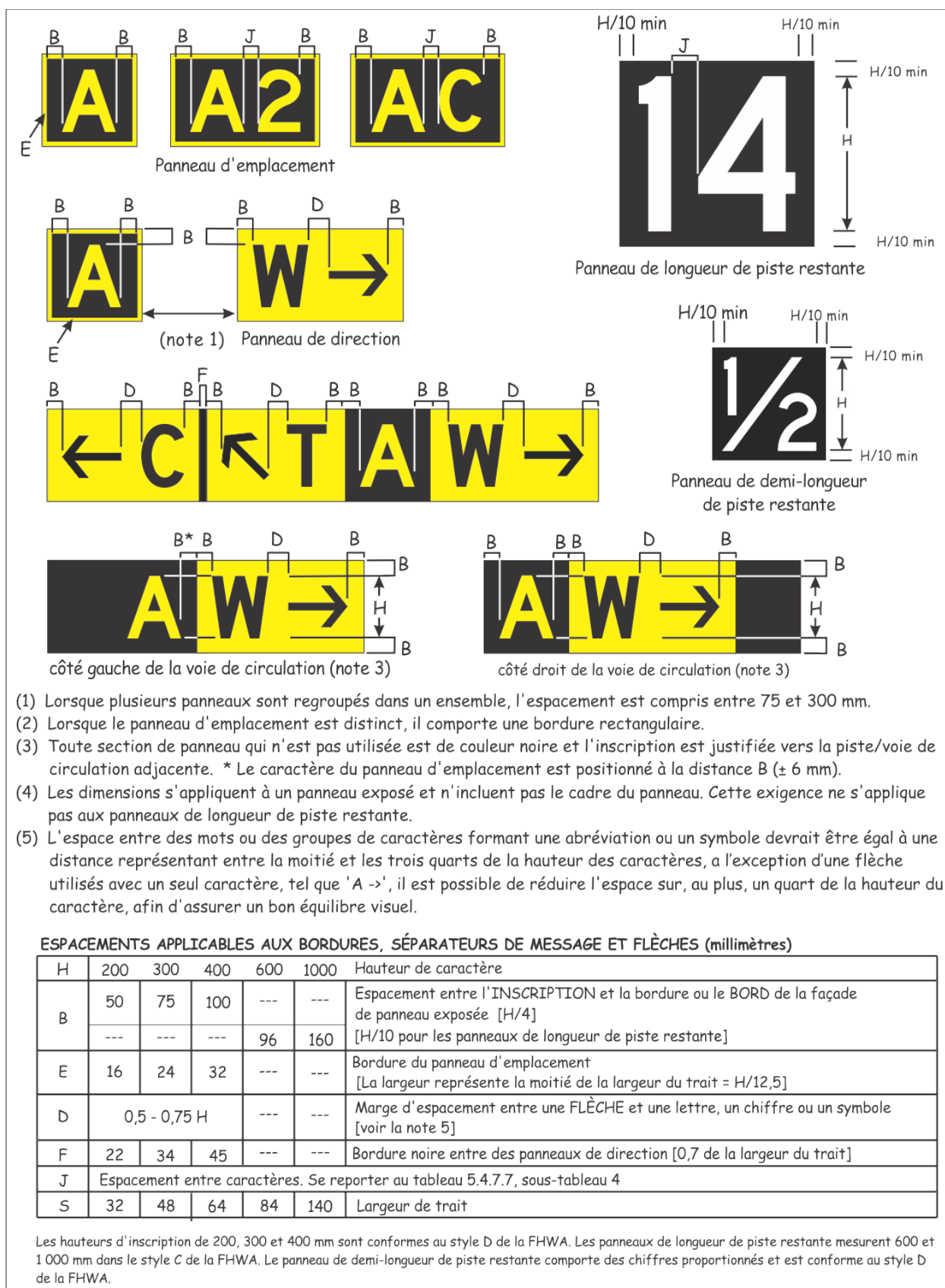
Figure 5-68 (a) : Dimensions des inscriptions
