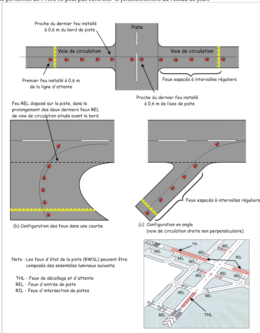
Figure 5-44 : Feux d'état de la piste – Feux d'entrée de piste (REL)
