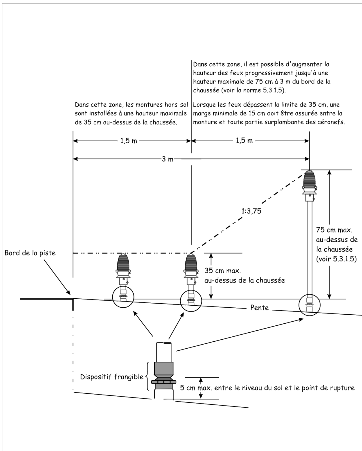
Figure 5-21 : Hauteur de montage des feux hors-sol
