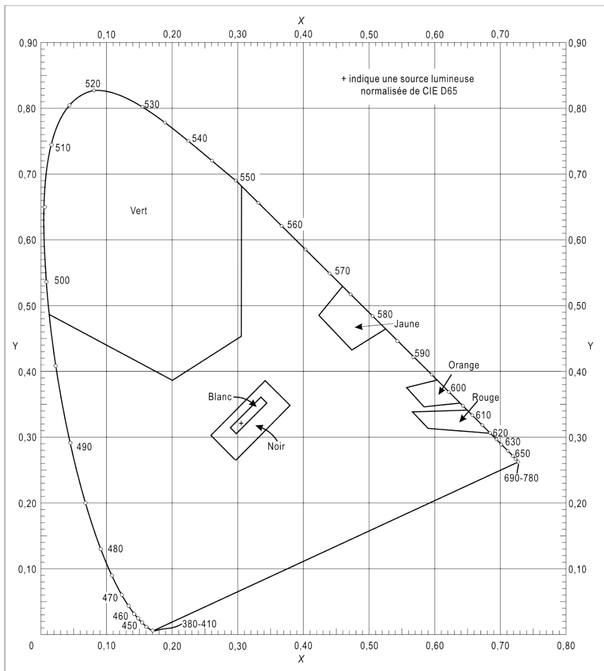
Figure A-2 : Couleurs ordinaires des marques, des panneaux à éclairage externe et des balises non réfléchissantes
