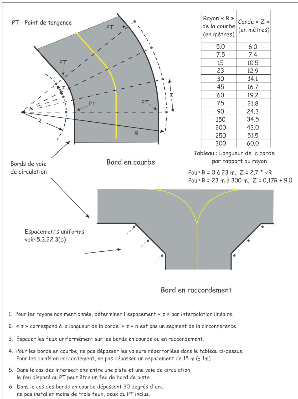
Figure 5-53 : Espacement des feux sur des bords de voie de circulation en courbe
