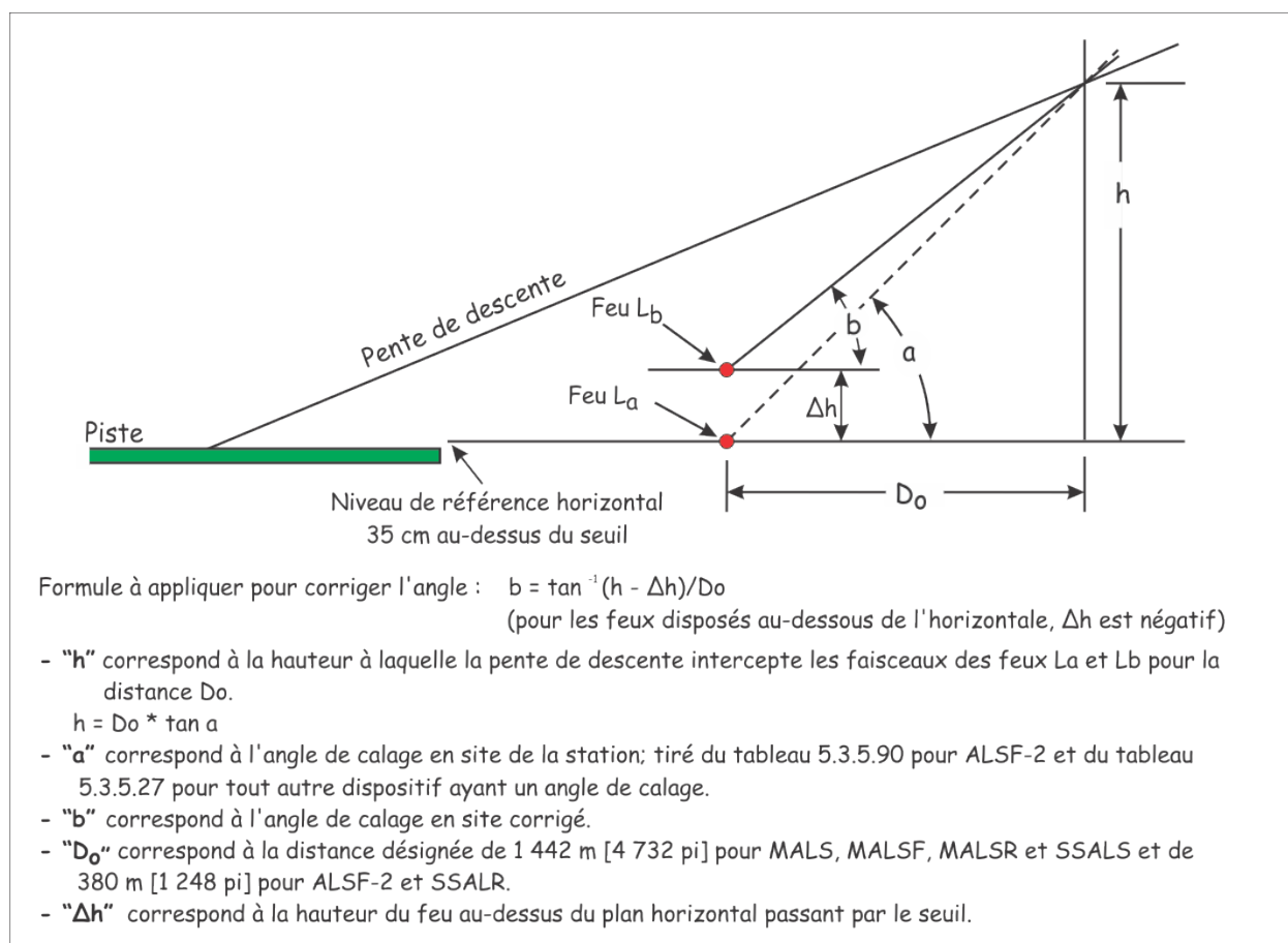
Figure 5-28 : Correction de l'angle de calage en site
