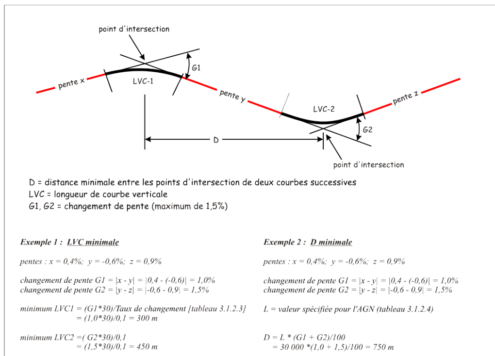
Figure 3-1 : Limites de pente longitudinale de piste
