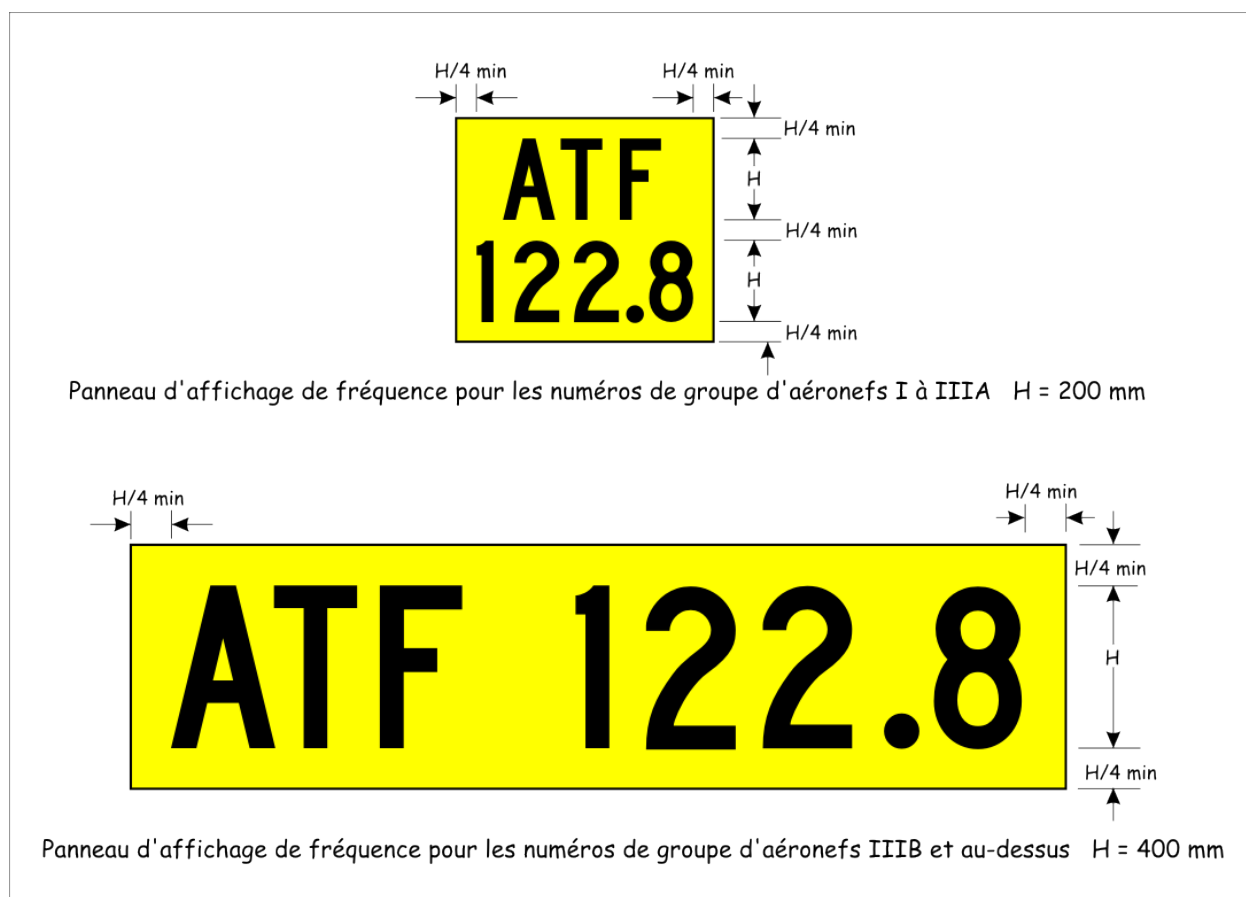
Figure 5-65 : Exemples de panneaux d'affichage de fréquence
