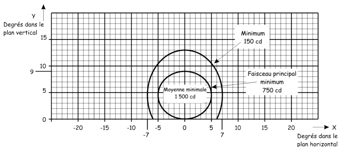
(a) Feux de décollage et de point d'attente (THL) et feux d'intersection de pistes
