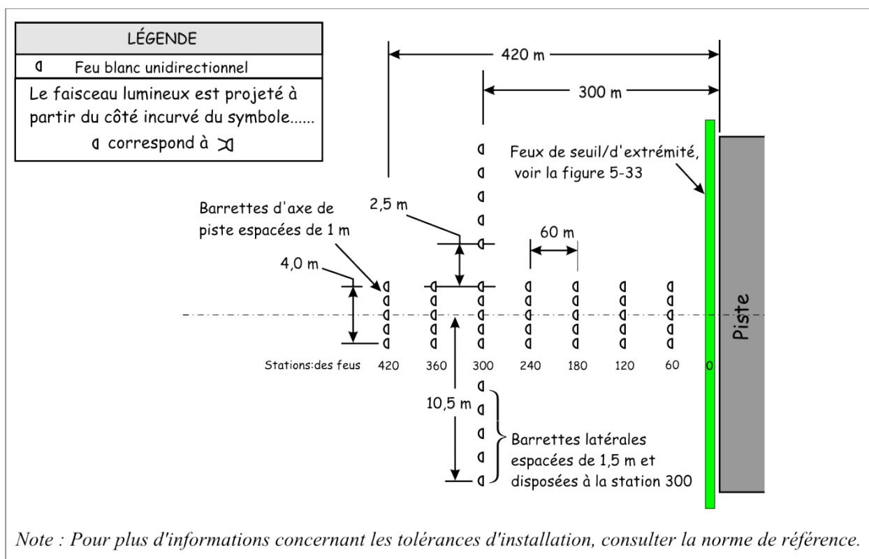
Figure 5-26 : Configuration des dispositifs MALSS/SSALS
