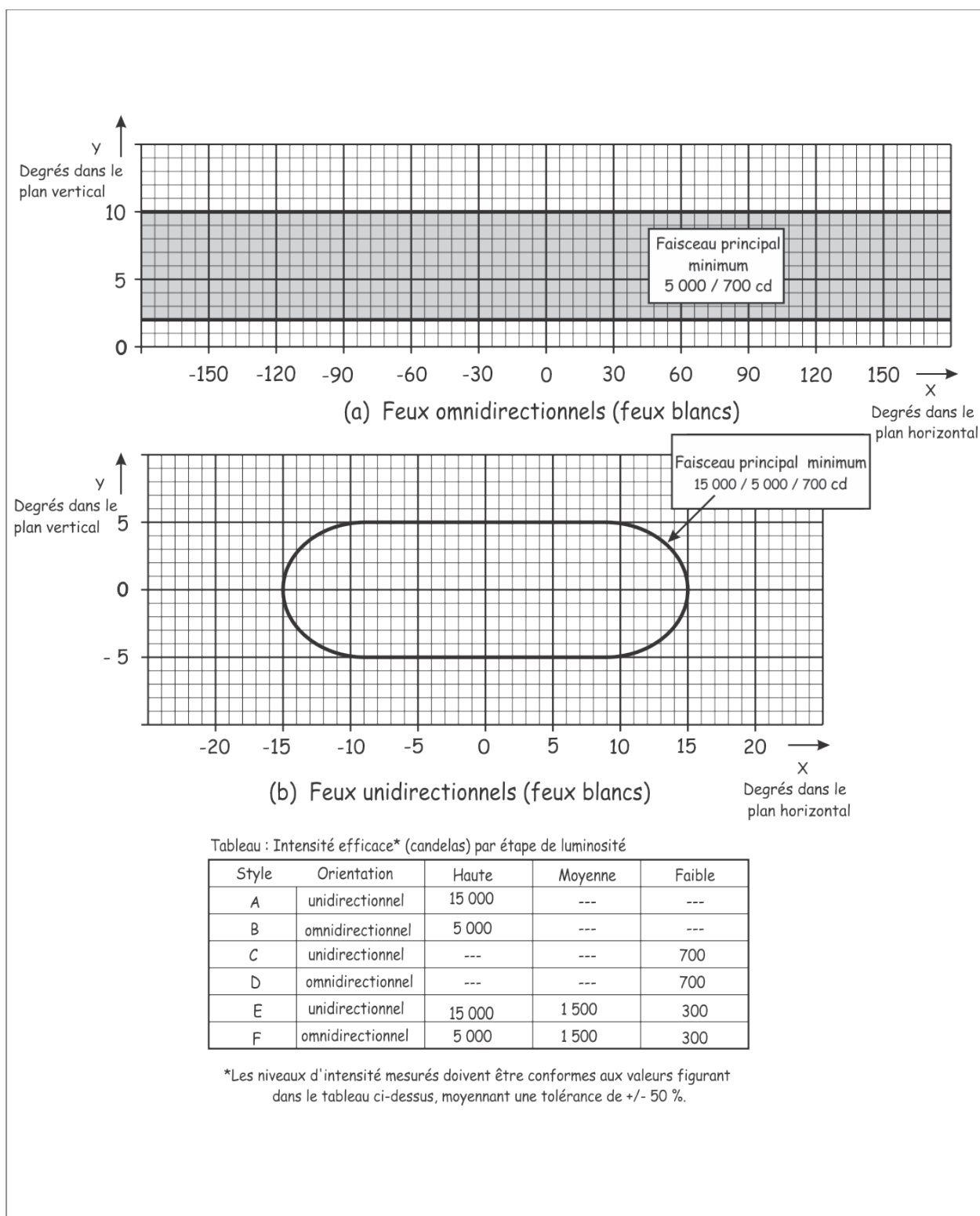
Figure B-23 : Diagramme isocandela des feux séquentiels des dispositifs (a) RTIL et ODALS (feux blancs) et (b) RTIL, LDIN, ALSF-2, SSALR, MALSR et MALSF (feux blancs)
