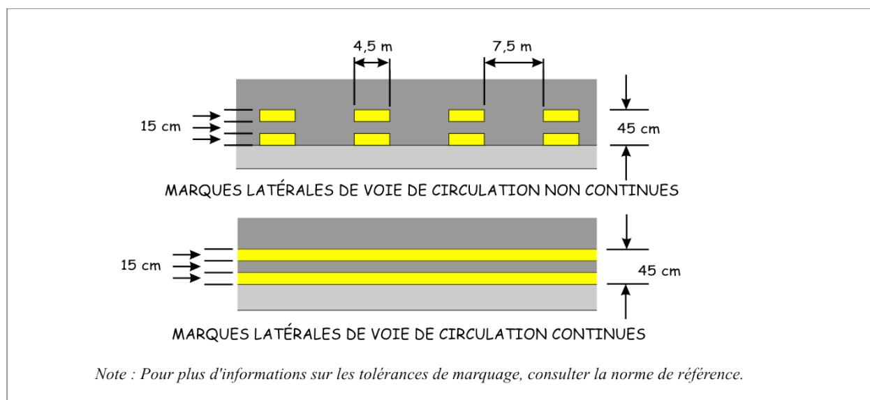
Figure 5-10 : Marques latérales de voie de circulation
