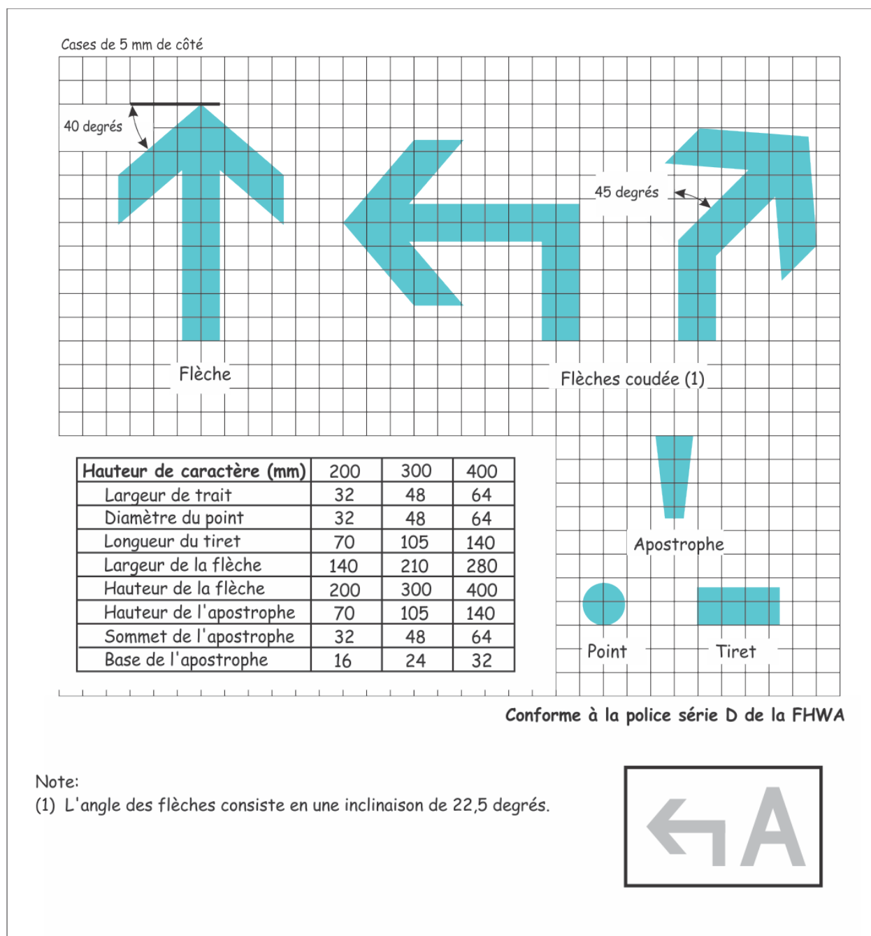
Figure 5-69 (d) : Proportions des caractères
