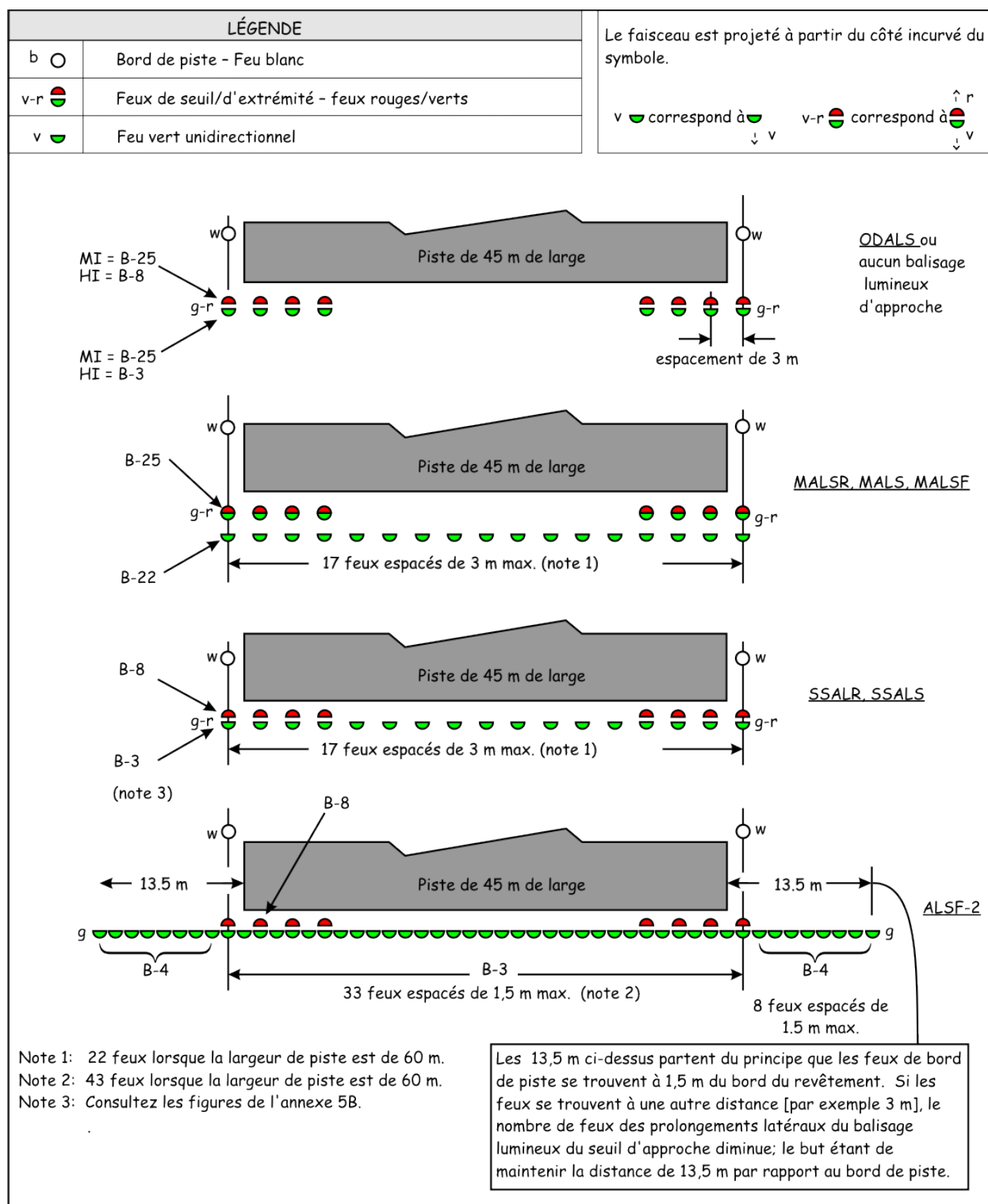
Figure 5-33 : Configuration des feux de seuil d'approche, de seuil de piste et d'extrémité de piste
