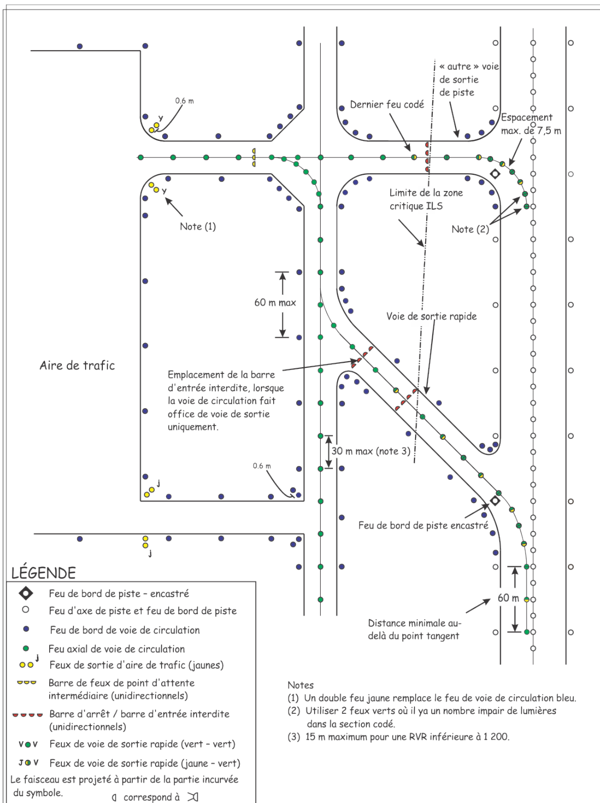
Figure 5-49 : Feux de voie de circulation
