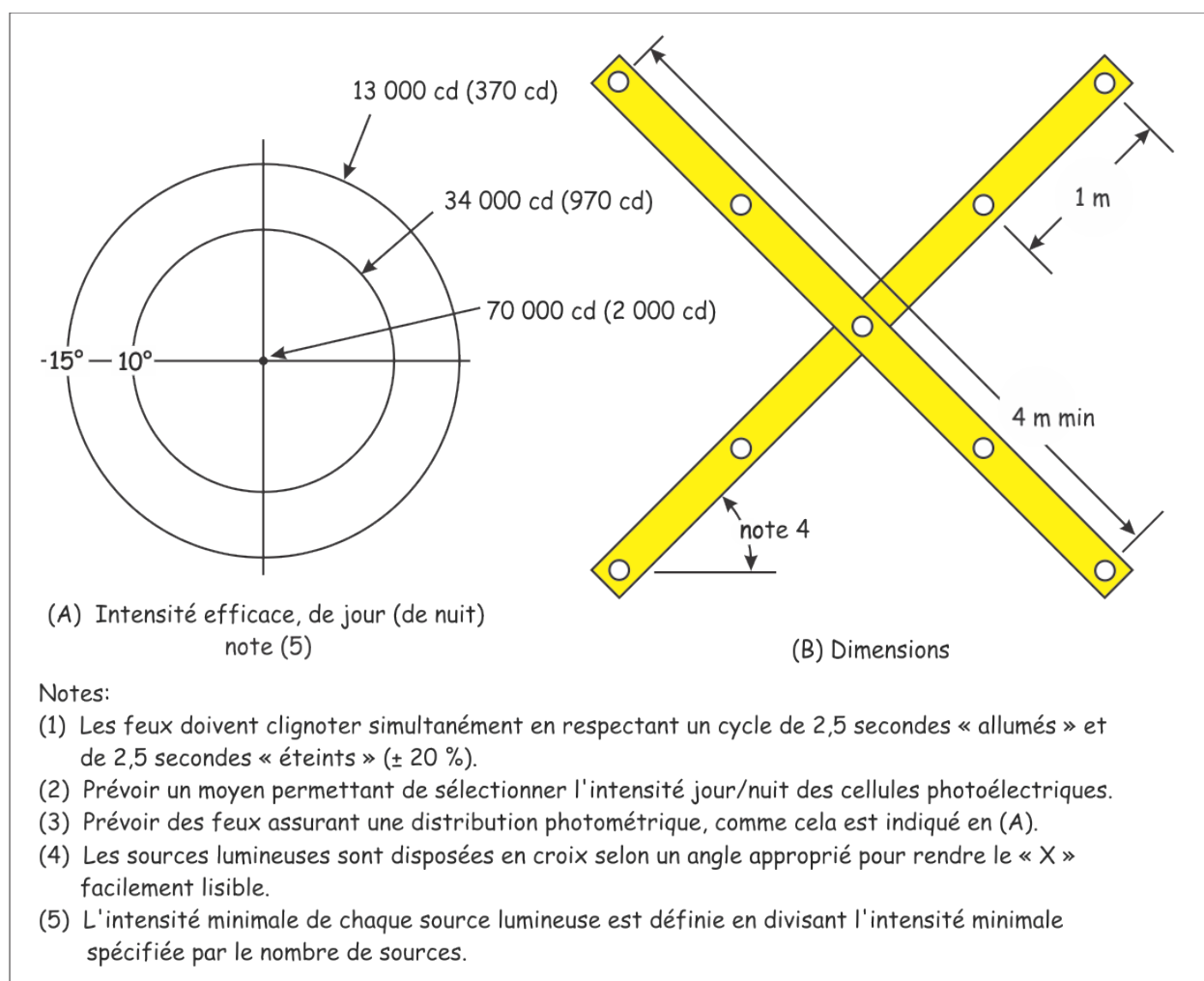
Figure 5-58 : Balise « X » éclairée de zone fermée
