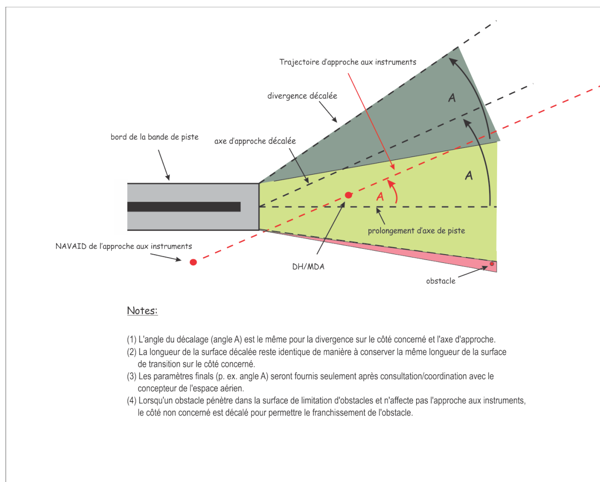
Figure 4-3 (a) : Surface d'approche décalée (piste de précision ou non-précision)
