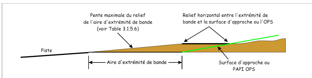
Figure 4-6 : Relief au-delà de l'extrémité de bande et dépassant la surface d'approche ou l'OPS
