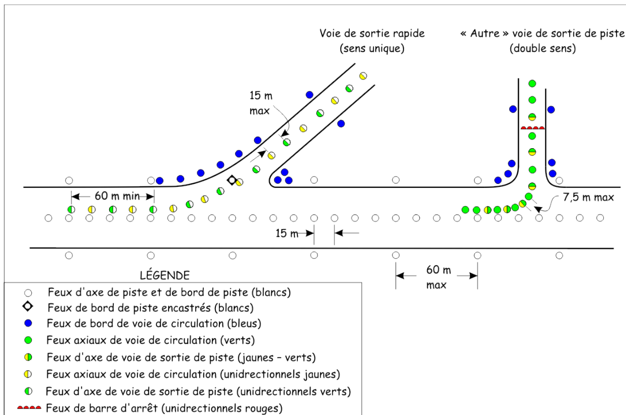
Figure 5-51 : Feux d'axe de voie de circulation
