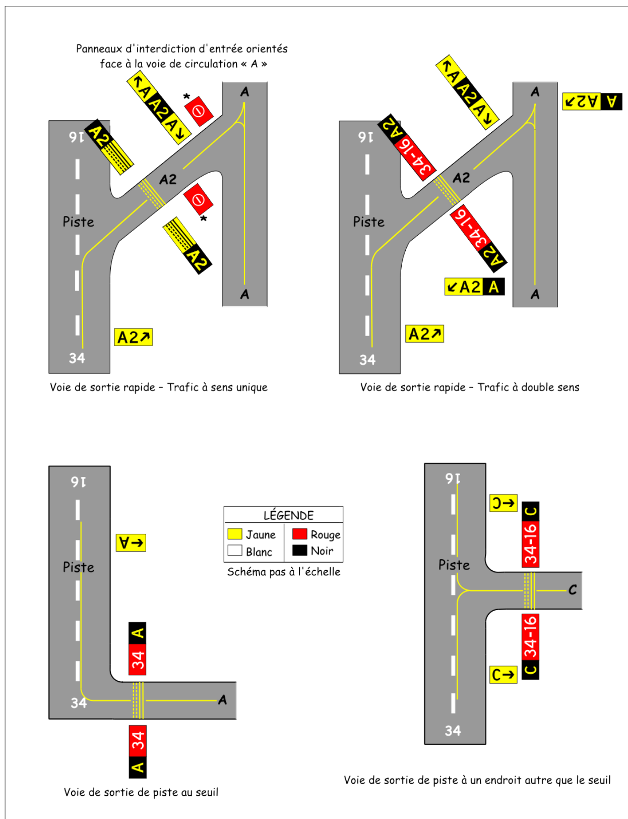
Figure 5-63 : Exemples d'emplacements des panneaux de sortie de piste et de dégagement de piste
