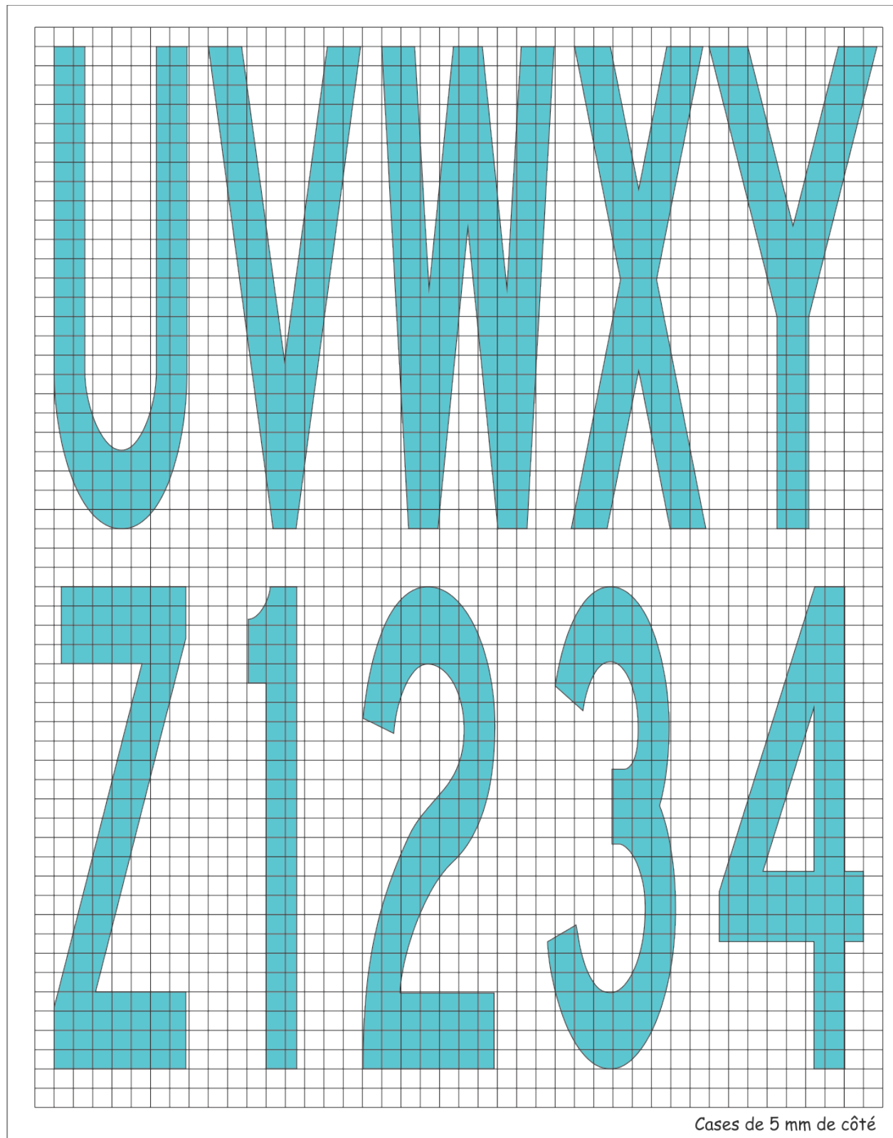
Figure 5-19 (c) : Marques de panneau peint sur la chaussée – Proportions des caractères
