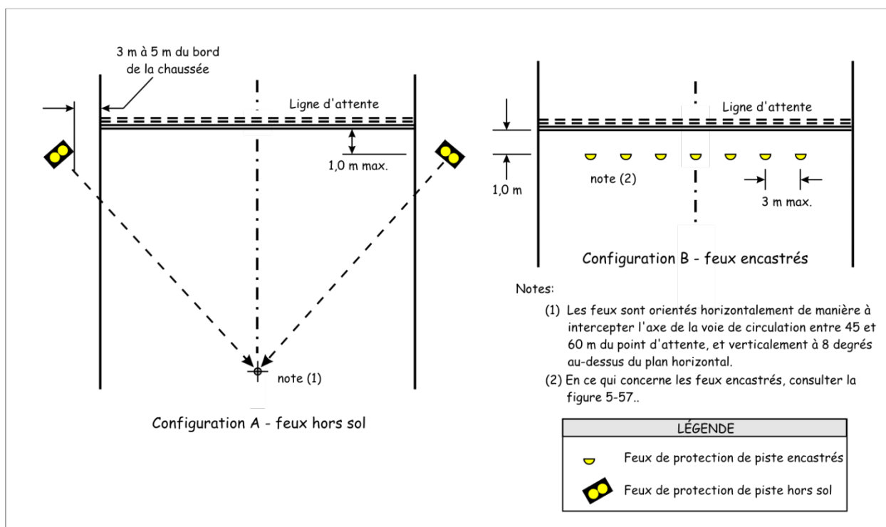
Figure 5-56 : Configuration A et B des feux de protection de piste
