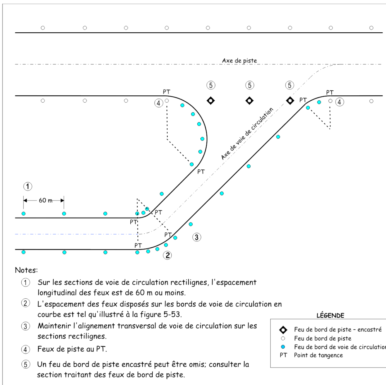
Figure 5-54 : Configuration des feux de bord de voie de circulation
