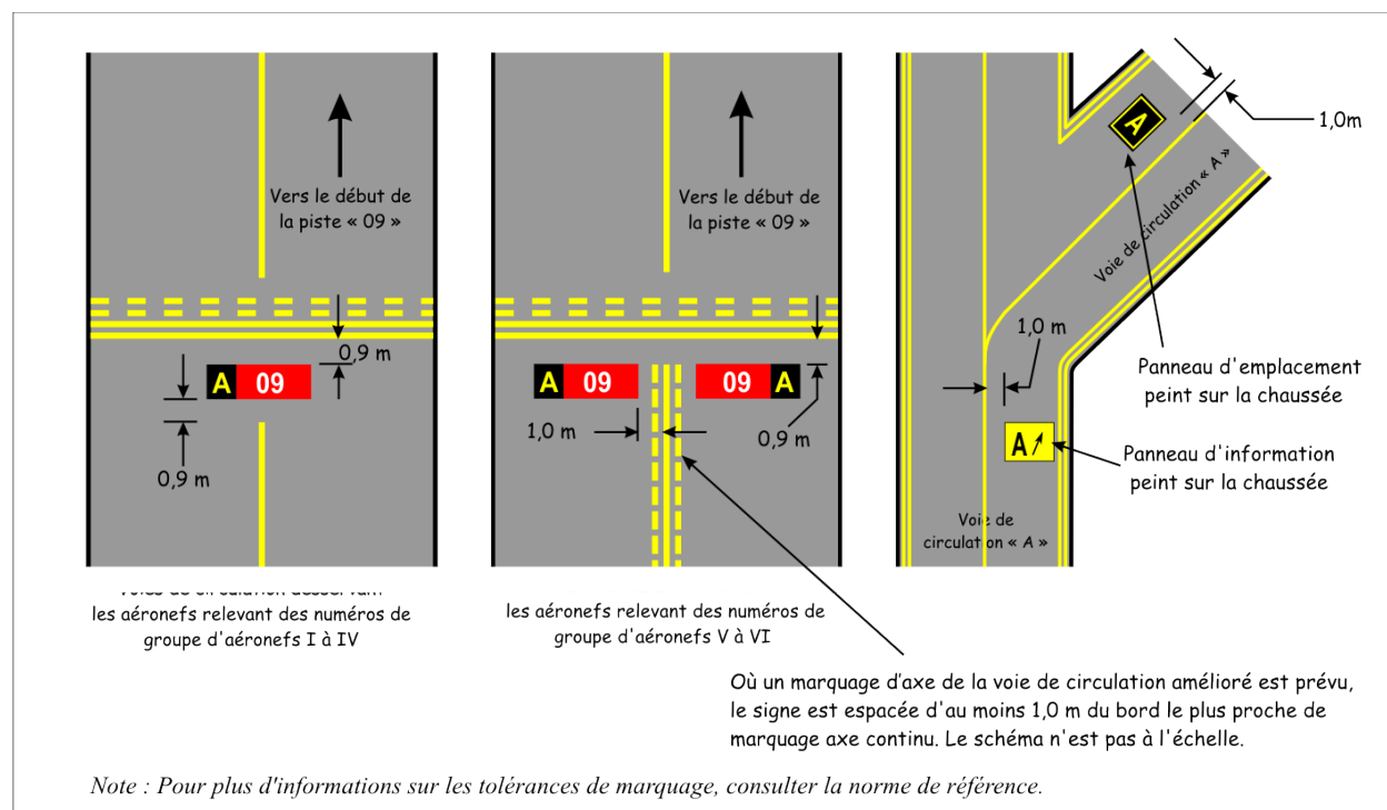
Figure 5-18 : Marques de panneau peint sur la chaussée
