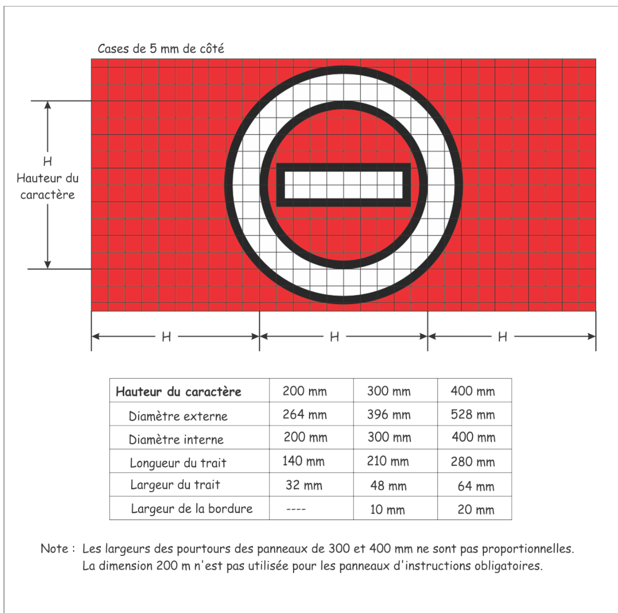
Figure 5-69 (f) : Proportions des caractères – Panneau d'interdiction d'entrée
