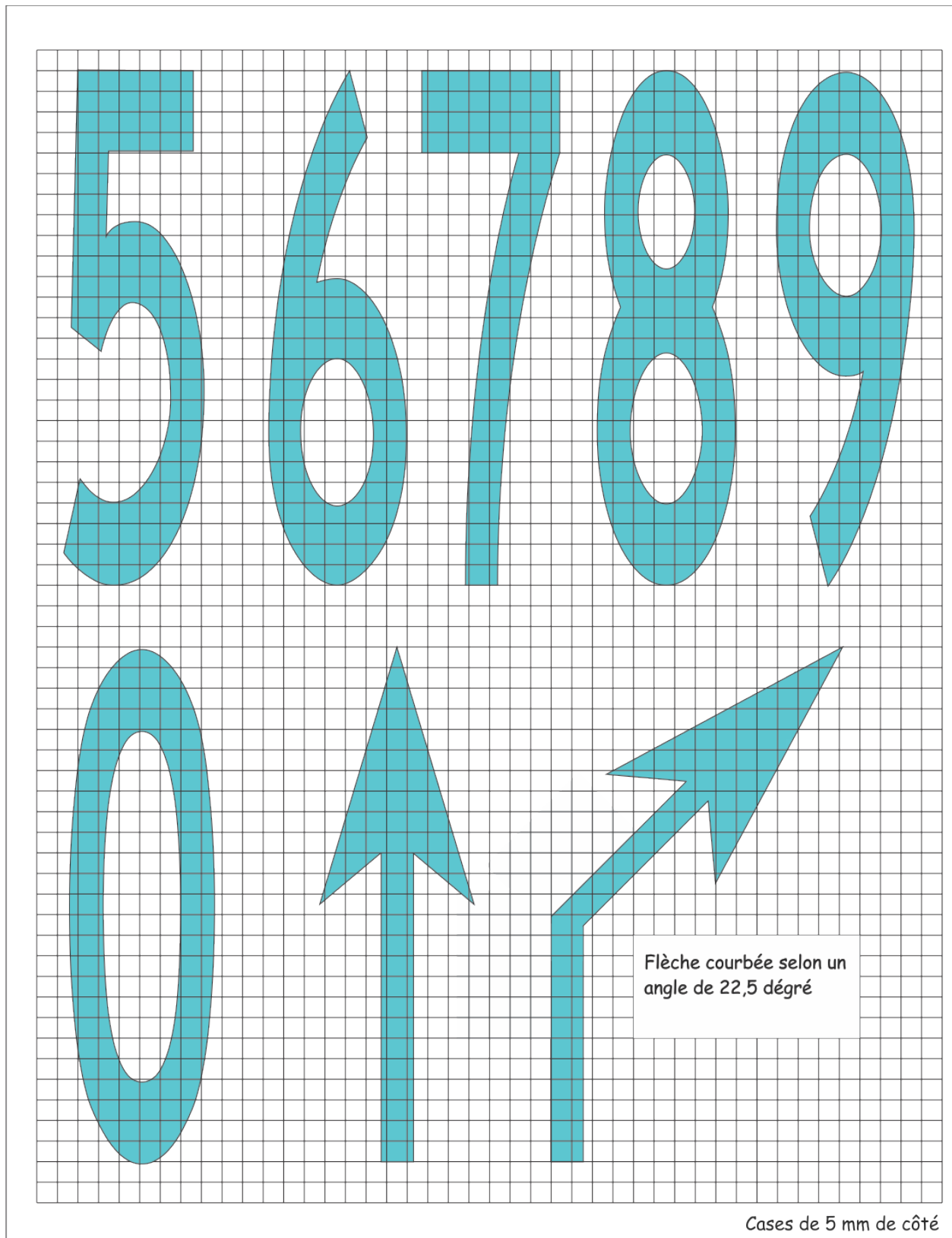
Figure 5-19 (d) : Marques de panneau peint sur la chaussée – Proportions des caractères
