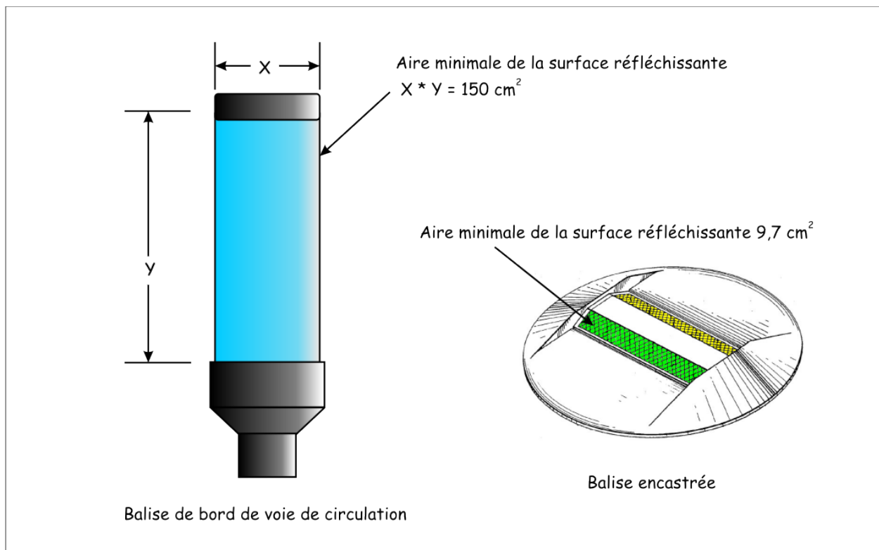
Figure 5-72 : Exemples de balises de bord et d'axe de voie de circulation
