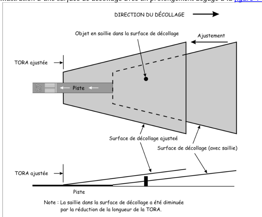
Figure 4-4 : Mesures de substitution concernant la pénétration dans la surface de décollage
